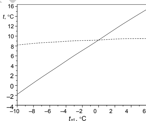
Рис. 2. Изменение температуры нагретого воздуха и подогрева приточного воздуха в конденсаторе: — — температура нагретого воздуха t_{n2} ; - - - — подогрев приточного воздуха в конденсаторе (t_{n2} - t_{n1})
