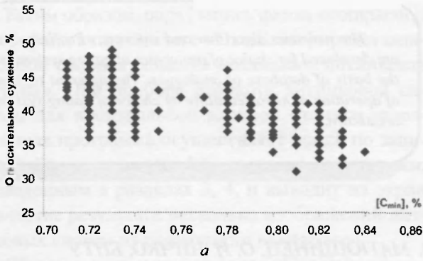
Рис. 13. Корреляционное поле минимального относительного сужения катанки и содержания углерода в катанке для проволоки диаметром 1,6 мм: a – минимальное значение содержания углерода; б – максимальное значение содержания углерода
