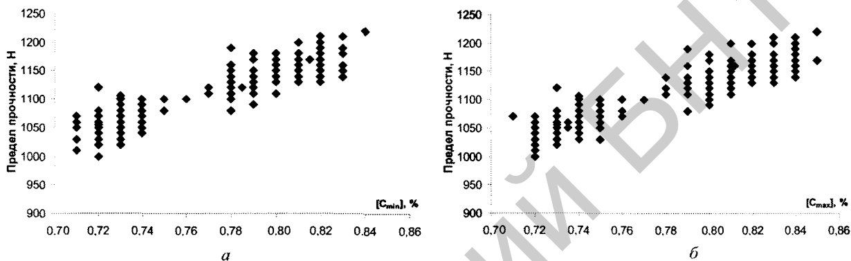
Рис. 13. Корреляционное поле максимального предела прочности катанки и содержания углерода в катанке для проволоки диаметром 1,6 мм: a – минимальное значение содержания углерода; б – максимальное значение содержания углерода
