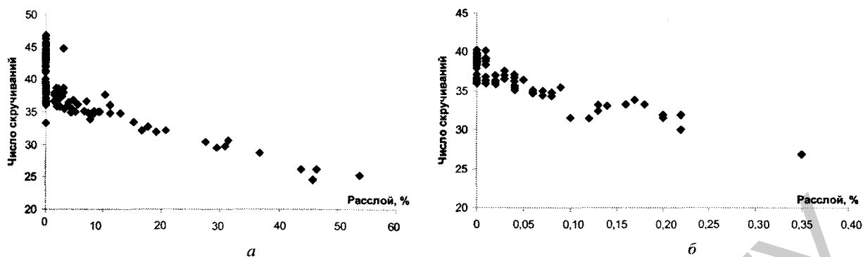
Рис. 2. Корреляционное поле числа скручиваний и величины раслоса для различных диаметров проволоки: а – диаметр 1,6 мм; б – диаметр 1,55 мм
