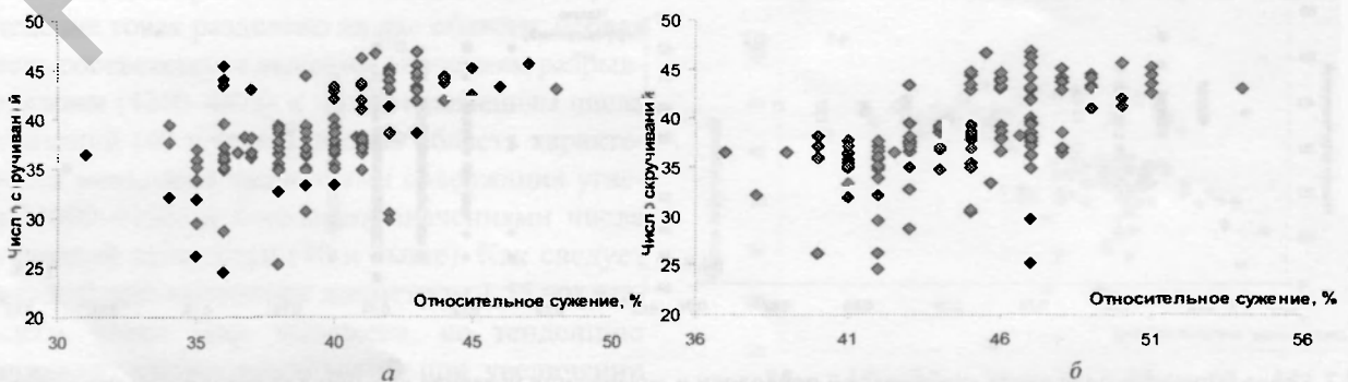
Рис. 9. Корреляционное поле числа скручиваний проволоки и относительного сужения катанки для проволоки диаметром 1,6 мм: а – минимальное значение относительного сужения; б – максимальное значение относительного сужения
