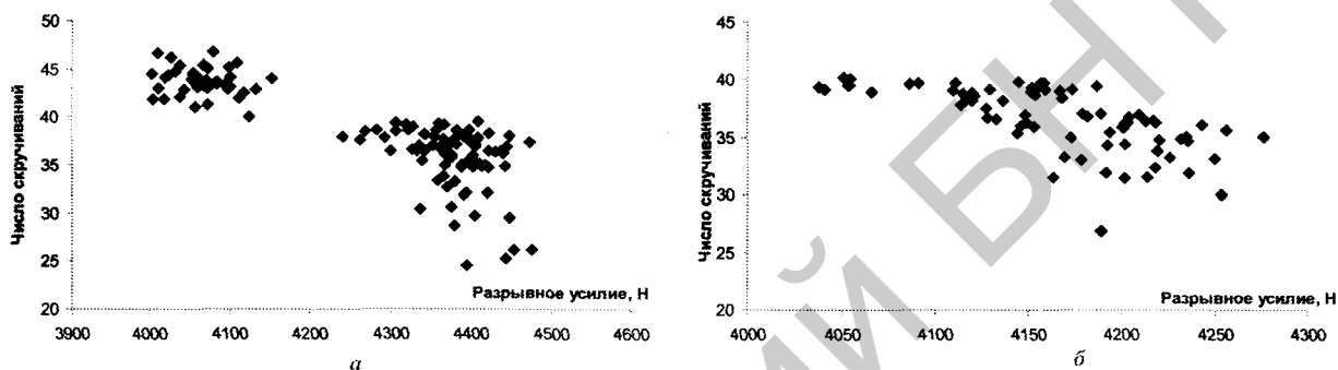
Рис. 3. Корреляционное поле числа скручиваний и разрывного усилия для различных диаметров проволоки: а – диаметр 1,6 мм; б – диаметр 1,55 мм
