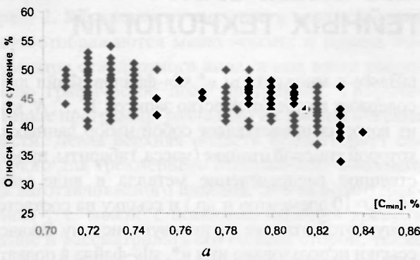
Рис. 14. Корреляционное поле максимального относительного сужения катанки и содержания углерода в катанке для проволоки диаметром 1,6 мм: a – минимальное значение содержания углерода; б – максимальное значение содержания углерода
