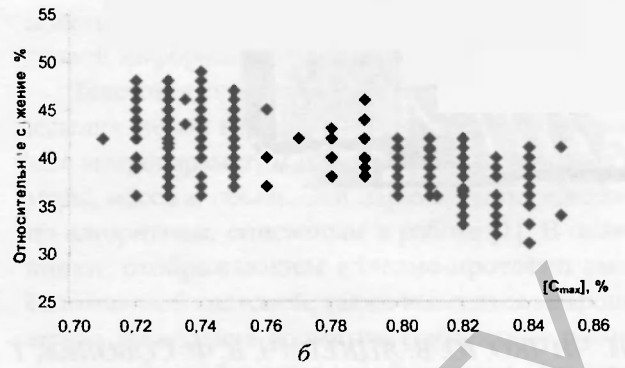
Рис. 13. Корреляционное поле минимального относительного сужения катанки и содержания углерода в катанке для проволоки диаметром 1,6 мм: a – минимальное значение содержания углерода; б – максимальное значение содержания углерода
