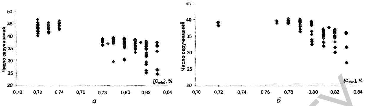
Рис. 5. Корреляционное поле числа скручиваний и минимального содержания углерода катанки для различных диаметров проволоки: a – диаметр 1,6 мм; б – диаметр 1,55 мм
