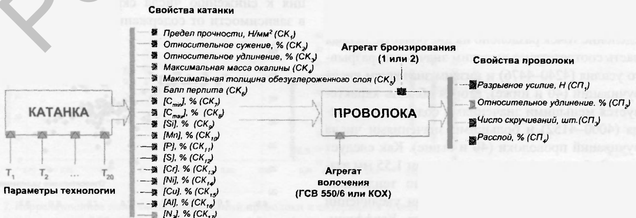
Рис. 1. Схема формирования свойств стальной бронзированной проволоки
