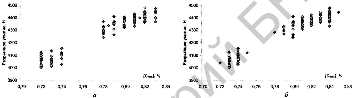
Рис. 10. Корреляционное поле разрывного усилия проволоки и содержания углерода катанки для проволоки диаметром 1,6 мм: а – минимальное значение содержания углерода; б – максимальное значение содержания углерода
