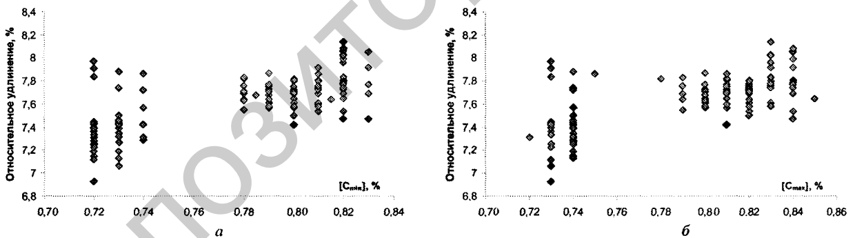
Рис. 11. Корреляционное поле относительного удлинения проволоки и содержания углерода в катанке для проволоки диаметром 1,6 мм: а – минимальное значение содержания углерода; б – максимальное значение содержания углерода
