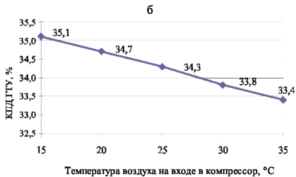
Рис. 1. ГТУ номинальной электрической мощностью 67,7 МВт SGT-1000F Siemens: зависимость мощности (а) и КПД (б) от температуры потока воздуха, поступающего в компрессор [1]
