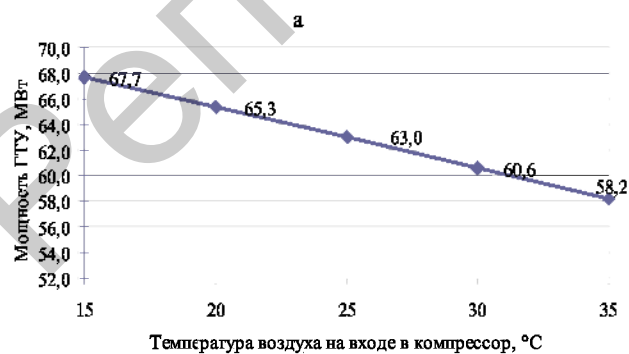
Рис. 1. ГТУ номинальной электрической мощностью 67,7 МВт SGT-1000F Siemens: зависимость мощности (а) и КПД (б) от температуры потока воздуха, поступающего в компрессор [1]
