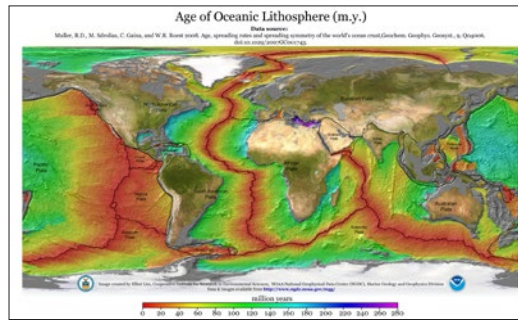
Fig. 5. Mapa geodinámico global de la Tierra, mostrando las placas tectónicas y la edad de la litosfera oceánica.
