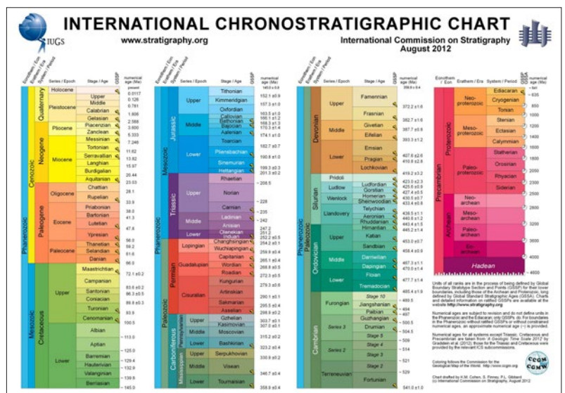
Fig. 7. Carta Cronoestratigráfica Internacional, elaborada por la Comisión Internacional de Estratigrafía de la IUGS.
