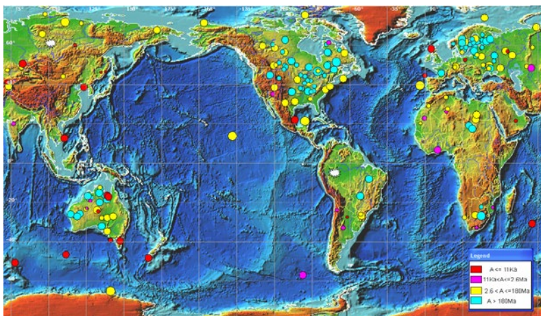
Fig. 9. Mapa de las estructuras de impacto confirmadas en la superficie terrestre (180 estructuras) y en el fondo oceánico (24 estructuras). El tamaño del círculo es proporcional al diámetro del cráter. El color muestra la edad de formación dividida en 4 grupos. Las estrellas blancas indican los epicentros de los dos eventos del siglo XX (Tinguska, 1908 y Brasil, 1930). Es importante tener en cuenta que 16 de las 24 estructuras conocidas en los fondos oceánicos se descubrieron entre 2005 y 2006. Créditos: Expert Database on the Earth Impact Structures (EDEIS), Tsunami Laboratory, ICMMG SD RAS, Novosibirsk, 2006.
