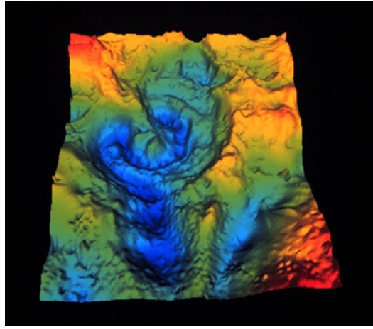
Fig. 8. Imagen generada por ordenador mostrando el mapa de gravedad del cráter de Chicxulub (Península del Yucatán). Fuente: NASA.
