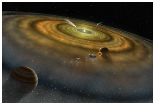
Fig. 1. Imagen artística representando la nebulosa solar primitiva y el proceso de formación planetaria por acreción de planetesimales. Fuente: NASA.
