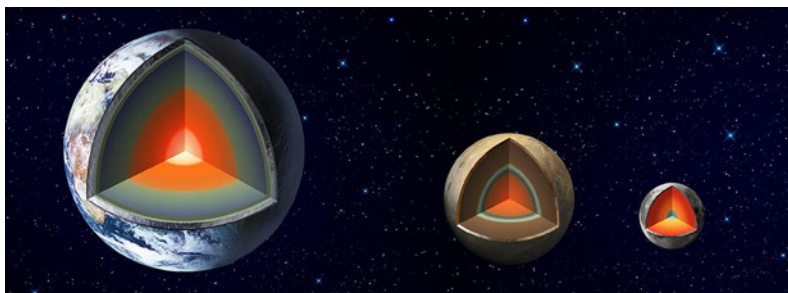
Fig. 4. Representación artística mostrando las estructuras comparadas de la Tierra, Marte y la Luna. NASA/JPL-Caltech.
