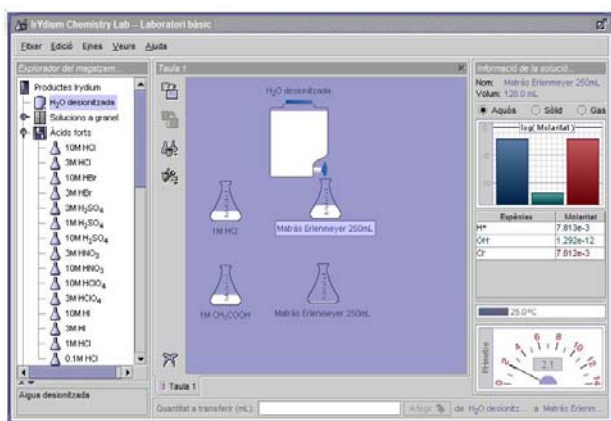
Figura 3. Materials i productes del laboratori virtual utilitzats en la investigació de la variació del pH en diluir un àcid fort i un àcid feble.
