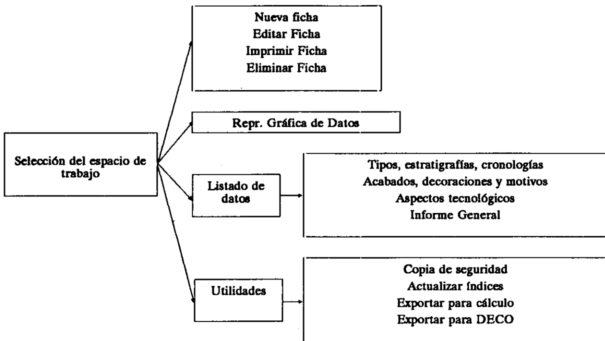
Fig. 2.—Organigrama del programa QW1.
