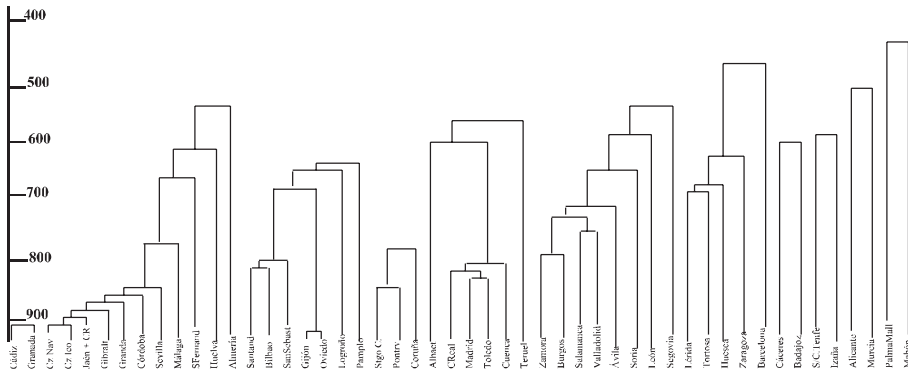
Gráfico 5: Agrupamiento de estaciones según el coeficiente de Pearson (x 1000)
