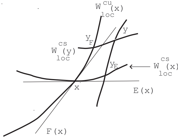
Figure 5 – Case y \notin W_{loc}^{cs}(x) , y \notin W_{loc}^{cu}(x) .
