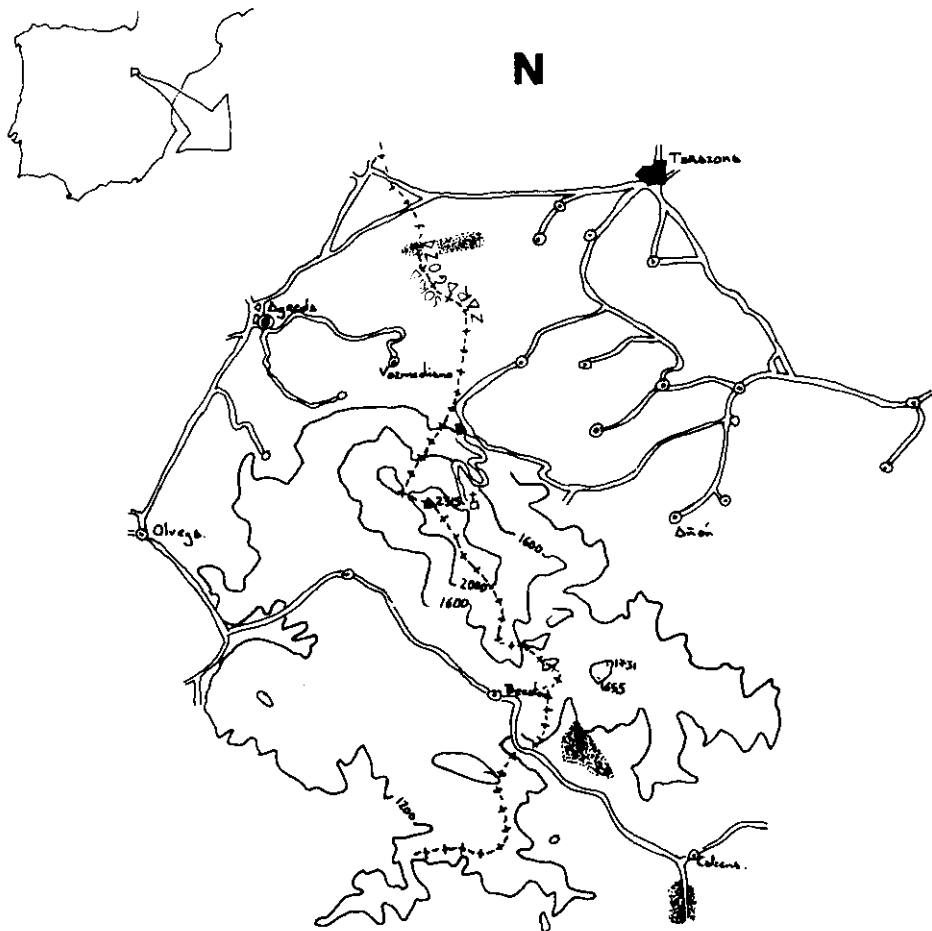
FIG. 1.—Localización de los principales relictos térmicos en el macizo del Moncayo (zonas punteadas).
