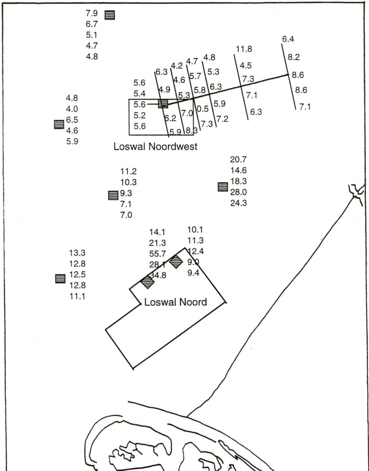
Fig. 3: Slibgehalten (totale fraktie <16 μm, %) van het sediment op en rond Loswal Noord en Loswal Noordwest.
