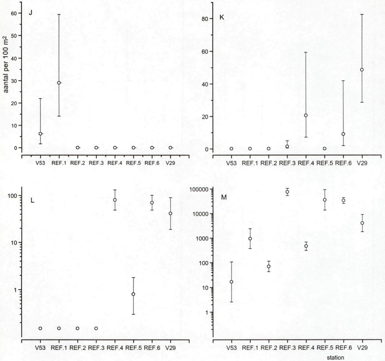
Fig. 10J-M: Gemiddelde dichtheden van schelpdieren (Mollusca) op Loswal Noord en de referentiestationen. De 95% betrouwbaarheidsgrenzen zijn aangegeven.
