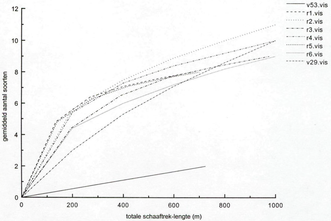
Fig. 7: Rarefaction curves voor makrobenthos (boven) en vissen (onder). Per station is het gemiddeld aantal soorten uitgezet dat is aangetroffen nadat een toenemend aantal schaaftrekken is uitgevoerd, resp. een toenemend aantal meters bodem met de schaaftrek is bemonsterd.
