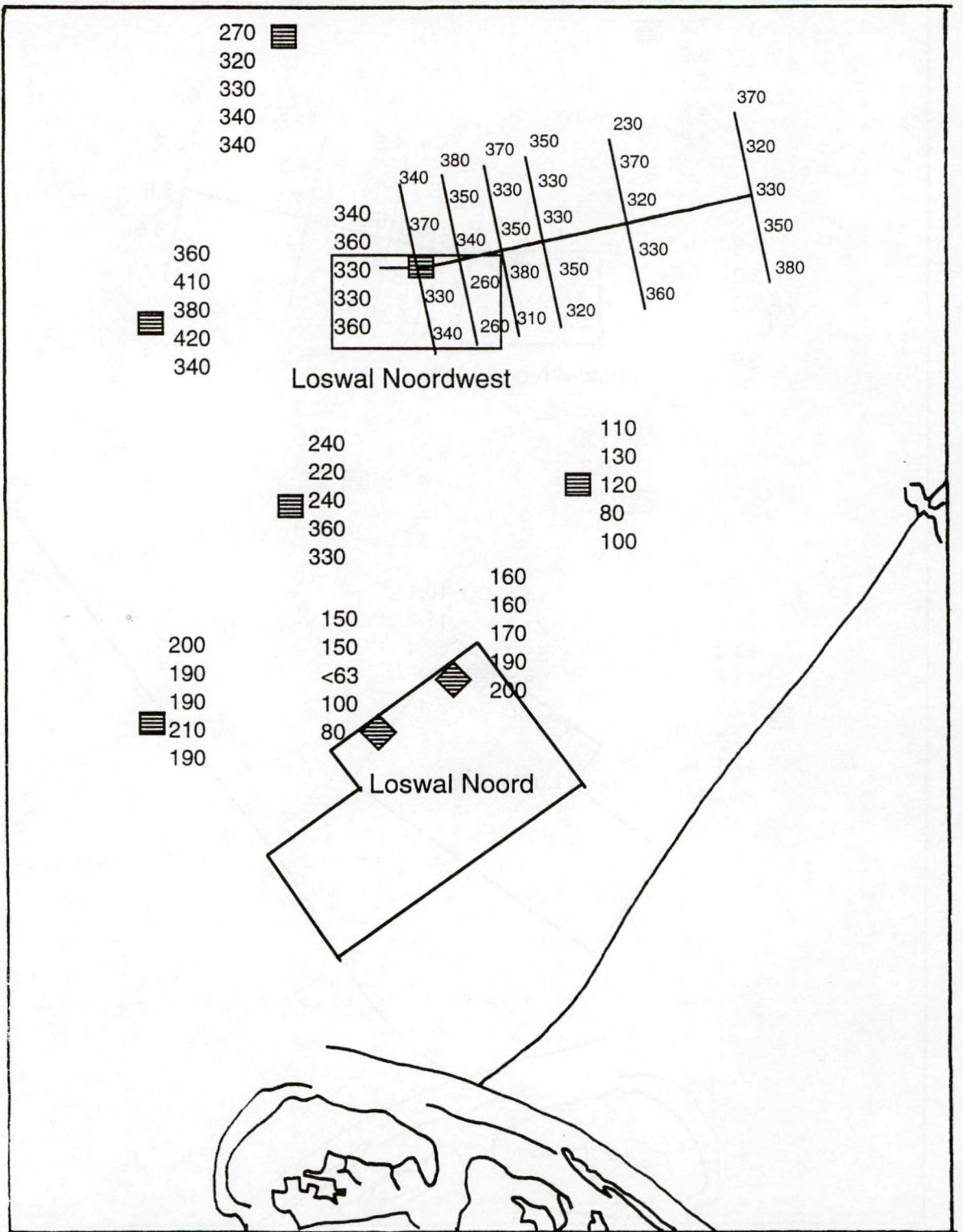
Fig. 4: Mediane korrelgrootte (µm) van het sediment (inclusief de slibfractie) op en rond Loswal Noord en Loswal Noordwest.
