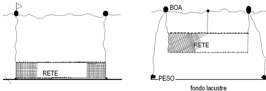
Figura 1 Rappresentazione schematica della metodologia di posa per le Reti Multimaglia Bentiche RMB (a sn) e Mesopelagiche RMP (a dx).
