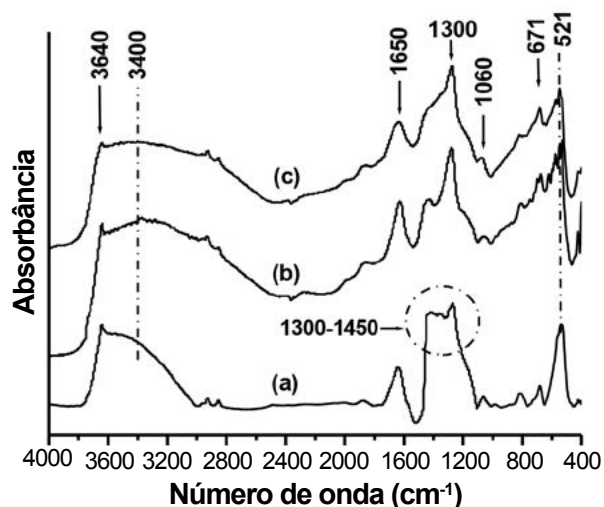
Figura 3: Espectros de DRIFT: (a) ES1; (b) ES2; (c) ES3.
