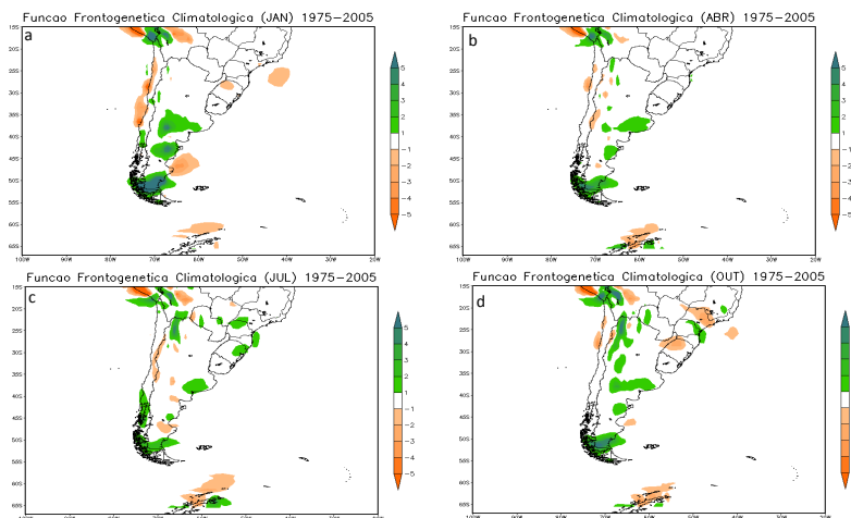
Figura 1: Média mensal para 30 anos da FF ( 10^{-10} \text{ K.m}^{-1}.\text{s}^{-1} ). a) JAN. b) ABR. c) JUL. e d) OUT.
