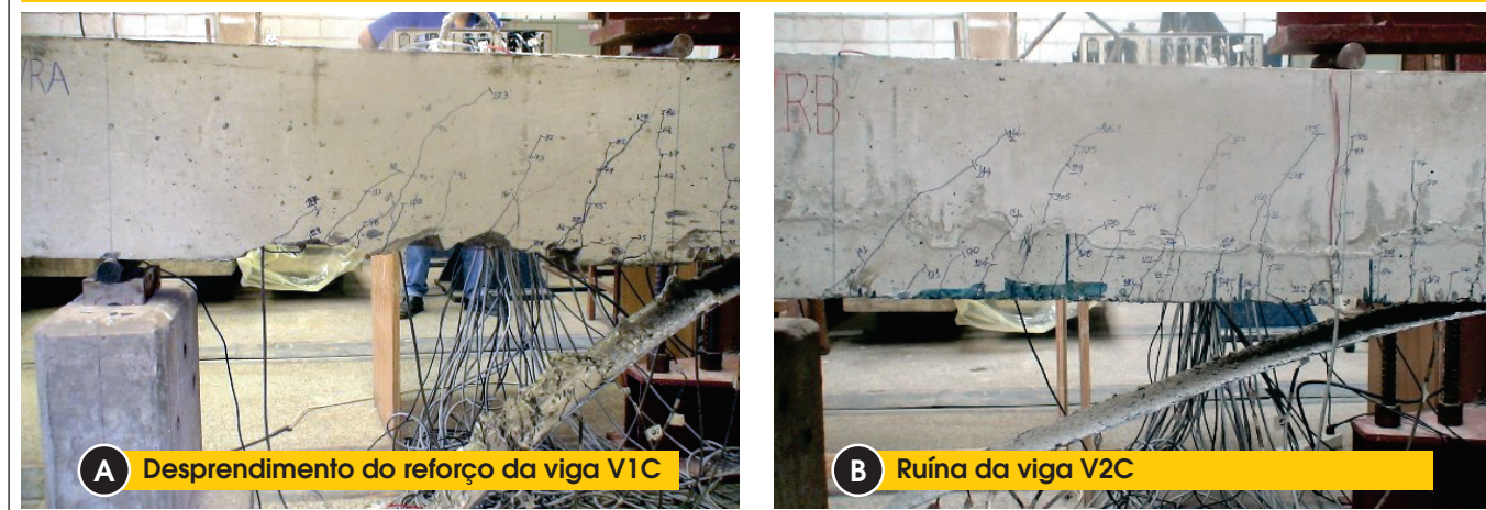
Figura 11 - Modo de ruína das vigas V1C e V2C
