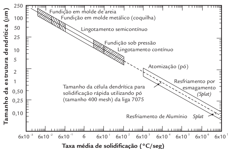
Figura 3 Relação entre o tamanho da estrutura dendrítica e a taxa de solidificação para ligas de alumínio (Spears & Gardner, 1963).
