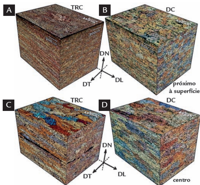
Figura 1 Microestruturas obtidas por MO, nas regiões central e próxima à superfície das chapas da liga AA4006 (no estado como recebido), obtidas por (A) e (C) lingotamento contínuo e (B) e (D) lingotamento semicontínuo.
