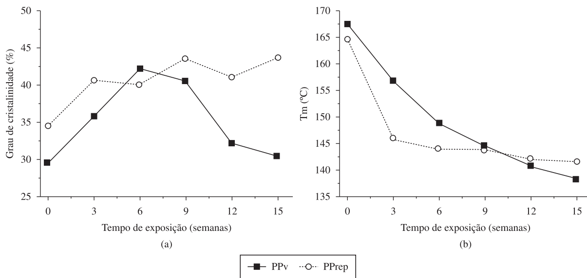
Figura 4. Efeito do tempo de exposição no: a) grau de cristalinidade e b) temperatura de fusão cristalina do PPv e do PPrep.
