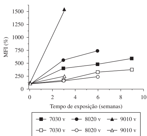
Figura 7. Efeito do tempo de exposição à radiação UV no MFI das blendas PP/HIPS. Os dados para as blendas PPrep/HIPS já foram apresentados [21] e são apresentados aqui apenas por fins comparativos.
