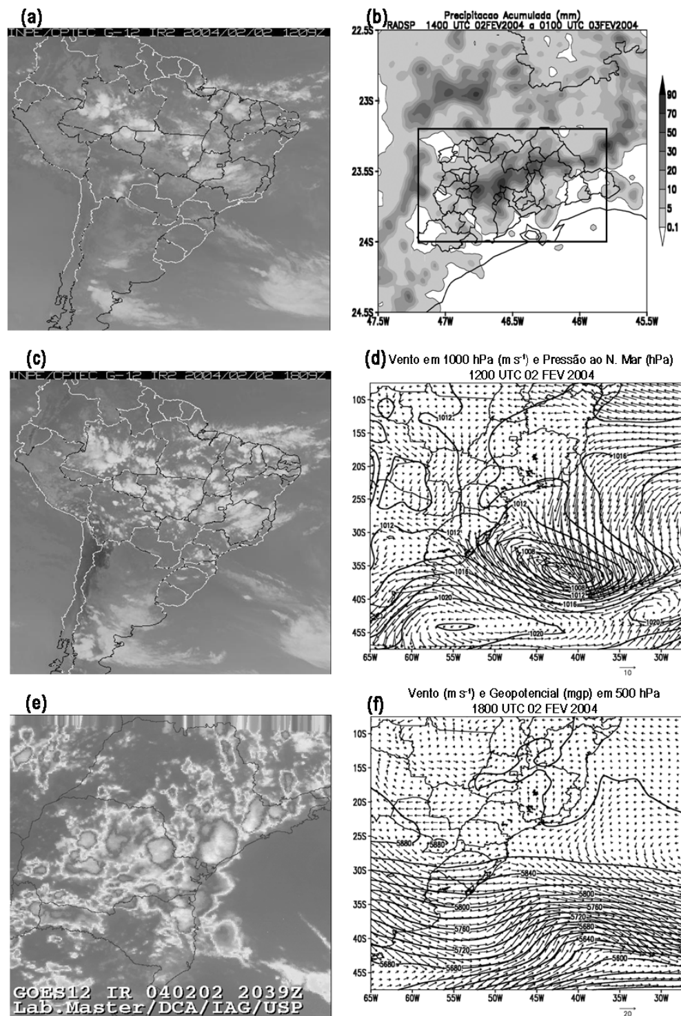
Figura 10 - (a) Imagem GOES-12 no canal infravermelho às 1209 UTC 02 FEB 2004. (b) Precipitação acumulada estimada com as medidas RADSP no período indicado no topo da figura. (c) Imagem GOES-12 no canal infravermelho às 1809 UTC 02 FEB 2004. (d) Análise GFS para os campos de vento em 1000 hPa e pressão reduzida ao nível do mar às 1200 UTC 02 FEB 2004. O vetor de referência corresponde a 10 m s^{-1} . O intervalo das isóbaras é de 2 hPa. (e) Imagem GOES-12 no canal infravermelho às 2039 UTC 02 FEB 2004; (f) Análise GFS para os campos de vento e altura geopotencial em 500 hPa às 1800 UTC 02 FEB 2004 O vetor de referência corresponde a 20 m s^{-1} . O intervalo das isolinhas é de 20 mgp.
