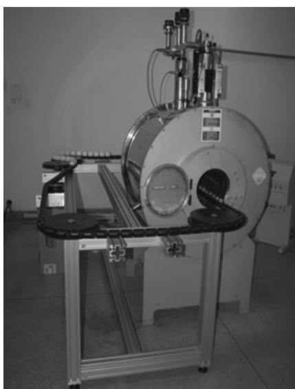
Figura 3. Esteira de poliacetal, usada para medidas online, formada por 105 gomos de 65 mm atravessando o bore de 30 cm de diâmetro do magneto de 2,1 T
