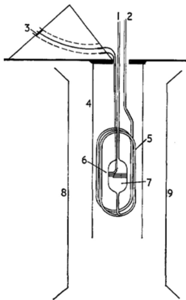
Figura 1. Configuração da sonda de RMN proposta por McIvor, incorporando a região de pré-magnetização: 1, entrada da amostra em fluxo; 2, saída da amostra em fluxo; 3, conexão da sonda de RF; 4, proteção metálica; 5, serpentina de polarização; 6, bobina de RF; 7, célula de compartimento da amostra; 8 e 9, partes do pólo do magneto. Reproduzida da ref. 13, com permissão da IOPscience Publishing Limited
