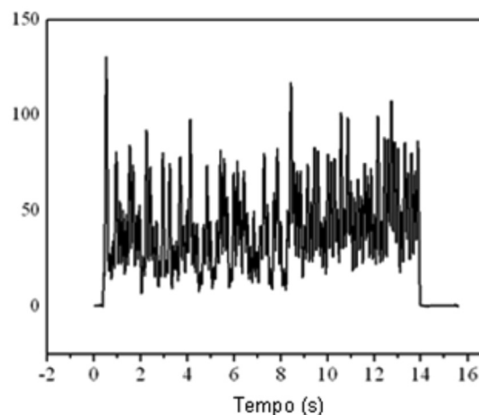
Figura 4. Sinal de RMN online, obtido pela técnica CWFP, de amostras de sementes oleaginosas. Adaptada da ref. 36, com permissão da American Chemical Society
