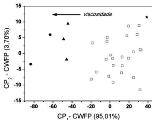
Figura 6. Gráfico dos escores obtidos com a análise por PCA dos dados obtidos por CWFP. Adaptada da ref. 39, com permissão da Wiley
