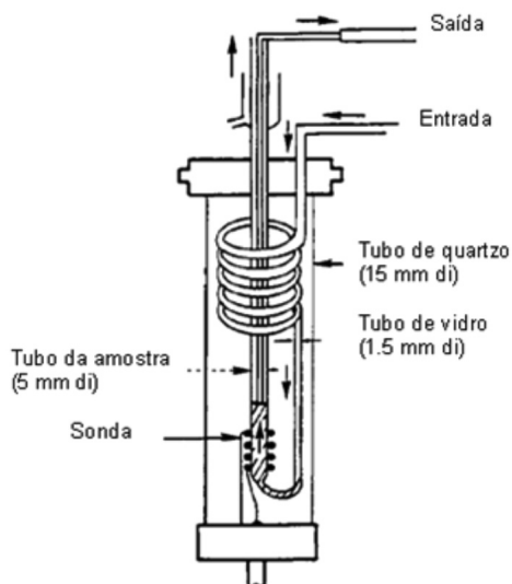
Figura 2. Sistema para acoplamento de RMN-TF em fluxo com o aparelho de HPLC, incorporando a região de pré-magnetização. A amostra entra por um tubo espiral de quartzo de 15 mm, que faz com que a amostra se mantenha por mais tempo no interior no magneto, possibilitando sua polarização antes de entrar na região de detecção da sonda. Adaptada da ref. 21, com permissão da American Chemical Society
