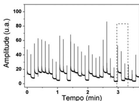
Figura 5. Sinal de 31 amostras de espécies oleaginosas obtidos com a sequência CWFP online utilizando o método stop and flow. Adaptada da ref. 39, com permissão da Wiley
