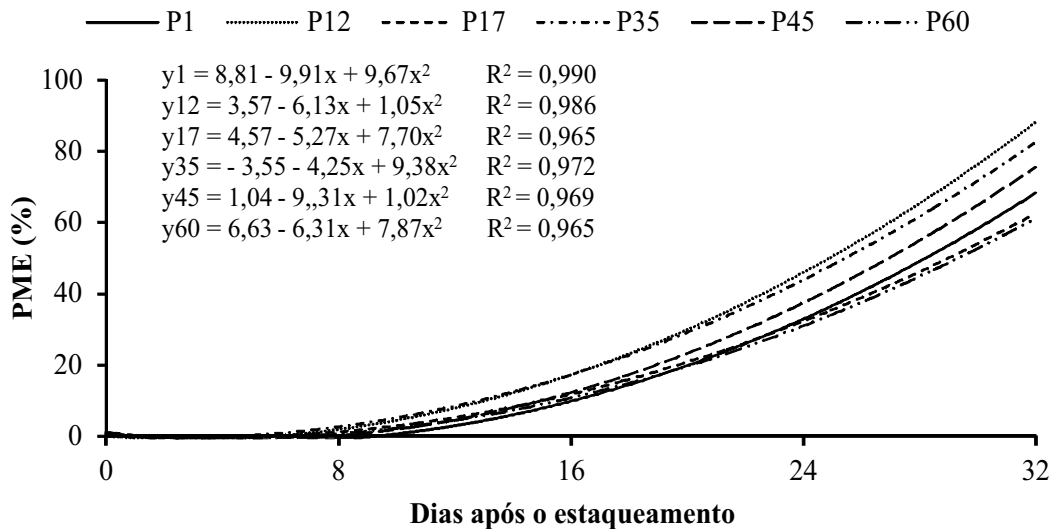
Figura 2 – Porcentagem de miniestacas enraizadas (PME), em seis progênies de meios-irmãos de Anadenanthera macrocarpa , em função do tempo após o estaqueamento.
