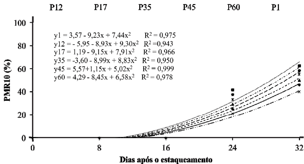
Figura 3 – Porcentagem de miniestacas com raízes maiores que 10 cm (PMM10), em seis progênies de meios-irmãos de Anadenanthera macrocarpa , em função do tempo após o estaqueamento.
