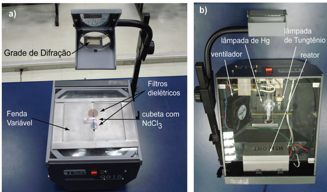
Figura 15. a) Fotografia mostrando o retroprojektor em uma configuração típica de observação dos espectros de transmissão. b) Figura do interior do retroprojektor, enfatizando as modificações realizadas
