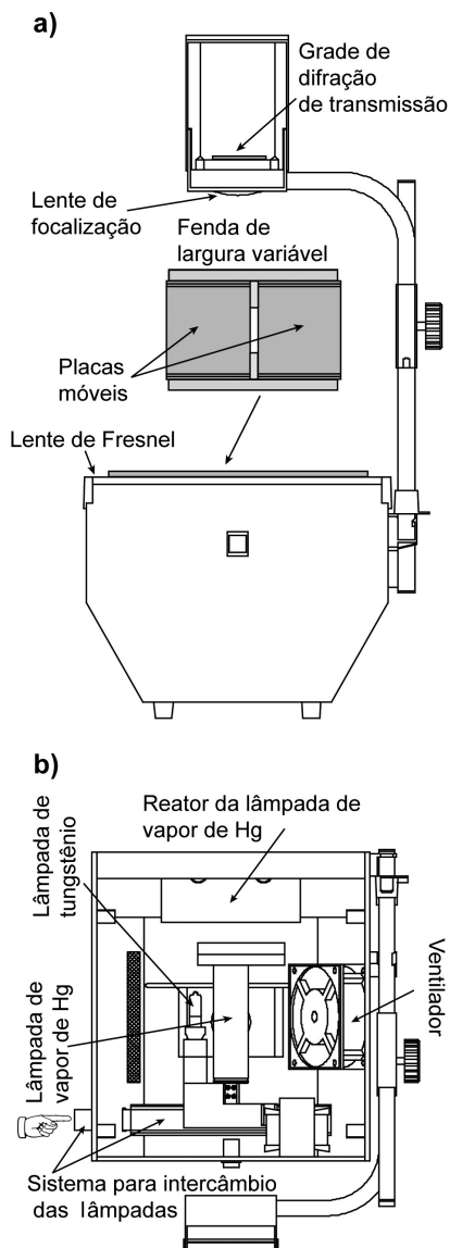
Figura 1. a) Desenho esquemático da vista lateral do retroprojetor com a fenda de largura variável evidenciada. b) Corte transversal (visto de cima) do interior do retroprojetor. (Ver fotografia do retroprojetor modificado na Figura 1S do material suplementar)
