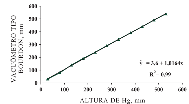
Figura 2. Calibração do vacuômetro de Bourdon e a equação de ajuste (Brito, 2007).
