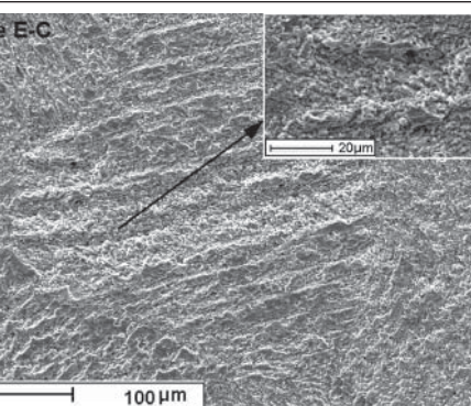
Figura 4 - Sequência de micrografias apresentando a evolução e os mecanismos de dano por E-C em um aço UNS S30803 nitretado em alta temperatura.
