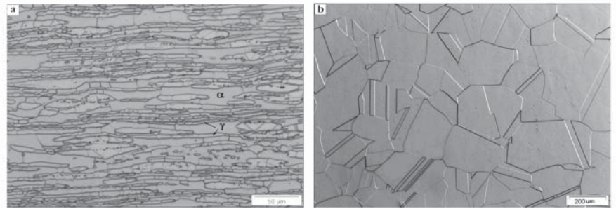
Figura 2 - Micrografias do aço UNS 30803 a) como recebido e b) após nitretação e recozimento.
