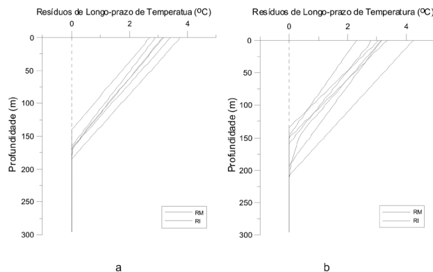
Figura 7 - Resíduos térmicos de longo-prazo de temperatura do subsolo do tipo (a) LCCV e (b) LSCV. RM é o valor residual médio e RI são os valores residuais individuais de \mathcal{R}_{i-f} para cada perfil.
