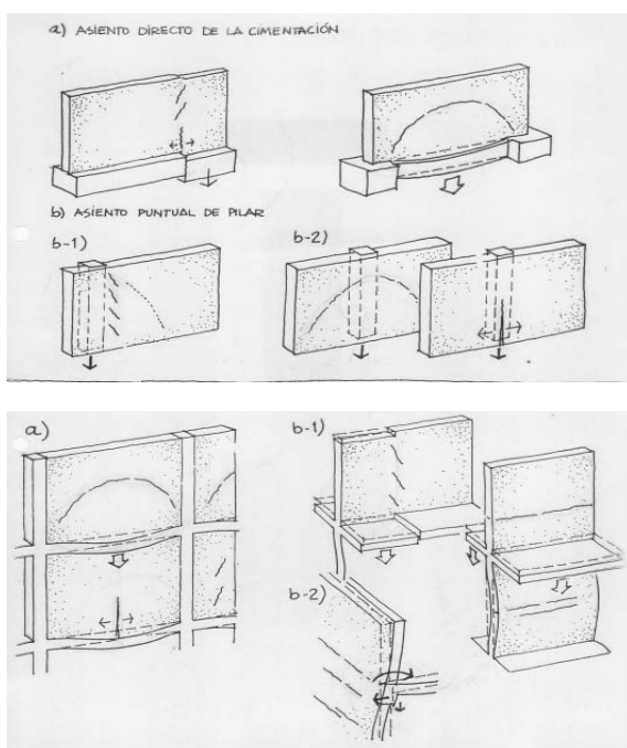
Figura 5.- Interacción entre estructura y fachada no portante (dibujos del autor).
