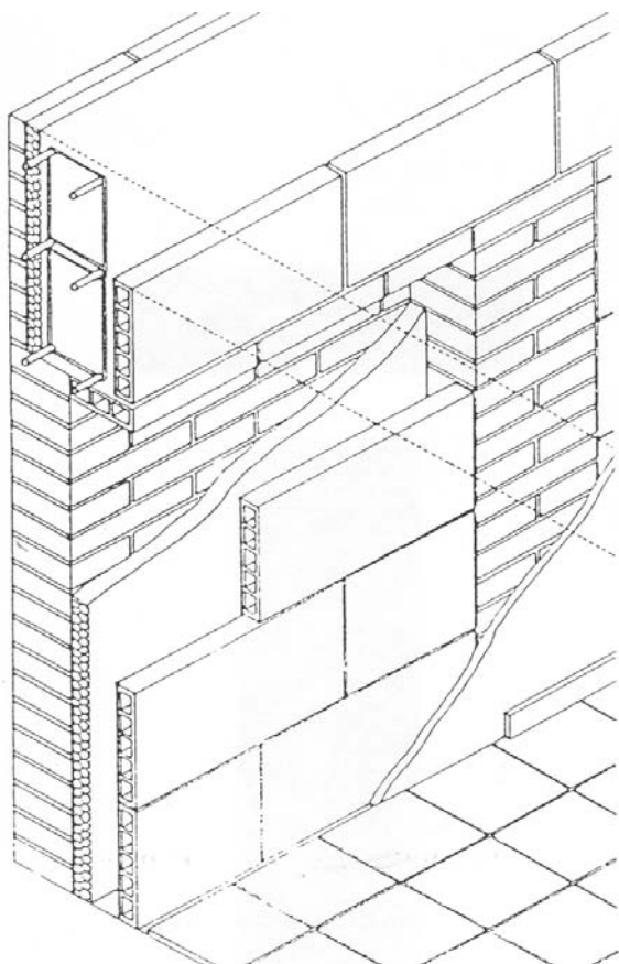
Figura 10.- Esquema de encuentro teórico de fachada y estructura.
