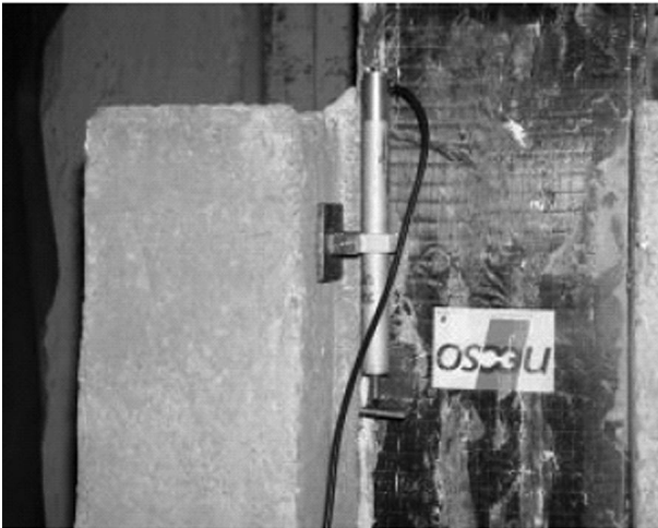
Figura 6. Detalle del sensor utilizado en los ensayos de "push-out".
