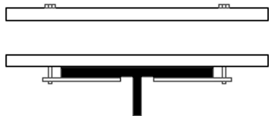
Figura 2. Conexión empotrada formada por dos tornillos que unen el tablero a las placas que se fijan a las vigas metálicas del puente, en este caso de sección en doble te.
