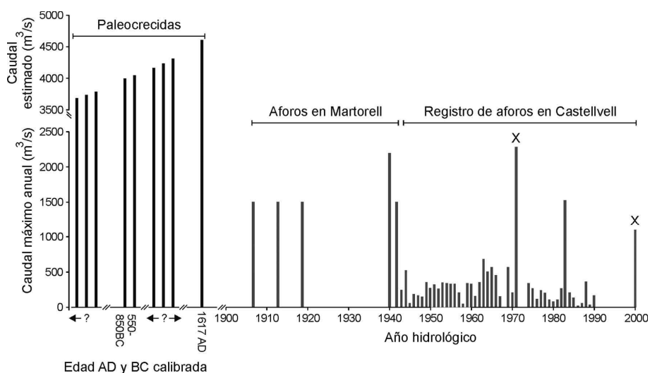
Figura 3. Caudales estimados de crecidas máximas producidas en los últimos 3000 años en el tramo medio-inferior de río Llobregat mediante registros geológicos, junto con los registrados en las estaciones de aforo de Martorell y Castellvell (Thorndycraft et al., 2004).
