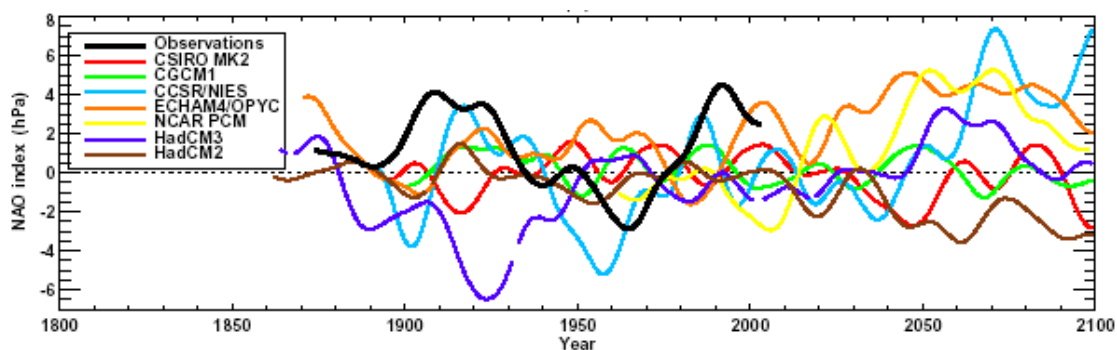
Figura 7. Series temporales del índice NAO (hPa) de la diferencia de la presión baja oceánica entre Gibraltar e Islandia obtenida a partir de datos observados (negro) y de datos simulados bajo un incremento en la concentración de los gases de invernadero. Todas las series se han suavizado mediante un filtro de 30 años. La falta de datos en la serie del HadCM3 se debe a la pérdida de algunos años en los datos de registro (según Osborn, 2004).
