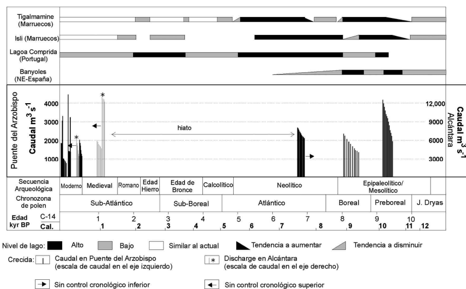
Figura 2. Distribución temporal de las paleocrecidas y estimación de caudales en el río Tago durante el Holoceno (según Benito et al., 2003a). Cada barra representa un evento de crecida. En la parte superior, se muestran los cambios en el nivel de agua en algunos lagos seleccionados del entorno de la Península Ibérica. Nivel en los lagos: Lago Tigalmamine (Marruecos) según Lamb et al., (1989); Lago Isli (Marruecos) según Zeroual (1995); Lagoa Comprida (Portugal) según Van der Brink, L.M., Janssen, C.R., (1985); y Banyoles (NE-España) según Pérez-Obiol and Juliá (1994), Roca y Juliá, (1997); Juliá et al., (1998); y Valero-Garcés et al., (1998).
