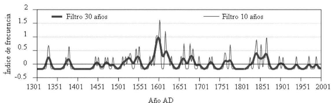
Figura 5. Evolución de la frecuencia de crecidas extraordinarias y catastróficas de los ríos Segre, Llobregat y Ter (según Llasat et al., 2005). Los datos aparecen representados después de aplicar un filtro de suavizado de 10 y 30 años.
