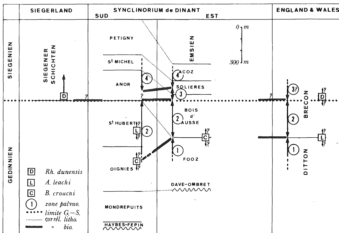
Figure 7.- Corrélations biostratigraphiques (spores et ostracodermes)
