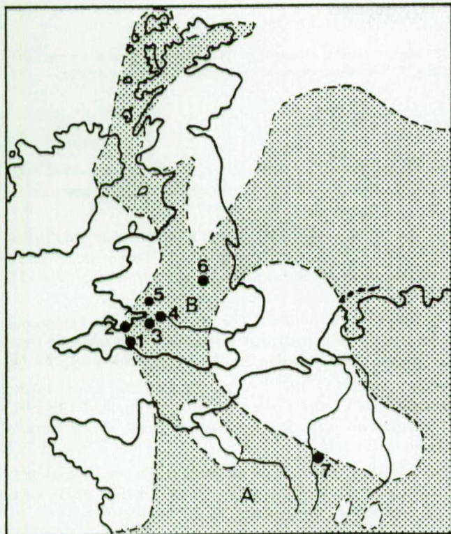
Fig. 3 — Distribution paléogéographique de Leptopterygius tenuirostris (CONYBEARE, 1822) et répartition présumée des mers et des continents au Lias inférieur. En blanc: continents; En gris: mers.
