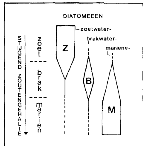
Afb. 7. Schematische weergave van de kwantitatieve verspreiding van schaaltes van respectievelijk zoetwater-, brakwater- en mariene diatomeeën in het sediment van een estuarium volgens de saliniteitsgradiënt.
