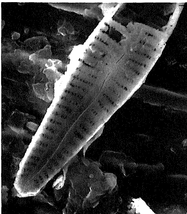
Afb. 1. Kiezelskelet van Gomphonema affine (S.E.M.). Een gedeelte van het bovenste schaal-tje is weggebroken zodat de binnenzijde zichtbaar is. Herkomst: België, Holoceen. De maatstreep bij de figuren geeft steeds 10 micrometer weer.
