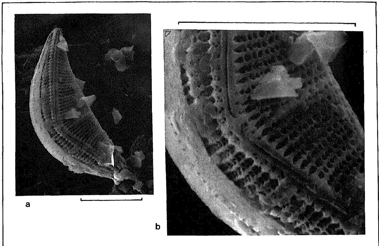
Afb. 3. Rhopalodia gibberula , een pennate diatomee (S.E.M.). a. Overzicht. b. Detailopname van het middengedeelte met de proximale raphes-uiteinden. Herkomst: België, Holoceen.
