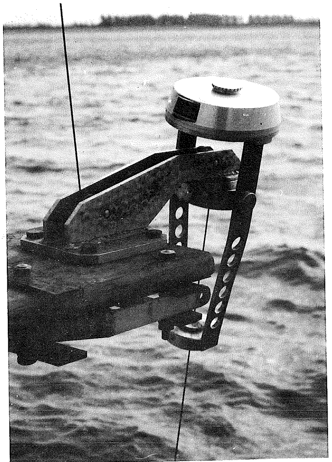
foto 12 Stroomrichtingsmeter, in bedrijf vanaf een meetschip.
