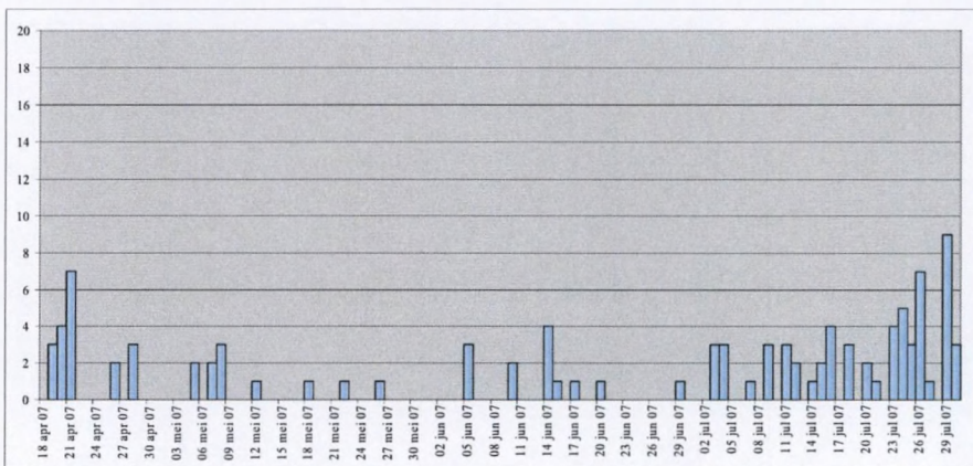
Figuur 7-21 - Aantal vaststellingen van bruinvissen per dag; verankering 18 april – 30 juli 2007
