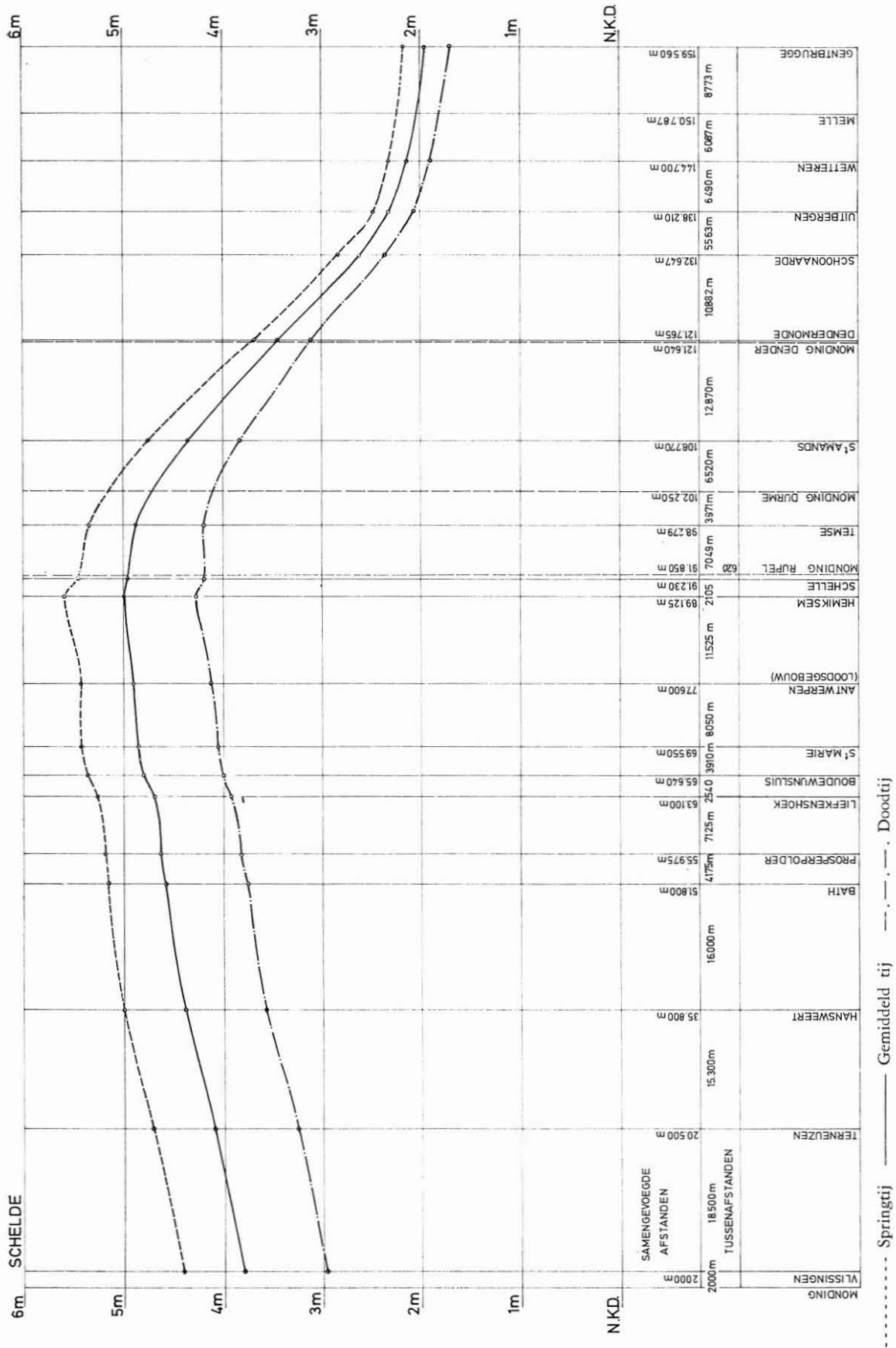
Fig. 5. — Getijamplituden voor spring-, gemiddeld- en doortij 1961 - 1970.
