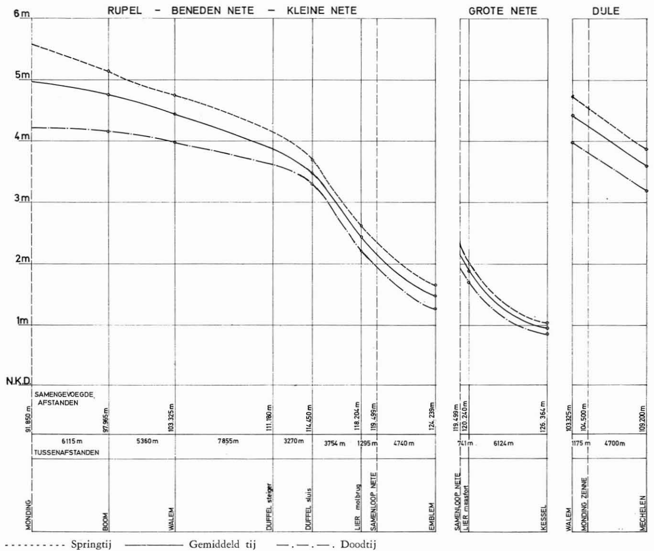
Fig. 6. — Getijamplituden voor spring-, gemiddeld- en doodtij 1961 - 1970
