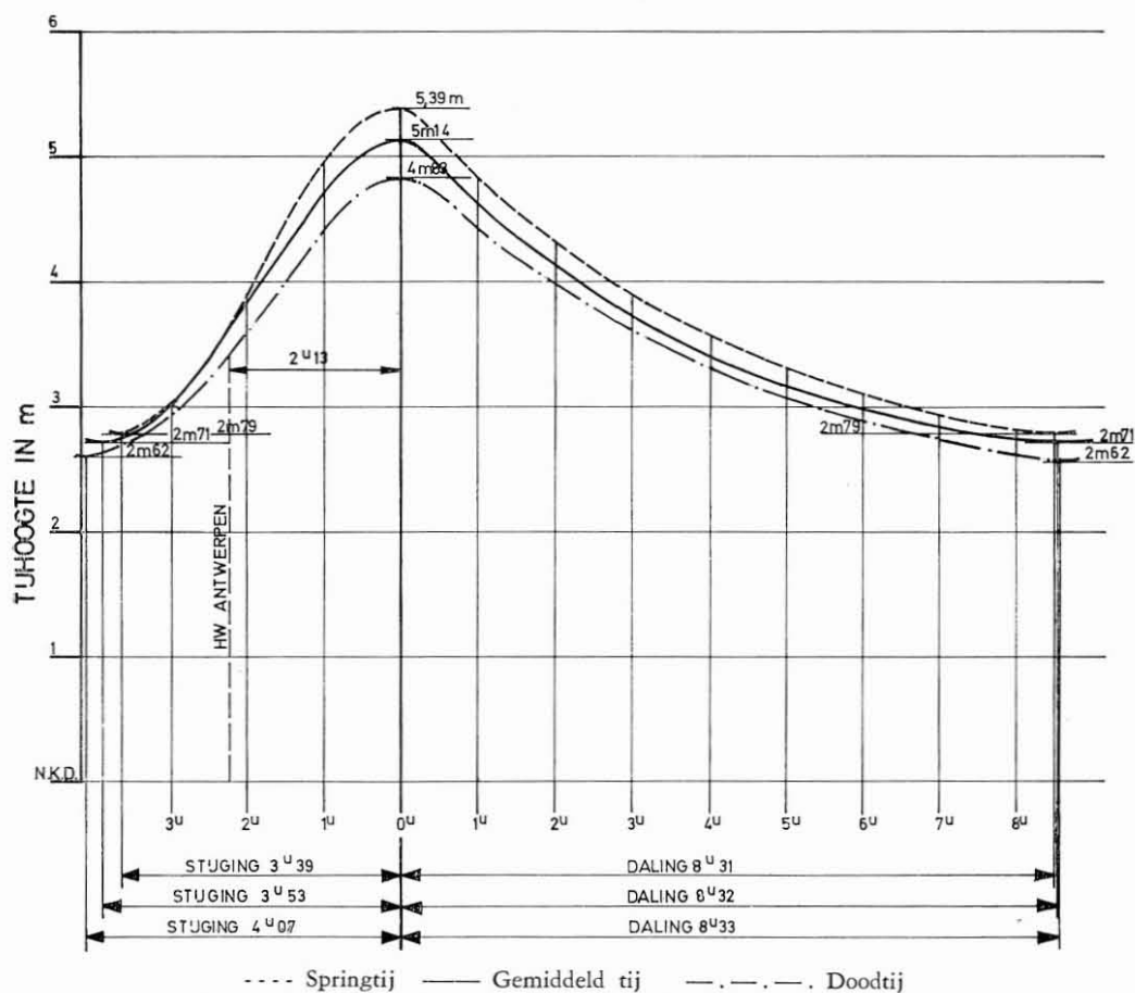
Fig. 14. — Gemiddelde tijkrommen (1961 - 1970) Benedennete - Lier (Molbrug).
