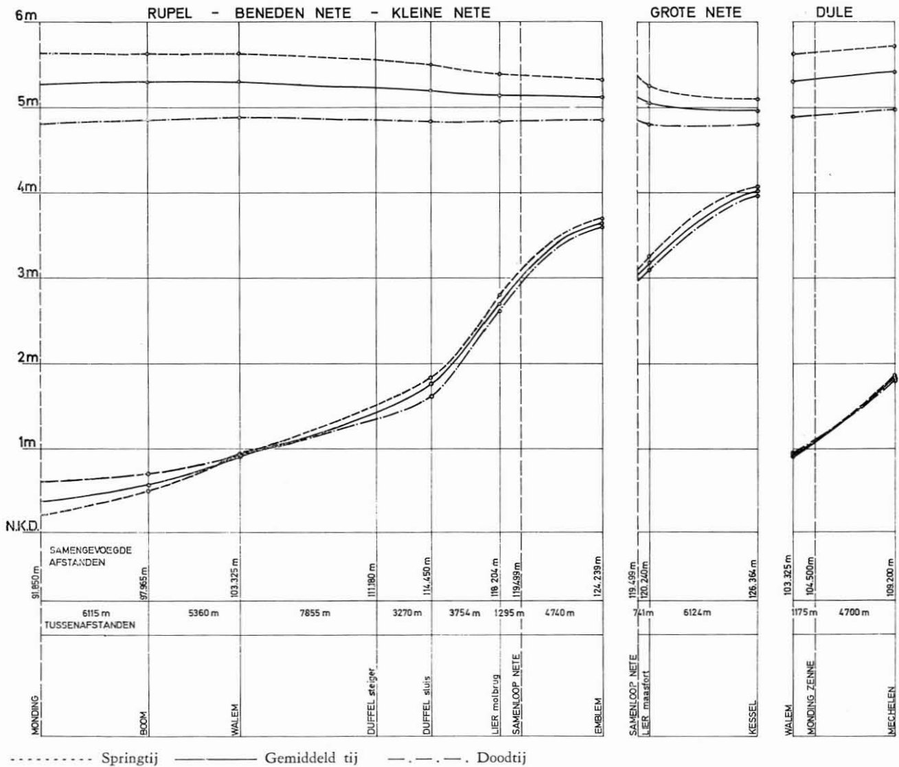
Fig. 3. — Meekundige plaatsen van hoog- en laagwaters voor spring-, gemiddeld- en doodtij 1961 - 1970.
