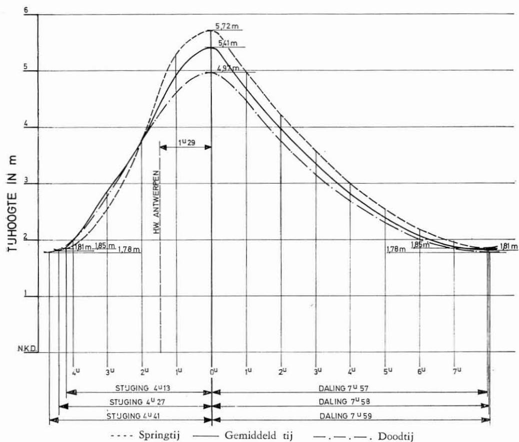
Fig. 15. — Gemiddelde tijkrommen (1961 - 1970) Dijle - Mechelen.
