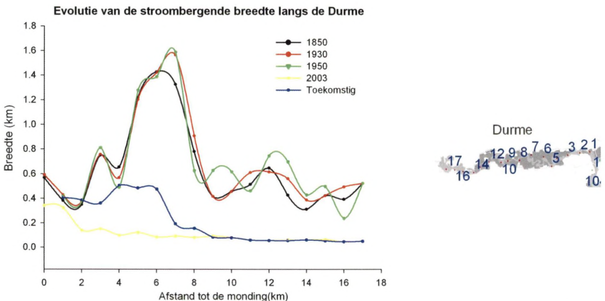
Figuur 3.86 Evolutie van de stroombergende breedte langs de Durme vanaf 1850 tot het geplande herstel in het meest wenselijk alternatief van het Sigmoplan / Evolution of storage width along the Durme from 1850 till now and the planned future scenario (MeWa)
