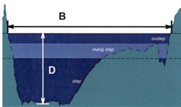
Figuur 3.92 Schematische weergave van de bepaling van de breedte-diepteverhouding / Schematical view of the determination of the storage width (B) – maximum channel depth (D) ratio
