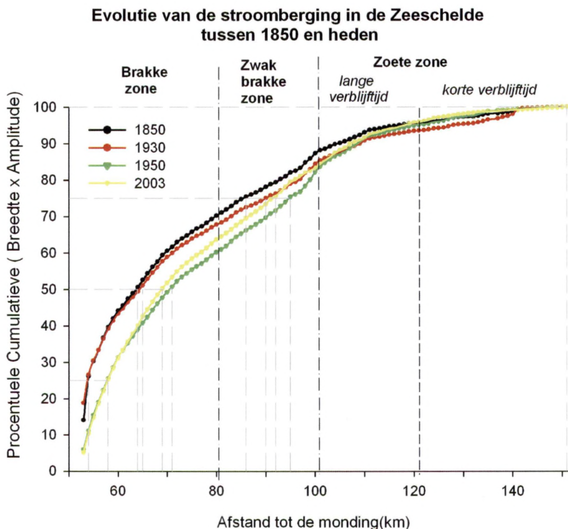
Figuur 3.90 Evolutie van de cumulatieve stroomberging langs de Zeeschelde gradiënt / Evolution of the cumulative storage capacity along the Zeeschelde
