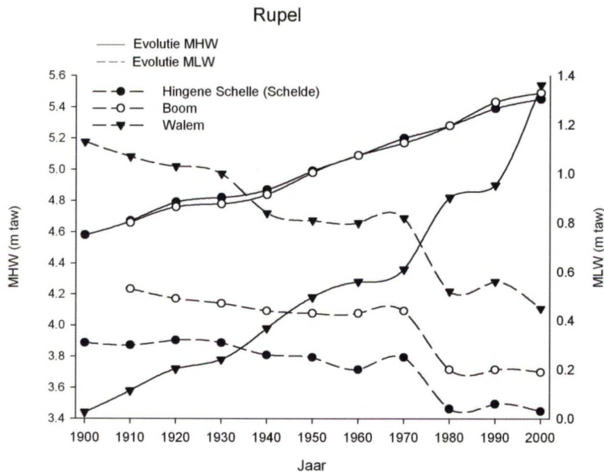
Figuur 3.48 Evolutie van de gemiddelde hoogwaterlijn (MHW) en de gemiddelde laagwaterlijn (MLW) per decennium voorafgaand het weergegeven jaar in Rupel over de periode van 1891-1900 tot 1991-2000 / Evolution of decennial mean high water and mean low water in the Rupel from 1891-1900 till 1991-2000
