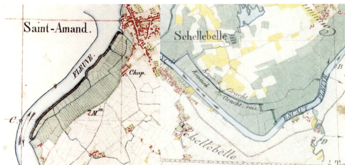
Figuur 3.28 De grote centrale afvoergrachten in de vloeisystemen bij Sint-Amands (links) en Schellebelle (Koningssloot, rechts) waren aan weerszijden aangetakt aan de Schelde en er staan geen sluizen op aangegeven / Main central drainage channels in the tidal systems at Sint-Amands (left) and Schellebelle (right) connected at both ends to the Scheldt. No sluices are indicated
