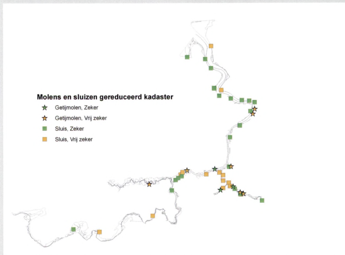
Figuur 3.54 Getijmolens en sluizen ten tijde van het gereduceerd kadaster. Zekere getijmolens zijn gedocumenteerd in de literatuur en staan aangeduid op het gereduceerd kadaster, vrij zekere getijmolens zijn gedocumenteerd maar niet aangegeven op het kadaster of vice versa. Zekere sluizen worden met het geschrift 'éclusette' en als symbool een rood haakje aangegeven, vrij zekere sluizen hebben geen geschrift maar wel een rood haakje. De precieze locatie van de getijmolen te Dendermonde kon niet achterhaald worden en is niet aangeduid op de kaart / Tidal mills and sluices in 1850. Certain tidal mills are documented in literature and mapped on the Reduced kadaster, probable tidal mills are documented but not mapped or vice versa. Certain sluices are symbolized by a red bracket and indicated on the map as 'éclusette', probable sluices are symbolized but have no accompanied writing on the map. The exact location of the tidal mill at Dendermonde remains uncertain
