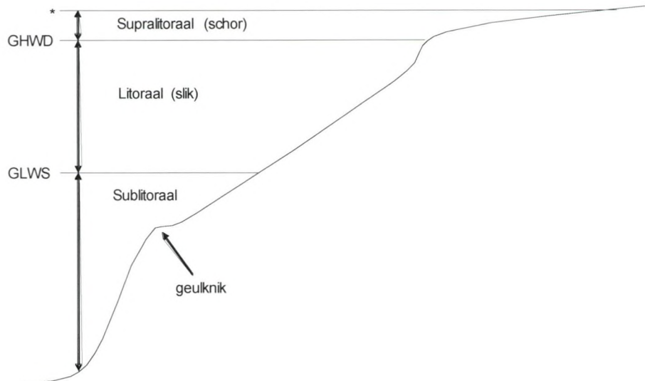
Figuur 2.4 Schema van de onder- en bovengrenzen van het litoraal, supra- en sublitoraal. GLWS=gemiddeld laagwater bij springtij, GHWD=gemiddeld hoogwater bij doortij, *=5 maal overspoeling per jaar / Schematic view of lower and upper boundaries of litoral, supralitoral and sublitoral zone. GHWD=mean high water at neap tide, GLWS=mean low water at spring tide, * = 5 times flooded per year
