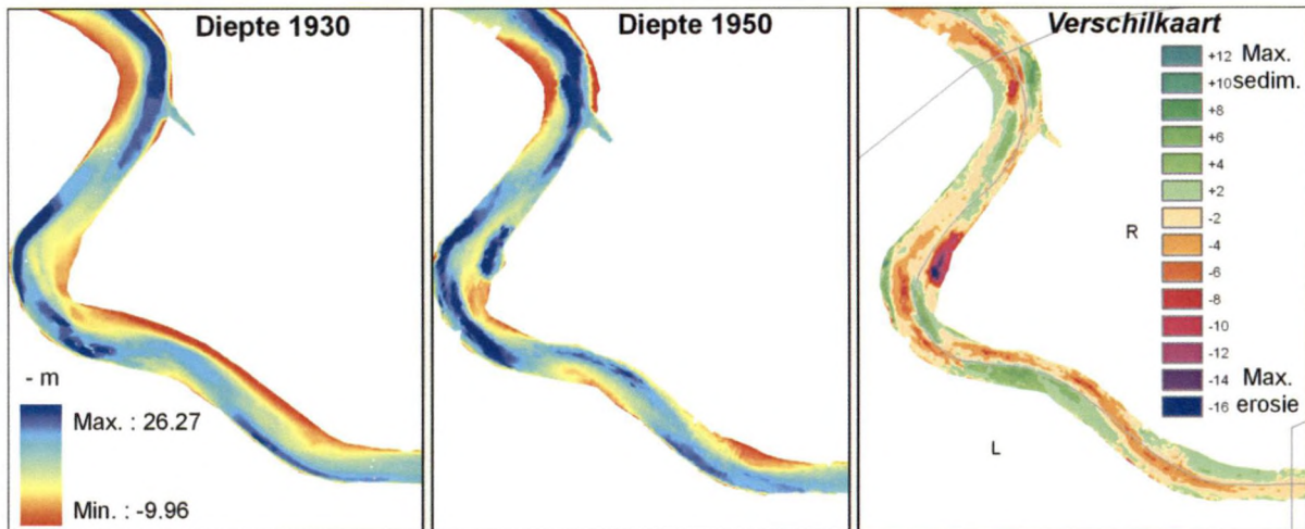
Figuur 3.8 Dieptekaart voor traject 11 in 1930 (links), 1950 (midden) en de tussentijdse netto diepte veranderingen (rechts). Bemerk de vermoedelijke zandwinning aan de plaat van de Parel / Bathymetrical map of Omes zone 11 in 1930 (left), 1950 (middle) and its nett depth changes (right). Note a possible sand exploitation effect on the mudflat of "De Parel"
