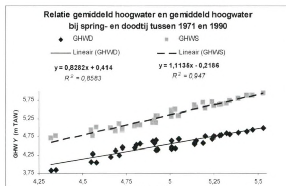
Figuur 2.6 Relatie tussen gemiddeld hoogwater bij spring- en doortij en gemiddeld hoogwater / Relationship between mean high water at spring tide and mean high water
