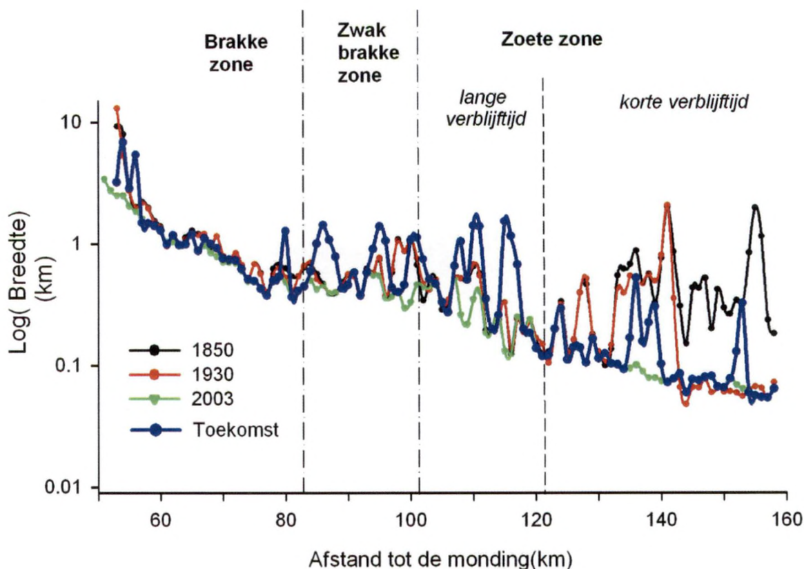
Figuur 3.81 Evolutie van de stroombergende breedte in de Zeeschelde vergeleken met het geplande herstel in het meest wenselijk alternatief van het Sigmaplan (toekomstscenario) / Evolution of storage width in the Scheldt since 1850 and the planned restoration in the MeWa
