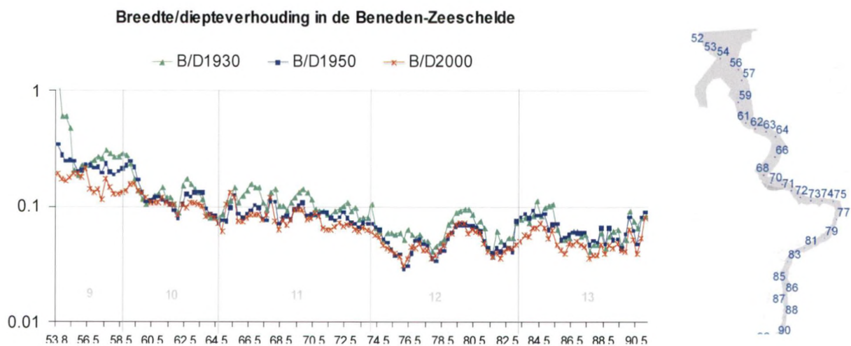
Figuur 3.93 Evolutie van de breedte-diepteverhouding in de Beneden-Zeeschelde van 1930 tot 2000 (logaritmisch) / Evolution of the width-depth ratio in the lower Zeeschelde from 1930 till 2000 (logarithmic)
