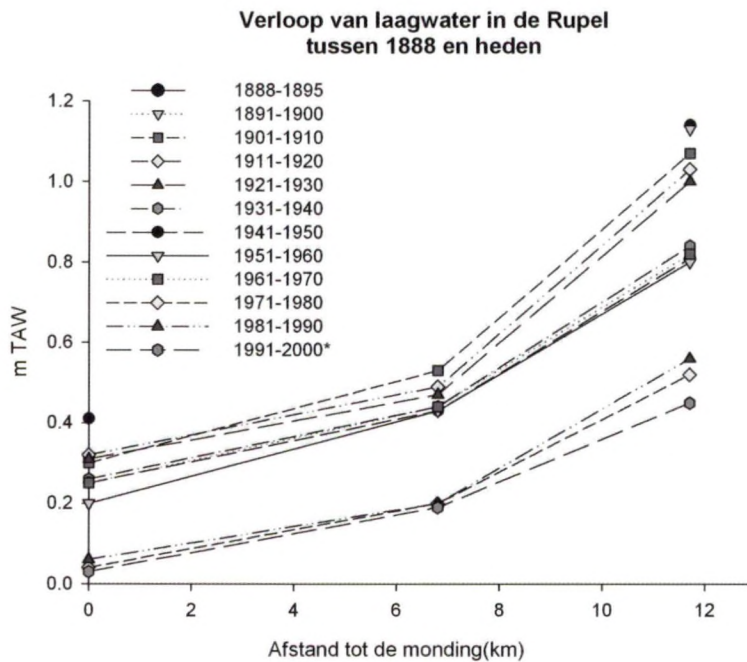
Figuur 3.47 Verloop van het gemiddeld laagwater tussen 1890 en 2000 in de Rupel/ Evolution of mean low water along the Rupel River between 1890 and 2000
