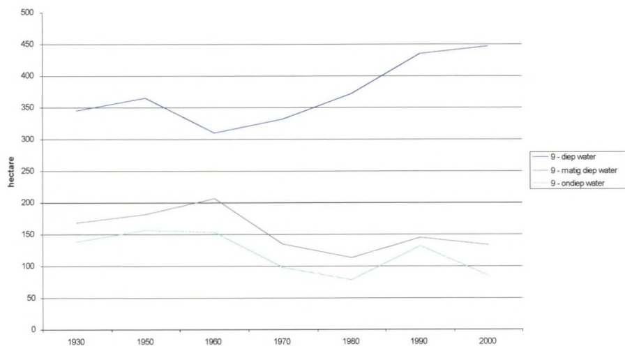
Figuur 3.2 Ontwikkelingen van het sublitoraal en naburig slik in het Omes traject 9 van 1930 tot 2003 / Evolution of the sublittoral zone and adjacent mudflat in Omes segment 9 from 1930 till 2003
