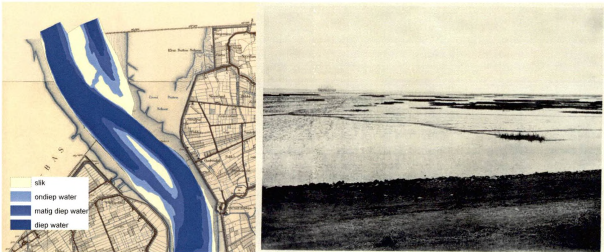
Figuur 3.12 Illustratie van het gebruik van de subtidale gegevens bij de interpretatie van de historische kaarten. De brede zone tussen de dijk en het laag slik moeten we waarschijnlijk interpreteren als een uitgestrekt pionierschor, zoals op deze foto van Massart uit 1904 nabij Zandvliet genomen bij laagtij (Massart & Bommer, 1908) / Example of the use of subtidal data for interpretation of historical maps. The broad area between dike and low tidal mudflats should be interpreted as a vast pioneer saltmarsh, as illustrated by this photograph of Massart taken in 1904 near Zandvliet at low tide.
