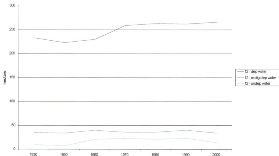
Figuur 3.5 Ontwikkelingen van het sublitoraal en naburig slik in het Omes traject 12 van 1930 tot 2003 / Evolution of the sublitoral zone and adjacent mudflat in Omes segment 12 from 1930 till 2003
