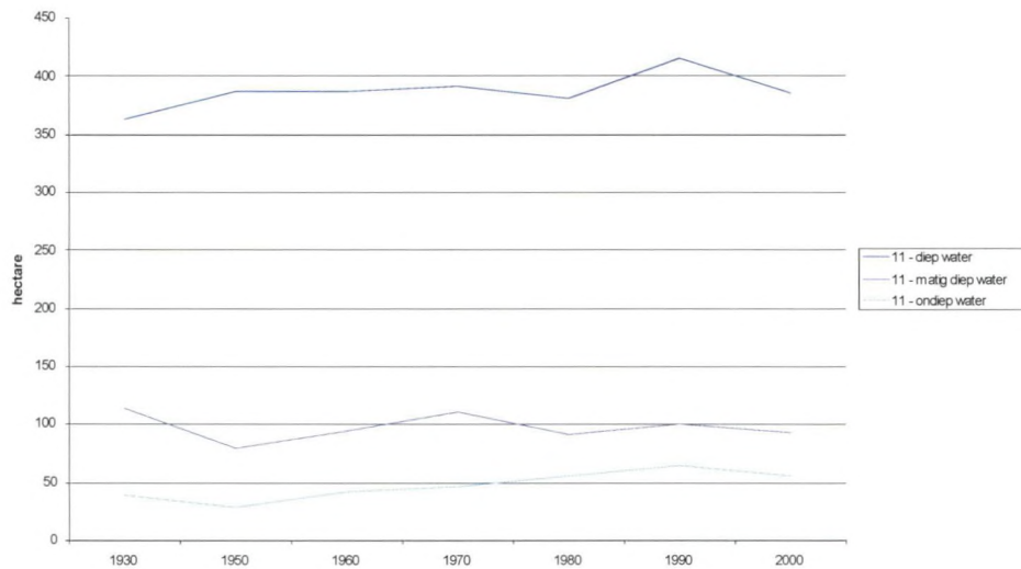
Figuur 3.4 Ontwikkelingen van het sublittoraal en naburig slik in het Omes traject 11 van 1930 tot 2003 / Evolution of the sublittoral zone and adjacent mudflat in Omes segment 11 from 1930 till 2003
