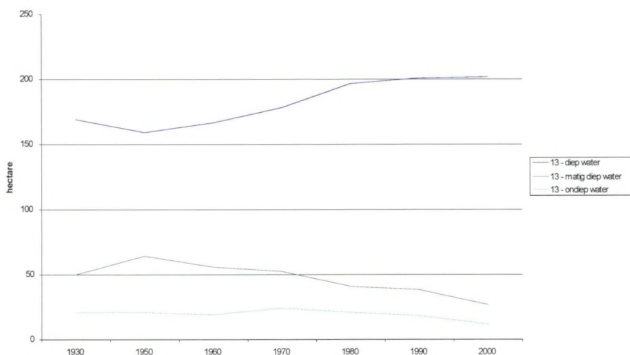
Figuur 3.6 Ontwikkelingen van het sublittoraal en naburig slik in het Omes traject 13 van 1930 tot 2003 / Evolution of the sublittoral zone and adjacent mudflat in Omes segment 13 from 1930 till 2003
