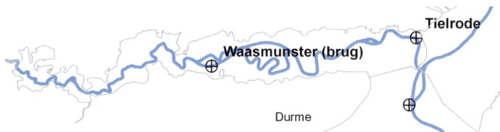
Verloop van hoogwater in de Durme tussen 1888 en heden
