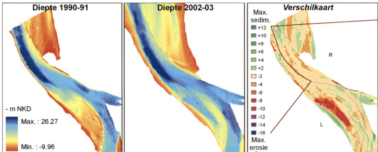
Figuur 3.9 Dieptekaart voor traject 9 in 1990-91 (links) en 2002-2003 (midden) en tussentijdse netto diepte veranderingen (rechts) / Bathymetrical map of Omes zone 9 in 1990-1991 (left) and 2002-2003 (middle) and the intervening nett depth changes (right).
