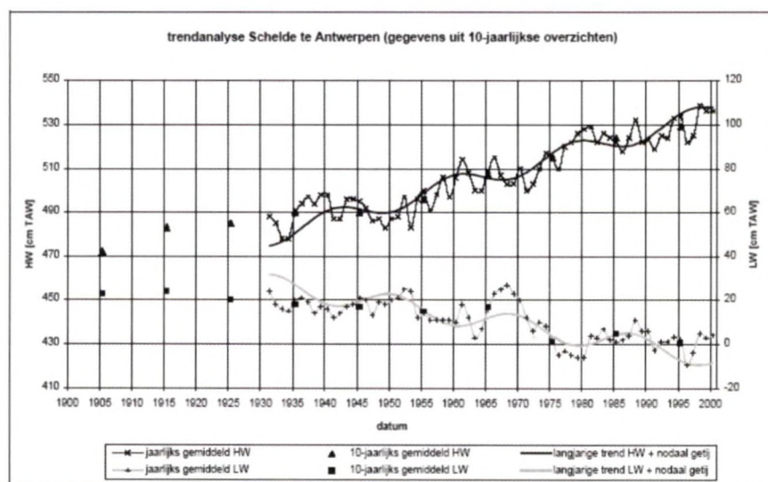
Figuur 2.12 Vergelijking jaargemiddelden en tienjarige gemiddelden voor Antwerpen uit Blanckaert (2003)/ Comparison of annual and decade means at Antwerp (from Blanckaert, 2003)
