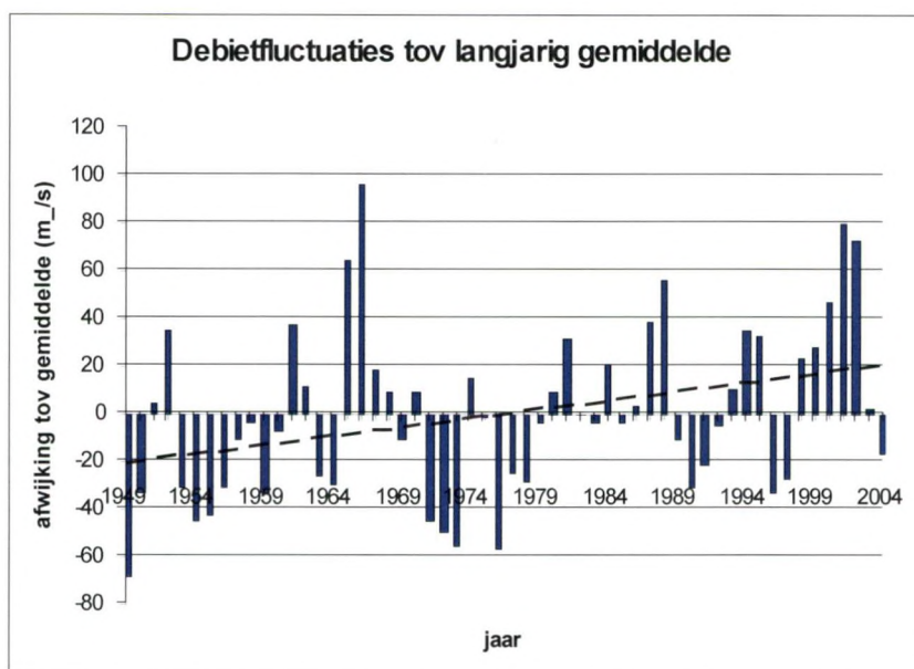
Figuur 3.59 Afwijking van het jaarlijks afvoerdebiet van de Schelde te Schelle ten opzichte van het langjarig gemiddelde (Gegevensbron: Ministerie Vlaamse Gemeenschap - Waterbouwkundig Laboratorium - Borgerhout) / Deviation on long-term mean of annual discharge of the Scheldt at Schelle (source: Ministerie Vlaamse Gemeenschap - Waterbouwkundig Laboratorium - Borgerhout)
