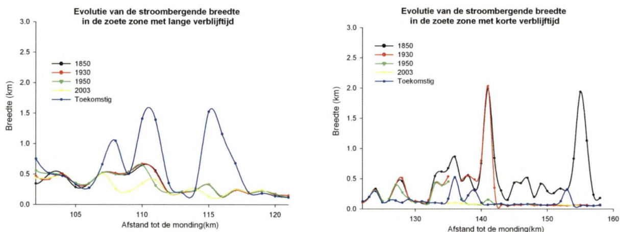
Figuur 3.83 Evolutie van de stroombergende breedte in de zoete zone vanaf 1850 tot 2003 samen met het toekomstig meest wenselijk alternatief van het Sigmoplan; a) zoete zone met lange verblijftijd, b) zoete zone met korte verblijftijd. / Storage width in the fresh water part of the Scheldt around 1930, 2003 and the planned future scenario; a) long retention zone, b) short retention zone
