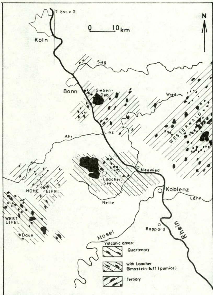
Fig. 9 - Volcanic products in the Rhenisches Schiefergebirge
