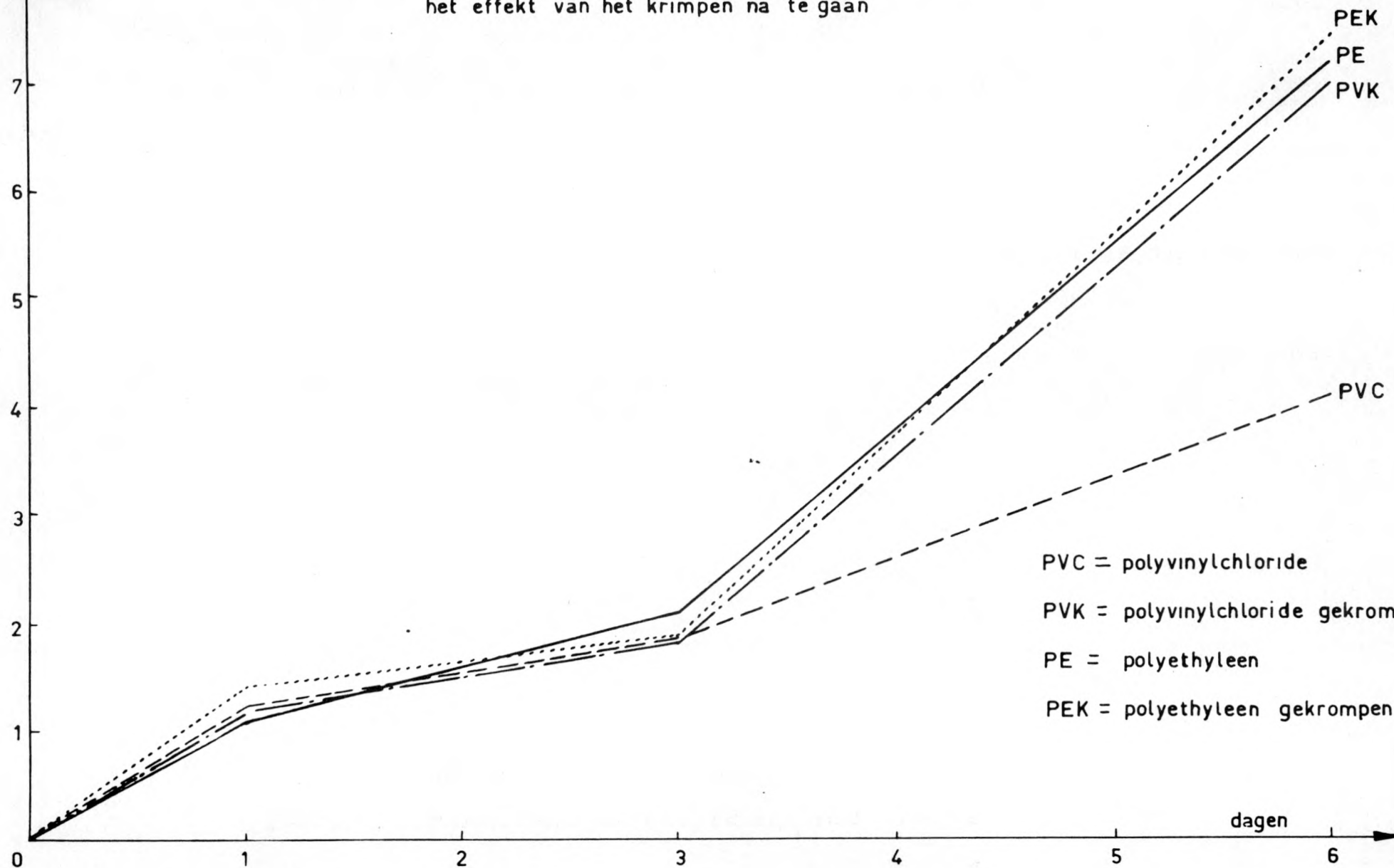
Figuur 20 - TMA-bepalingen op de vis die is aangewend om het effect van het krimpen na te gaan
