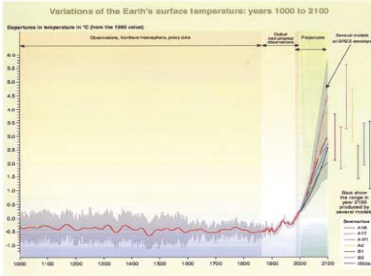
Figuur 1: Historische en toekomstig voorspelde variaties in de mondiale gemiddelde oppervlaktetemperatuur [IPCC, 2001].
