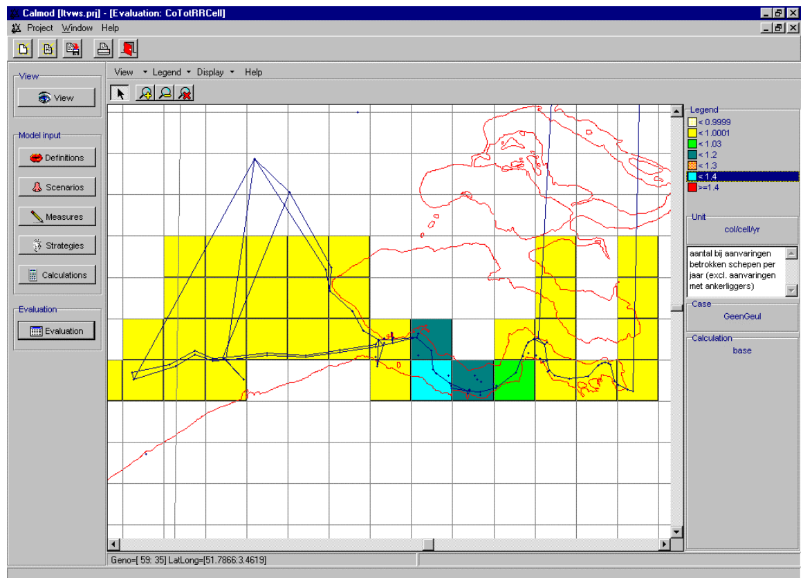
Figuur 9.2 Verandering van het aantal bij aanvaringen betrokken schepen indien de nevengeulen Everingen en de Schaar van Spijkerplaat niet meer gebruikt mogen worden
