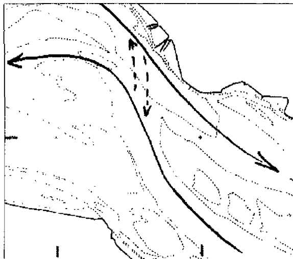
Figuur 3.6 Ontwijkend ebgeul-type (Drempel van Borssele, 1994)
