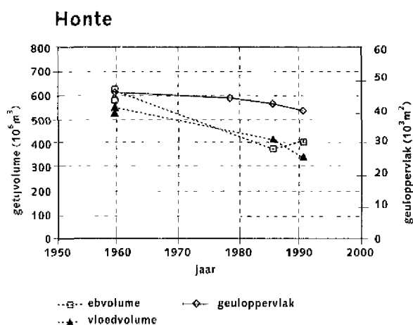
Figuur 3.7 Verloop van getijvolume en geuloppervlak voor de Honte en de Schaar van Spijkerplaat
