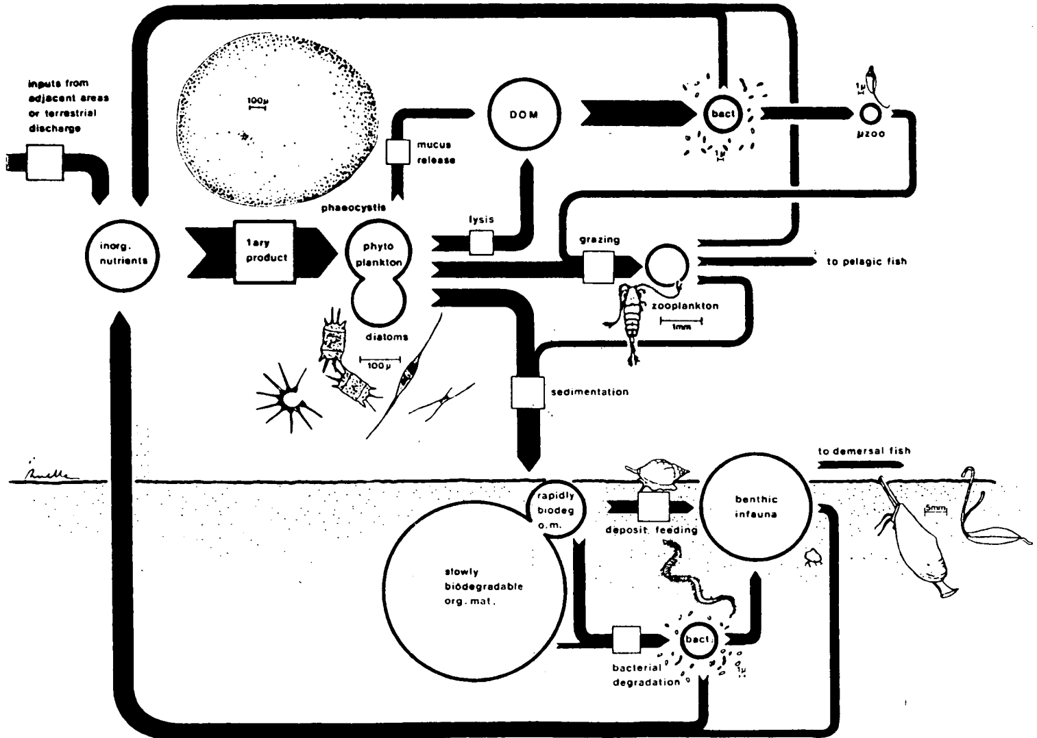
Fig.16 Schematische voorstelling van de dominante fluxen van nutriënten doorheen de eerste trofische niveau's van de voedselketen van een kustecosysteem (lit.25).
