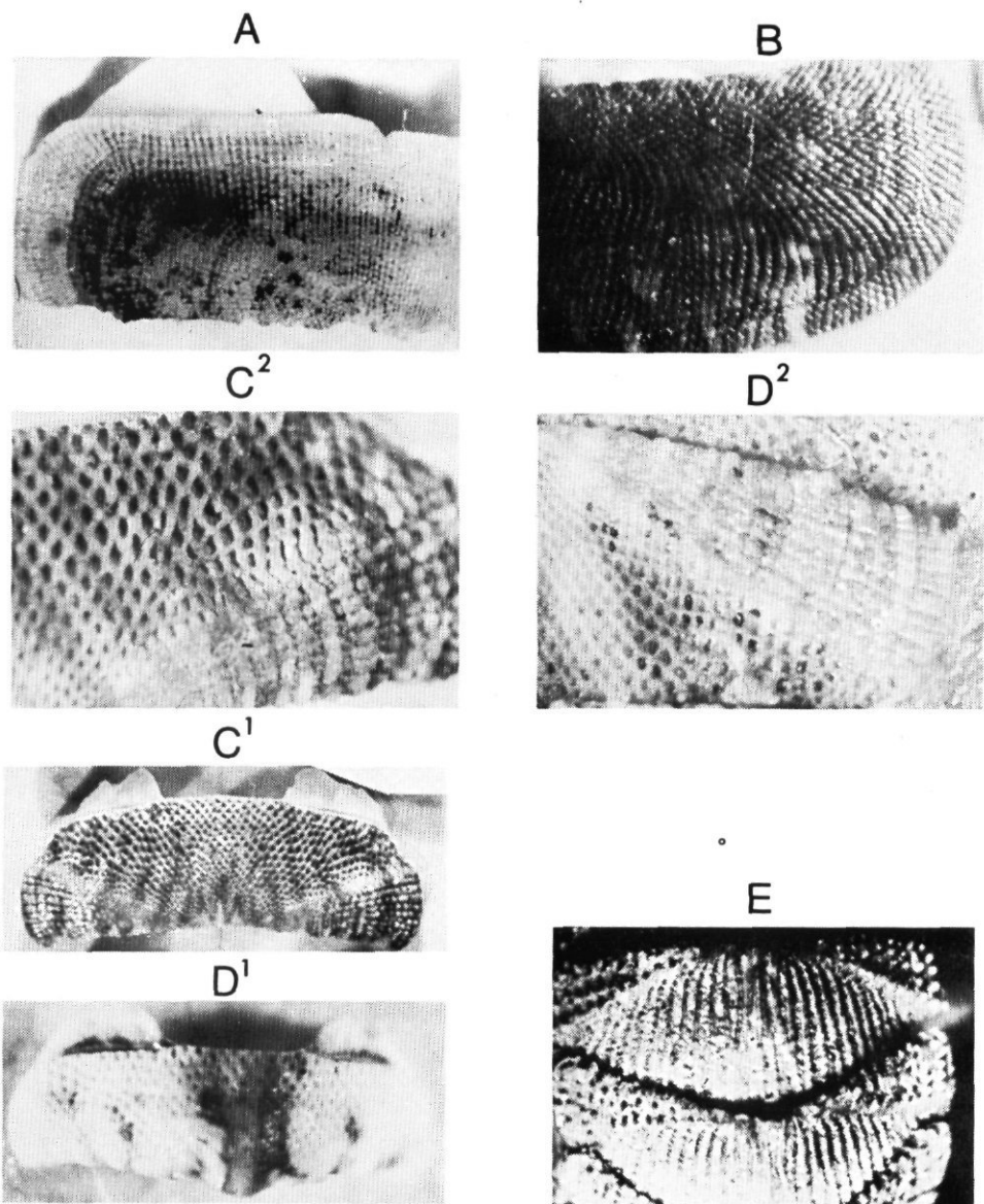
Fig. A. Lepidopleurus algesirensis Capellini, 1859. Côtes du Maroc, valve V; \times 12,5 .
