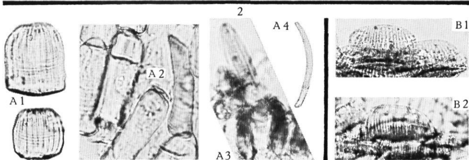
Fig. 1. Ischnochiton cessaci (Rochebrune, 1881).
