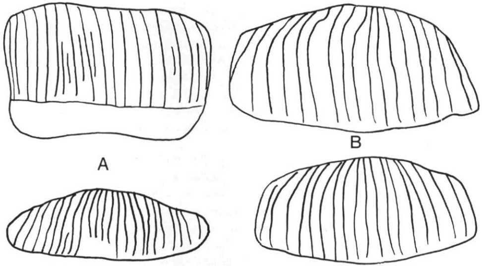
Fig. 9. Ecailles de la face supérieure; \times 270 . A, Ischnochiton tigrinus Krauss, 1848; Natal. B, Ischnochiton textilis (Gray, 1878); Port Elizabeth.
