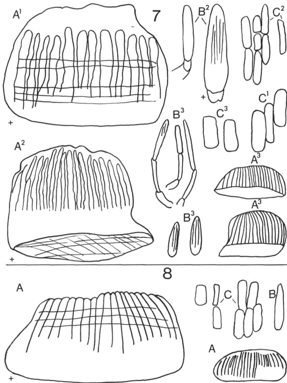
Fig. 7, 8. Éléments de la ceinture; \times 270 (+: \times 540 ).
