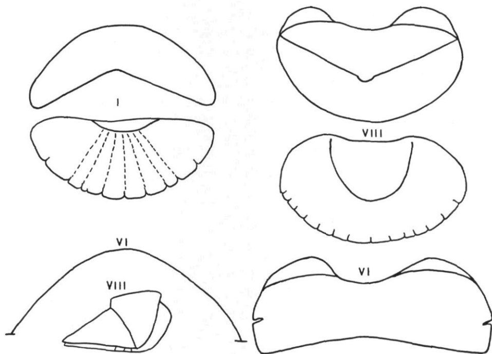
Fig. 3. Ischnochiton cessaci (Rochebrune, 1881). Praia Azul, contours des valves; \times 7,5 .
