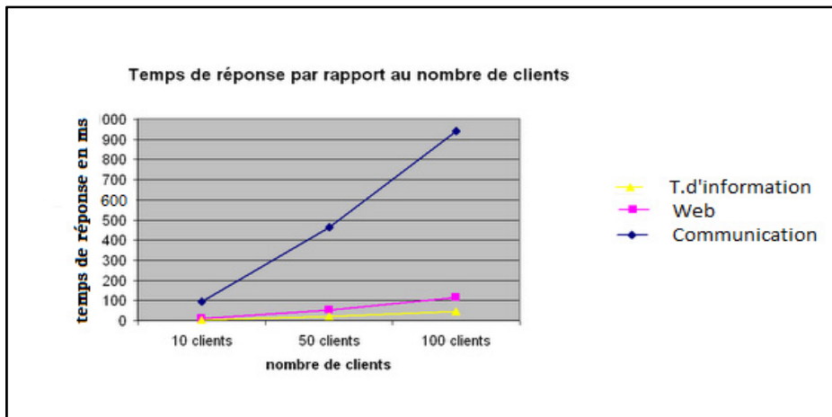
Figure 3.10 Temps de réponse par rapport au nombre de clients
