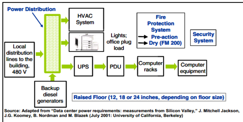
Figure 1.3 Architecture physique d'un centre de données Tirée de Bell (2005)
