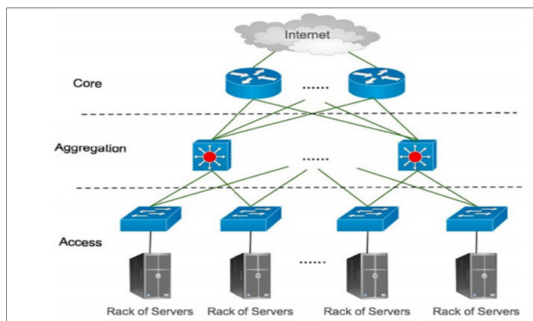
Figure 1.2 Conception en couche de l'infrastructure de réseau de centre de données Tirée de Zhang et al. (2010)
