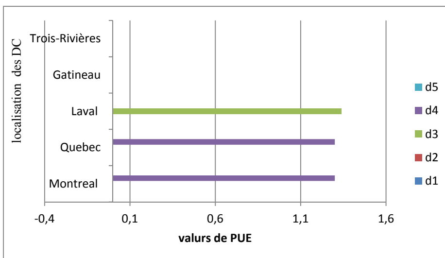
Figure 3.9 Valeurs des PUE pour chaque centre de données
