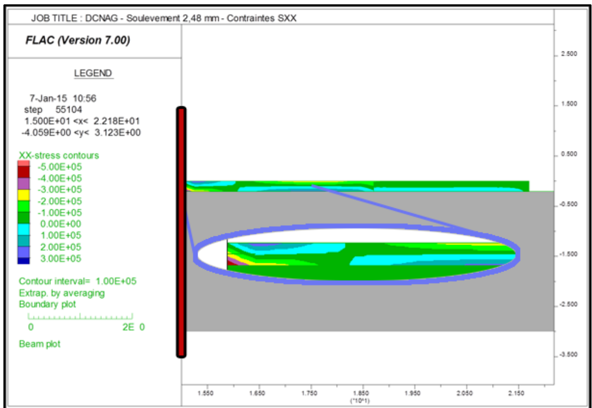
Figure 6.11 Contraintes en tension et en compression dans le revêtement de dalles courte armées goujonnées lors d'un soulèvement de 2,48 mm
