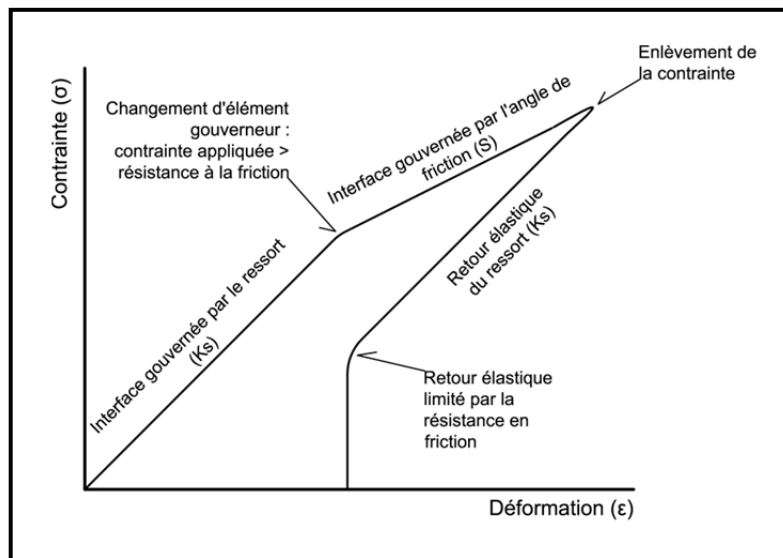
Figure 4.8 Transfert de contraintes horizontales Adaptée de Itasca (2011)
