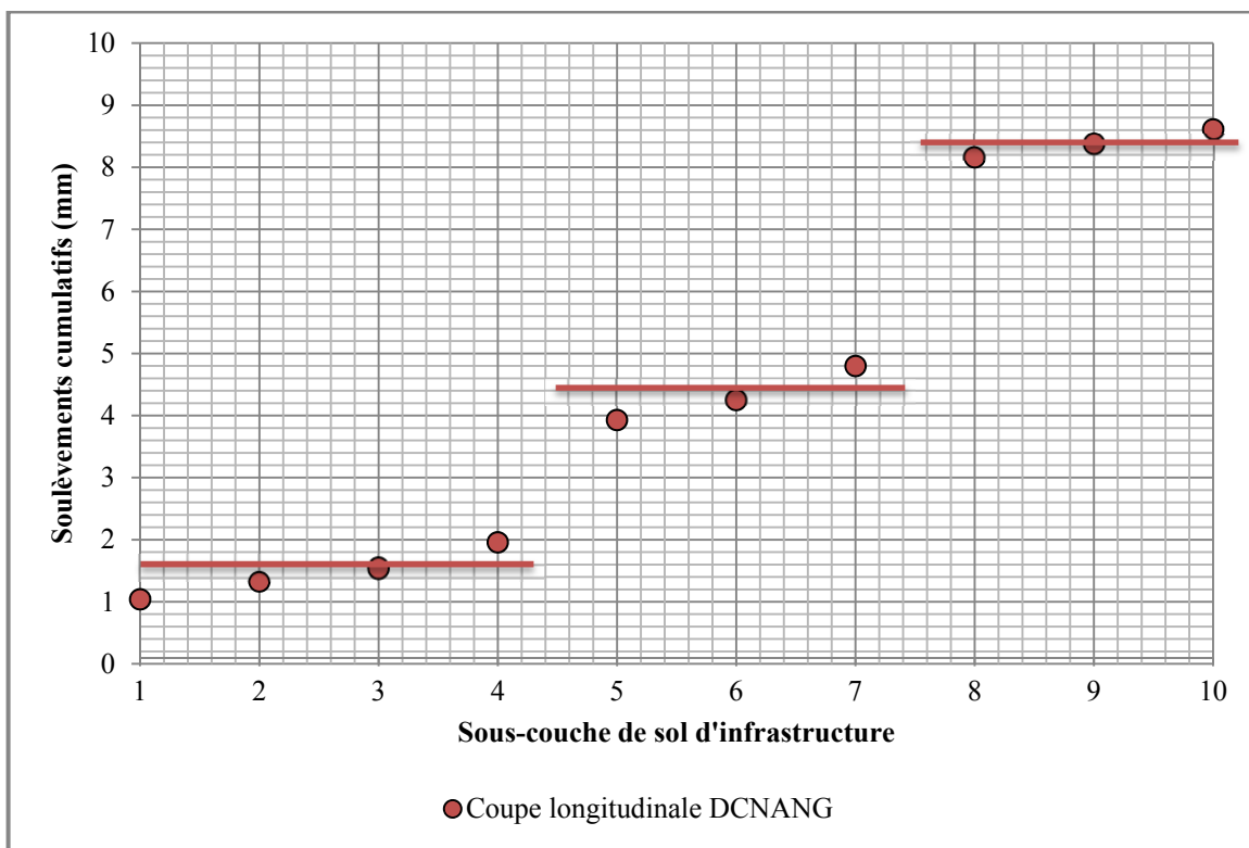
Figure 6.8 Soulèvements cumulatifs par sous-couche en utilisant l'approche par contraintes imposées pour la coupe longitudinale de DCNANG
