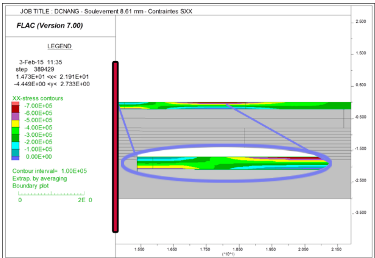
Figure 6.7 Contraintes en tension et en compression dans le revêtement DCNANG lors d'un soulèvement de 8,61 mm en utilisant l'approche de contraintes imposées
