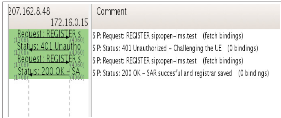
Figure 5.6 Procédure d'enregistrement Cloud OpenIMS
