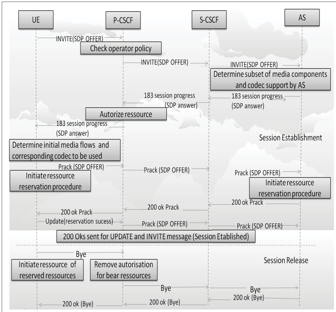
Figure 2.6 Signalisation et négociation de la QoS dans IMS (SIP/SDP) Tirée de Skorin-Kapov et al. (2007)
