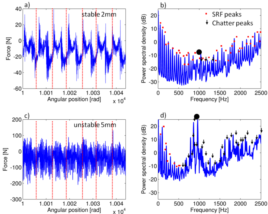
Figure 51 -Représentation angulaire et spectrale (PSD) des signaux de force dans la direction axiale F_z . (a,b) Conditions stables (3000rpm, 2mm, N 2 dents). (c,d) Conditions instables (3000rpm, 5mm, N 2 dents). Les points rouges caractérisent la fréquence de rotation de la broche et ses harmoniques. Les flèches noires dénotent les fréquences excitées liées au broutage. Les disques noirs montrent les résonances.
