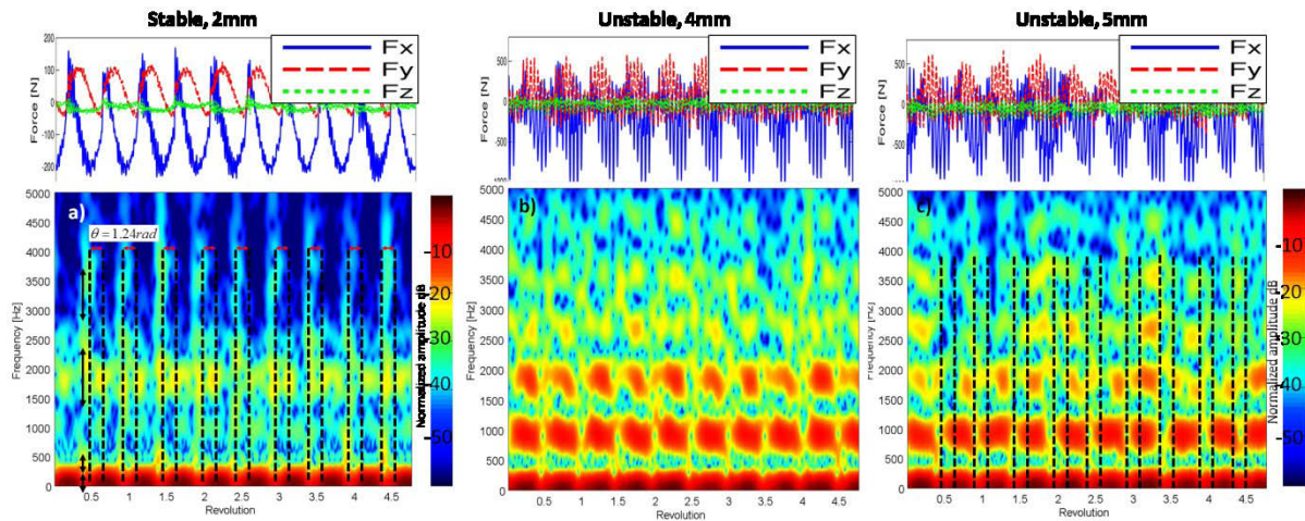
Figure 52 -Représentation angle fréquence de signaux de force résultante. (a) Conditions stables - 3000rpm et 2mm. (b) conditions instables 3000rpm et 4mm. (c) Conditions instables 3000rpm et 5mm.
