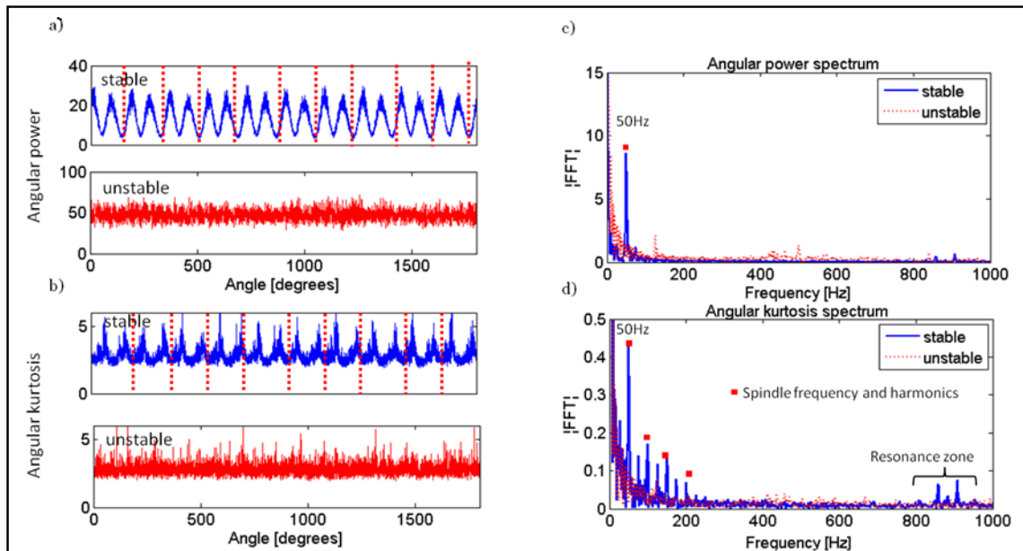
Figure 36 -(a,b) Puissance et Kurtosis angulaires dans les conditions stables (3000rpm, 3mm) et instables (3000rpm, 5mm) calculés sur 10 cycles et 300 blocs. (c,d) Spectre de puissance et du Kurtosis angulaires dans les deux conditions. Les points rouges dénotent la fréquence de rotation de la broche et ses harmoniques.
