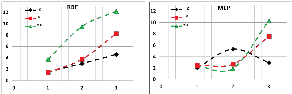
Figure 70 -Taux d'erreur de classification des trois scénarios.
