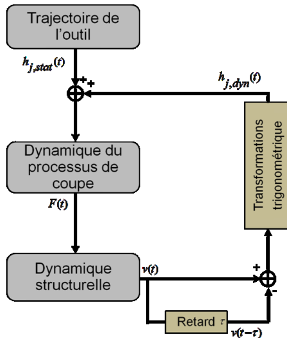
Figure 2 - Diagramme en bloc du processus d'usinage.
