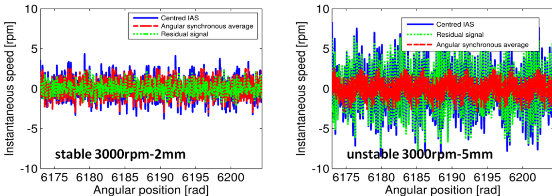
Figure 61 -Décomposition du signal de vitesse instantannée.
