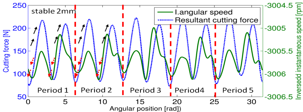
Figure 53 -Corrélation entre la force de coupe et la vitesse instantanée (inversée). La figure montre 5 rotations de la broche. Les deux signaux sont filtrés LPF (low pass filter) avec une fréquence de coupe de 230 Hz. La flèche noire montre l'augmentation de la force résultante quand la dent entre dans la matière. La flèche rouge montre le comportement du signal de vitesse.
