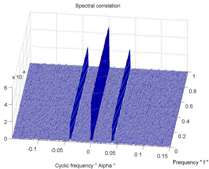
Figure 15 -Fonction de corrélation cyclique d'un signal modulé en amplitude. Cette fonction n'est pas nulle pour les fréquences cycliques \alpha = 0 et \alpha = \pm 2f_0 .
