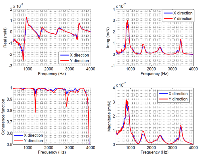
Figure 24 -Les fonctions de transfert suivant les axes x et y.
