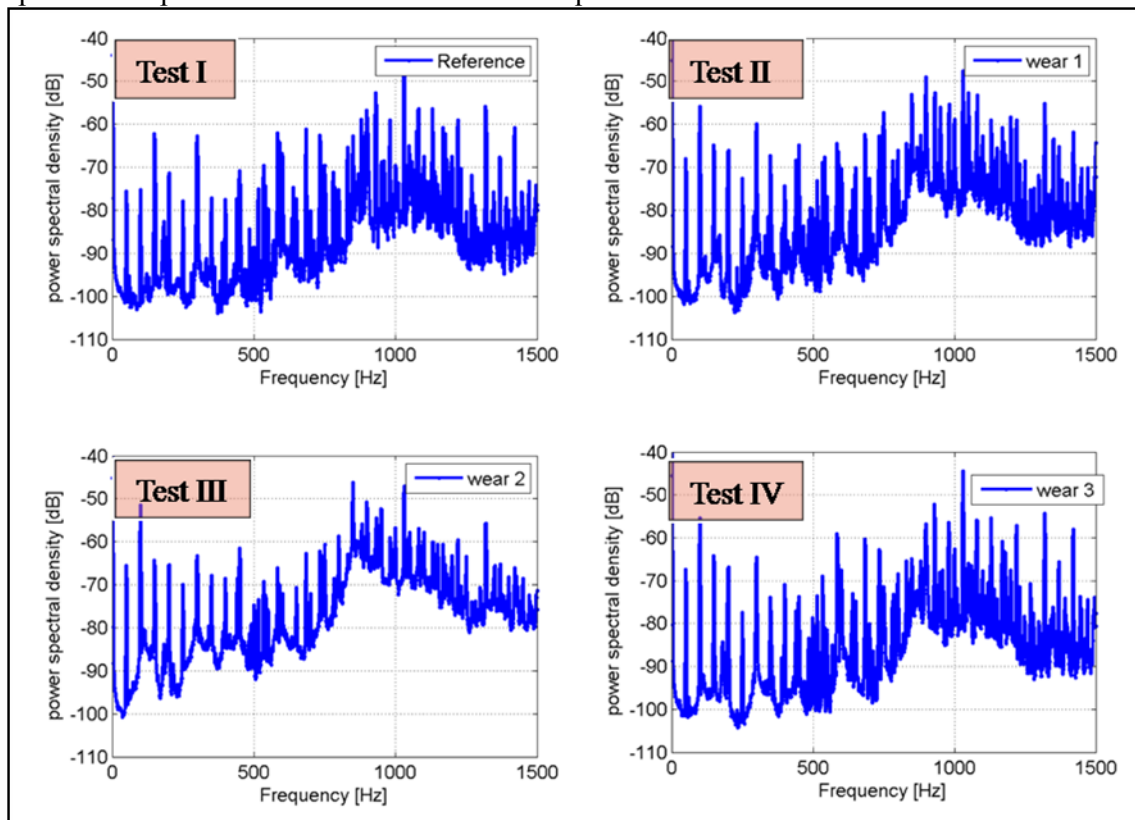
Figure 41 Densité spectrale de puissance de l'usure de l'outil de coupe pour les quatre scénarios.
