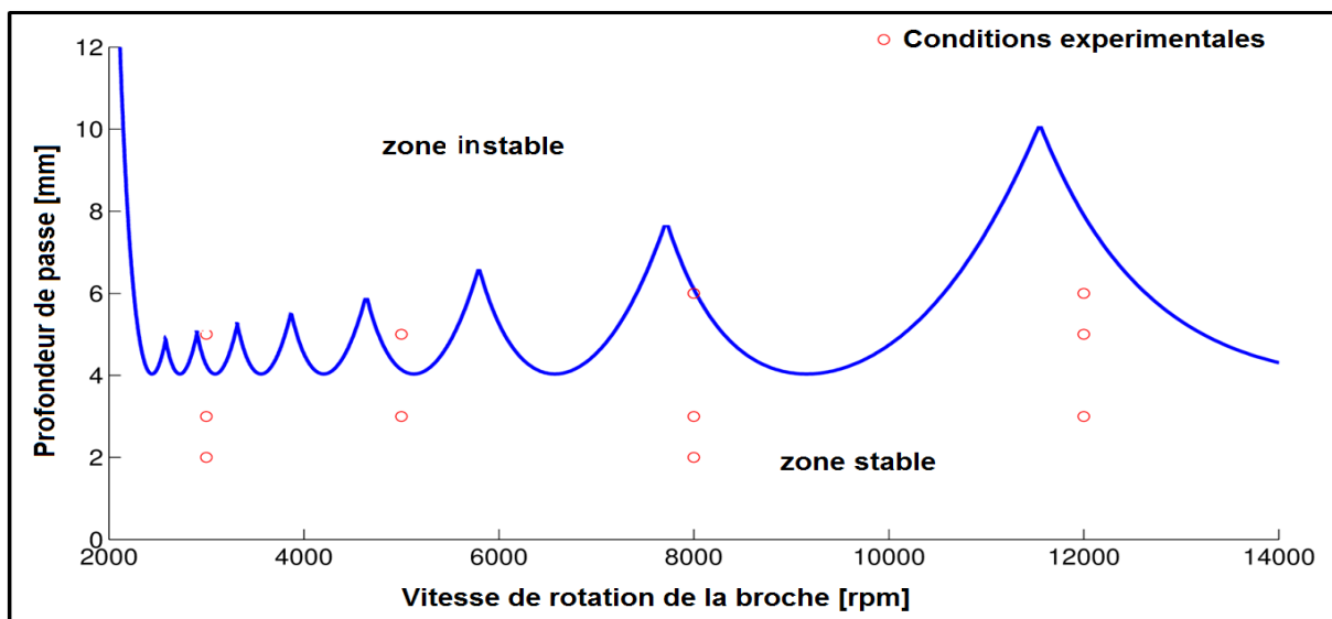
Figure 26 -Les conditions de coupe choisies à partir des lobes de stabilité. Diagramme des lobes de stabilité simulé pour : Un outil de 2 dents/ Opération de rainurage/ Aluminium A7075T6/ Centre d'usinage Horon/ Système outil porte outil broche flexible.
