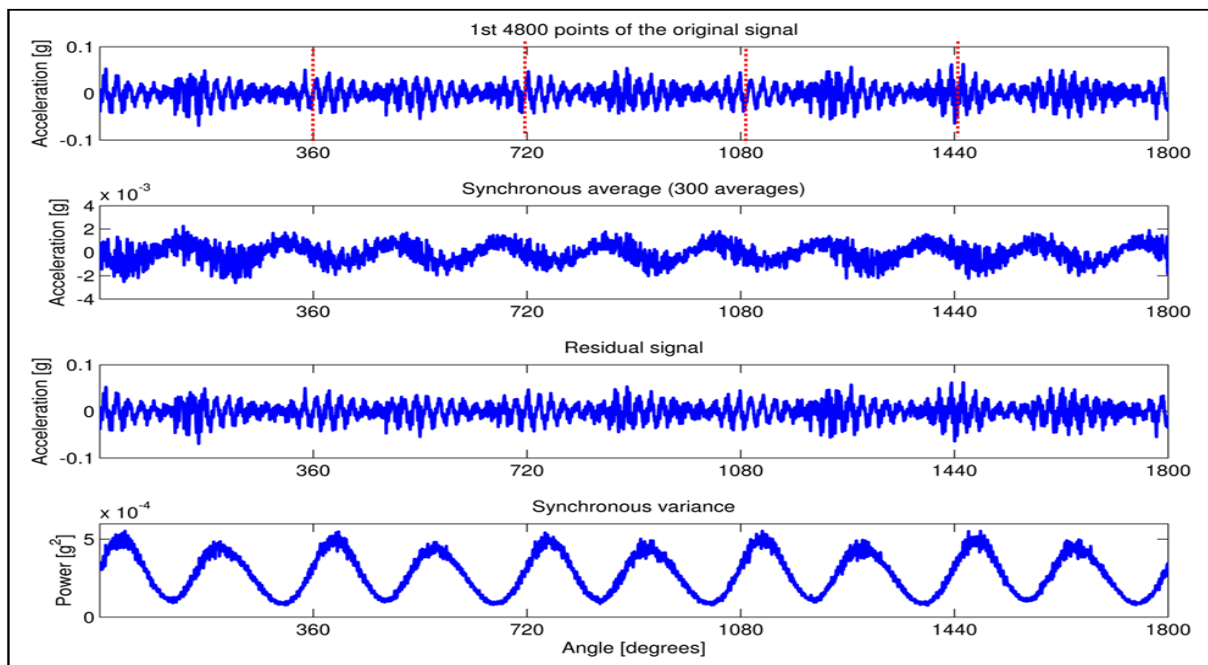
Figure 34 -Statistiques synchrones du premier et second ordre, estimés sur 300 cycles.
