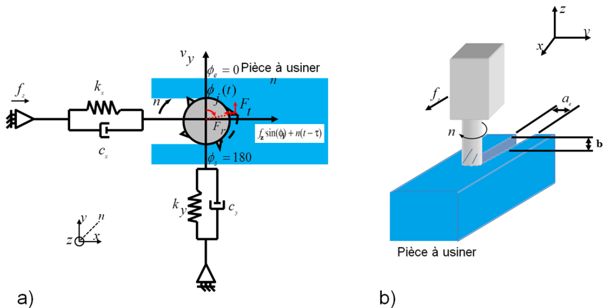
Figure 1 Représentation schématique du processus d'usinage (fraisage en rainure). a) vue en dessus, b) vue en 3D.
