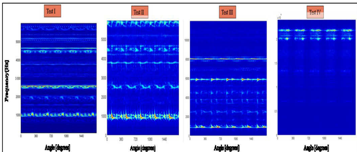
Figure 43 -Spectres de WignerVille pour les quatre scénarios.
