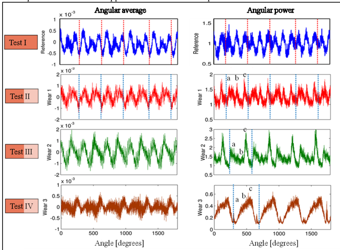
Figure 42 -Moyenne et puissance angulaires estimées sur 300 cycles pour les quatre scénarios. a, b et c indiquent le passage de chaque dent de l'outil.
