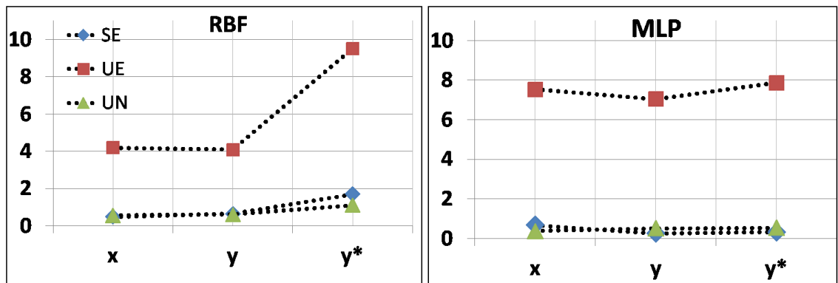
Figure 69 -Taux d'erreur de classification en utilisant les réseaux de neurones MLP et RBF selon trois positions.
