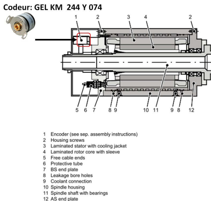
Figure 45 -Positionnement du codeur dans la broche de Huron K2X10 (site du constructeur).
