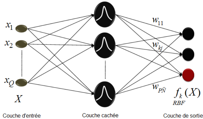
Figure 67 -Architecture de réseaux RBF.
