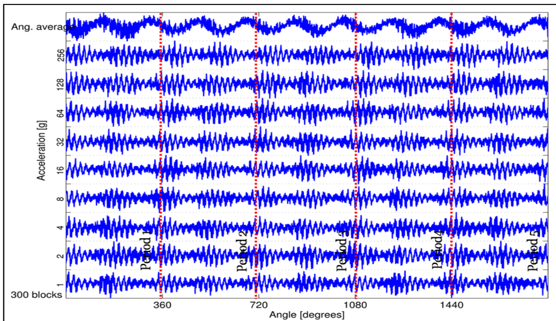
Figure 33 -Principe de la moyenne angulaire synchrone estimée sur 300 blocs de 5 cycles.
