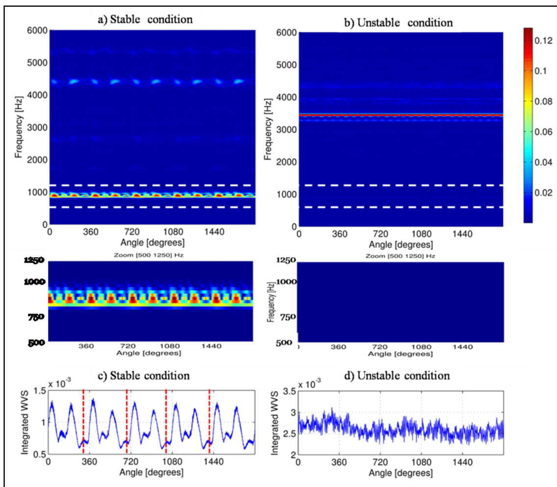
Figure 40 -(a,b) Spectres de WignerVille dans les conditions stables et instables, avec zoom. (c,d) Spectres de WignerVille intégrés.
