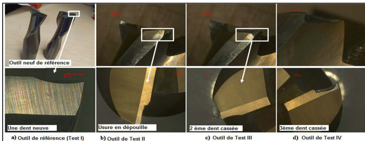
Figure 28 -Les photographies microscopiques des outils utilisés pour réaliser les quatre scénarios (I,II,III,IV).
