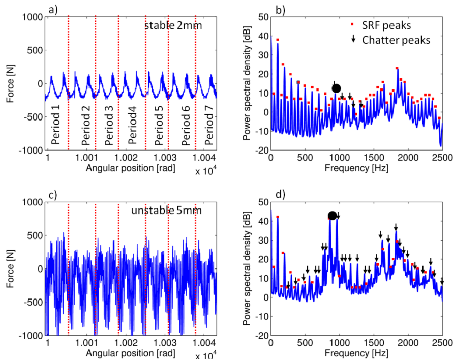
Figure 50 -Représentation angulaire et spectrale (PSD) des signaux de force dans la direction perpendiculaire à la direction d'avance FNf . (a,b) Conditions stables (3000rpm, 2mm, N 2 dents).
