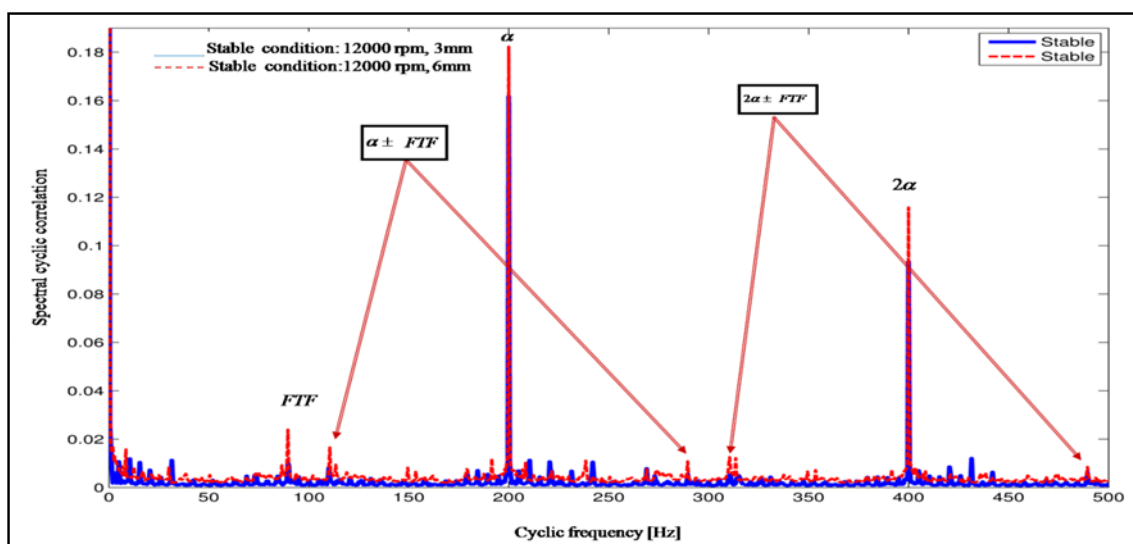
Figure 39 -Densité spectrale cyclique intégrée dans les conditions stables (courbe en bleu) et instables (courbe en rouge). FTF=89.5 Hz
