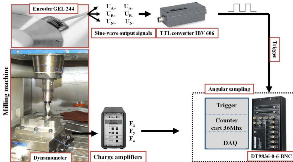
Figure 47 -Dispositif expérimental angulaire.
