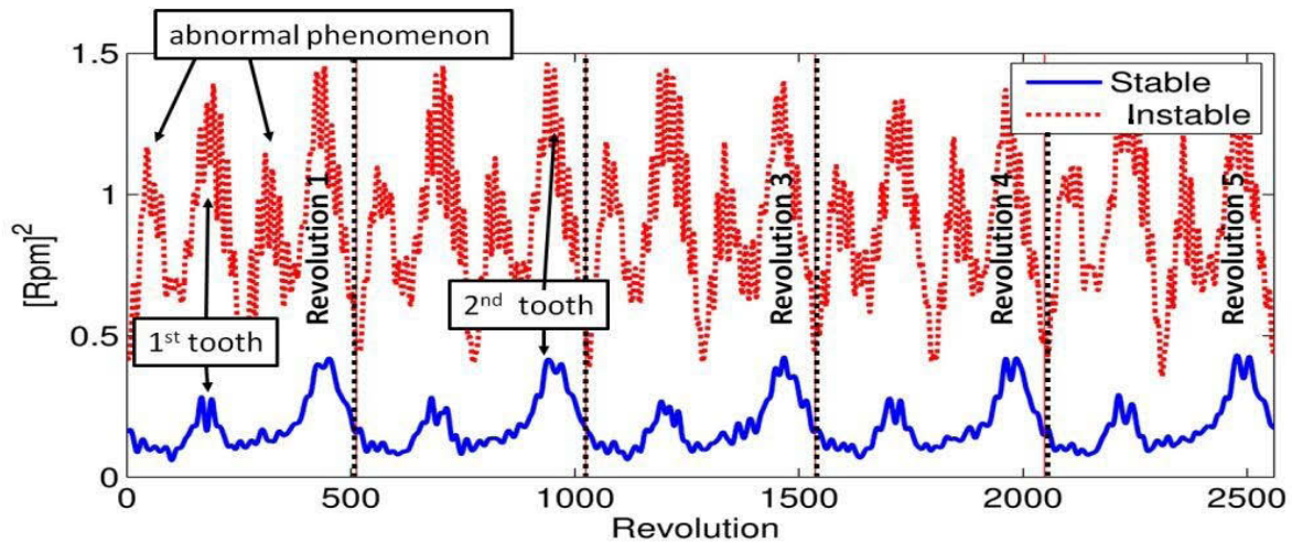
Figure 58 -Variance angulaire synchrone des signaux de vitesse pour les cas stable (bleu continue) et instable (rouge pointillée).
