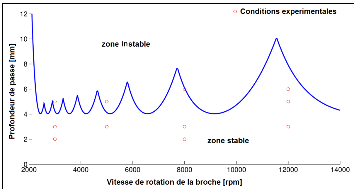
Figure 25 - Diagramme des lobes de stabilité simulé pour : Un outil de 2 dents/ Opération de rainurage/ Aluminium A7075T6/ Centre d'usinage Horon/ Système outil porte outil broche flexible.
