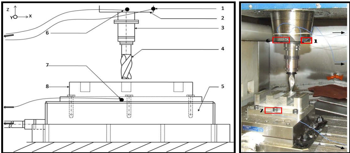
Figure 22 -Schématisation du dispositif expérimental (1) accéléromètre 1 (PCB352C22) (2) partie non rotative de la broche (3) porte outil (4) outil à deux ou trois dents (5) table dynamométrique [9255B] (6) accéléromètre 2 (PCB352C22) (7) accéléromètre 3 (PCB352C22) (8) pièce d'aluminium AA7075T6. Les flèches indiquent le transfert des données vers le système d'acquisition.
