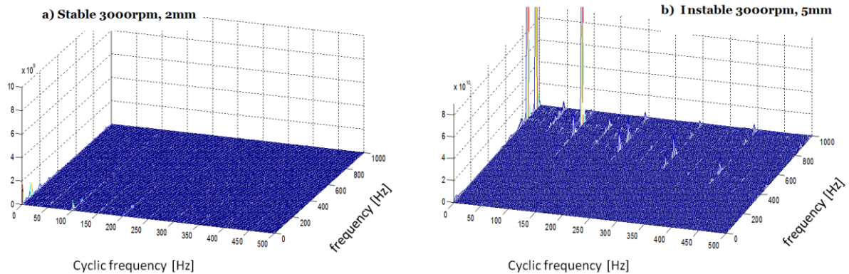
Figure 57 -Corrélation spectrale des signaux de force de coupe dans les cas stable (a) et instable (b).
