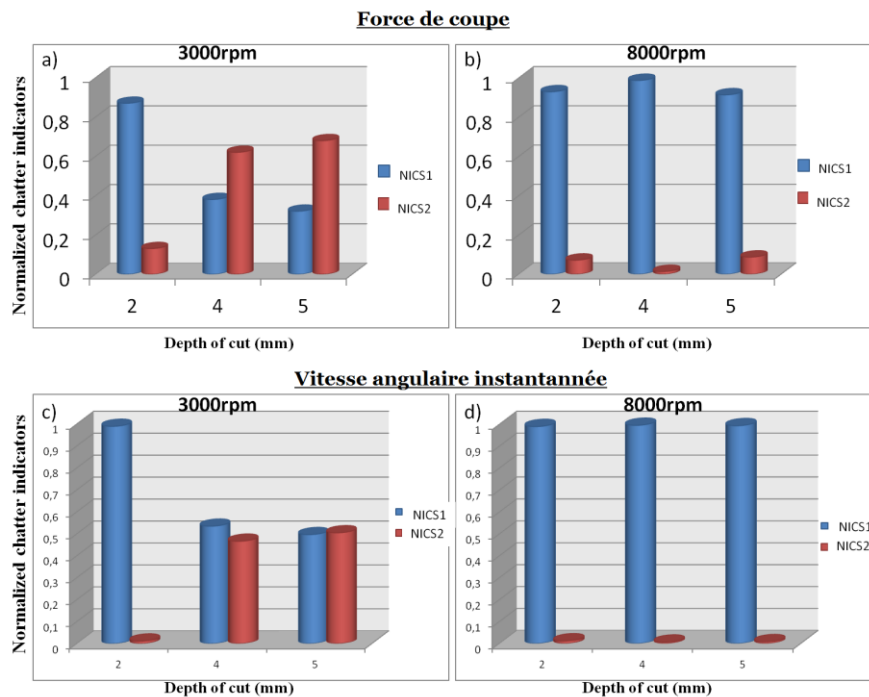
Figure 63 -Histogramme des indicateurs du broutage normalisés pour les signaux de force (a,b) et les signaux de vitesse (c,d) dans les conditions stables et instables (voir le tableau 4.1).
