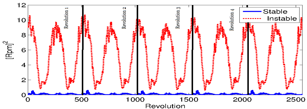
Figure 59 -Variance angulaire synchrone des signaux de force pour les cas stable (bleu continue) et instable (rouge pointillée).
