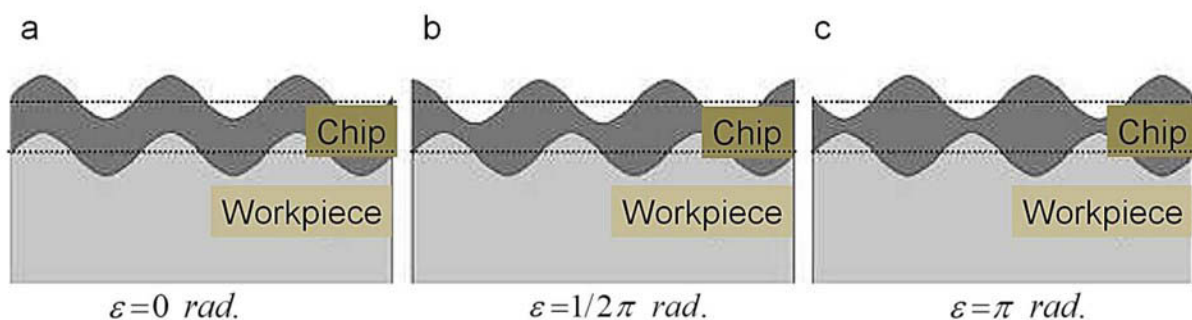
Figure 4 -L'effet de la différence de phase de deux passages consécutifs sur l'épaisseur du copeau [68].
