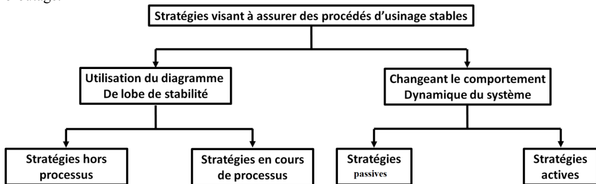
Figure 6 -Les stratégies visant à assurer des procédés d'usinage stables.
