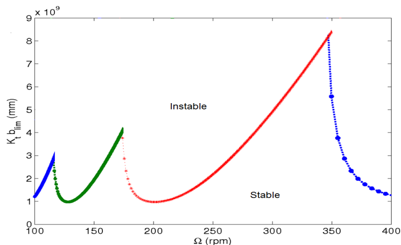
Figure 9 -Lobes de stabilité par la méthode analytique d'un système à 1 ddl. (Données prises des articles d'Altintas et Budak [76]).
