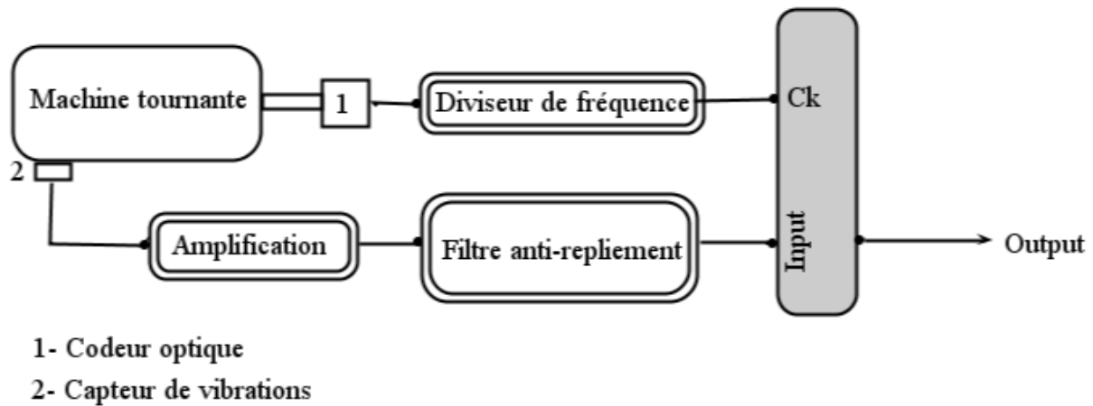
Figure 18 - Chaîne d'acquisition d'échantillonnage angulaire direct.
