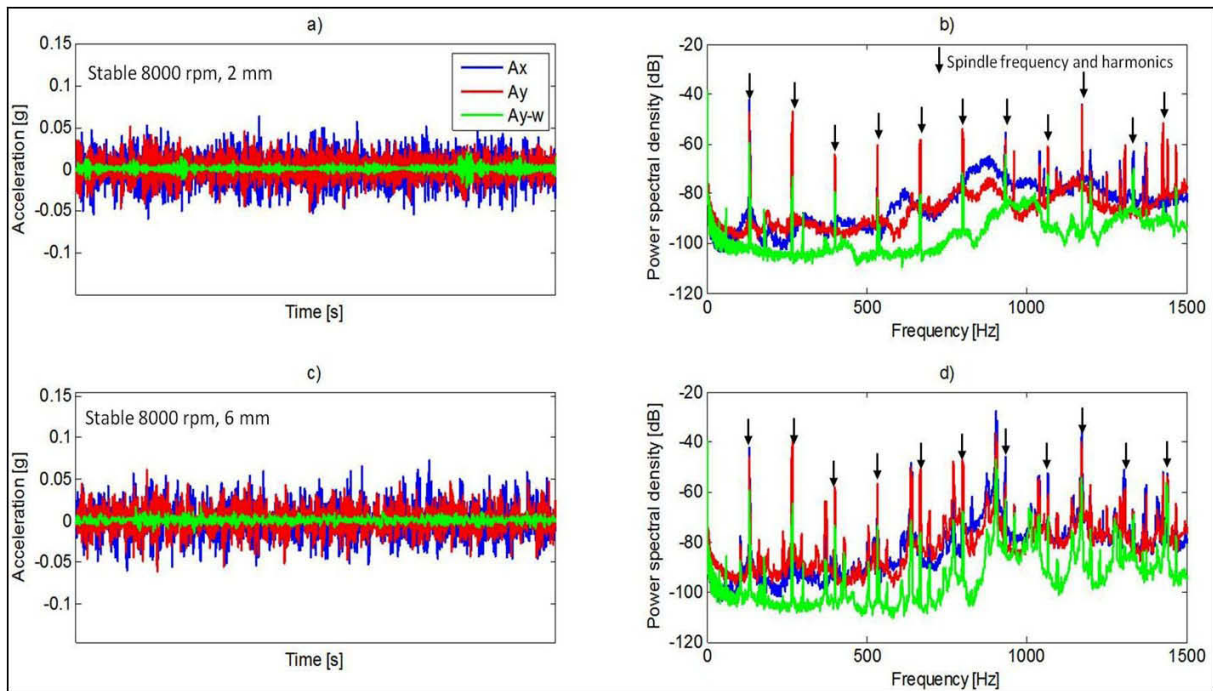
Figure 30 -Présentations temporelles et densité spectrale de puissance des signaux d'accélération. Ax : le signal issu du capteur placé dans la partie non rotative de la broche dans la direction X. Ay : le signal issu du capteur placé dans la partie non rotative de la broche dans la direction Y. Ayw : le signal issu du capteur placé sur la pièce dans la direction Y. (a) et (b) présentent les conditions stables (8000rpm, 2mm), (c) et (d) présentent les conditions instables (8000rpm, 6mm). Les paramètres de la PSD sont : la résolution fréquentielle est égale à 1.3 Hz, le nombre de moyennes utilisé est 60, la fenêtre utilisée est hamming et la méthode d'estimation utilisée est le périodogramme de Welch. Les flèches noires indiquent la fréquence de rotation de la broche et ses harmoniques. D'autres composants correspondent aux fréquences du broutage.
