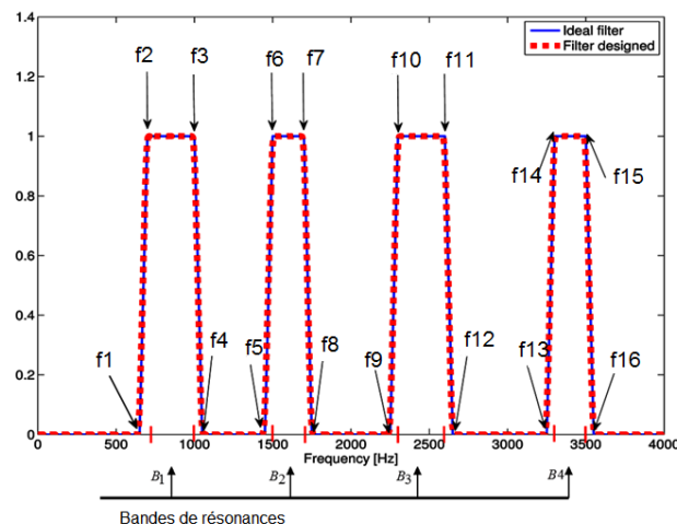
Figure 65 -Caractéristiques du filtre multi bande.
