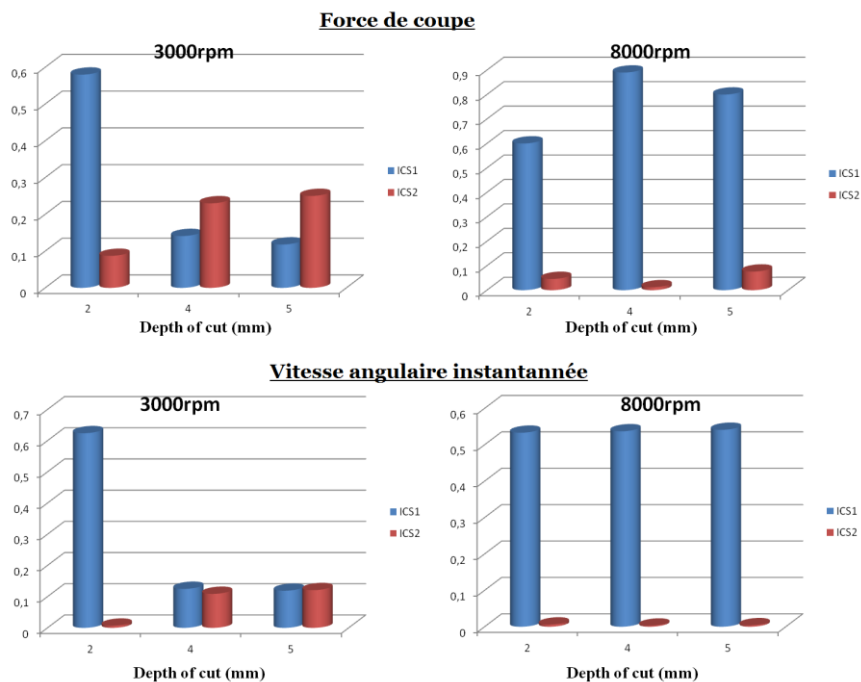
Figure 62 -Histogramme des indicateurs du broutage pour les signaux de force (a,b) et les signaux de vitesse (c,d) dans les conditions stables et instables (voir le tableau 4.1).
