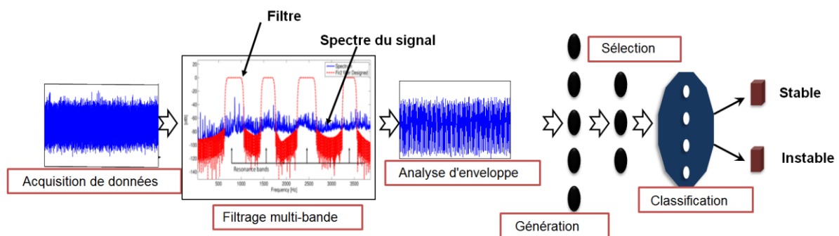
Figure 68 -Architecture de la méthodologie proposée.
