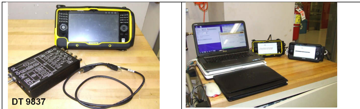
Système d'acquisition
