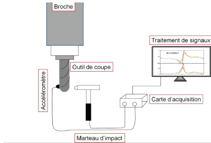
Figure 8 -Schéma de principe de test d'impact.
