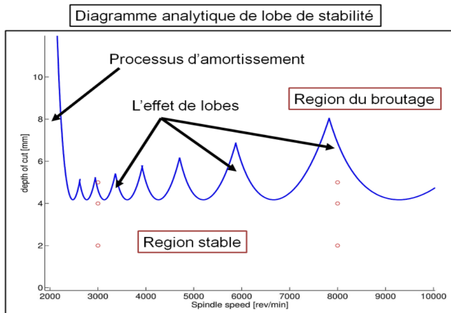
Figure 5 -Diagramme des lobes de stabilité.
