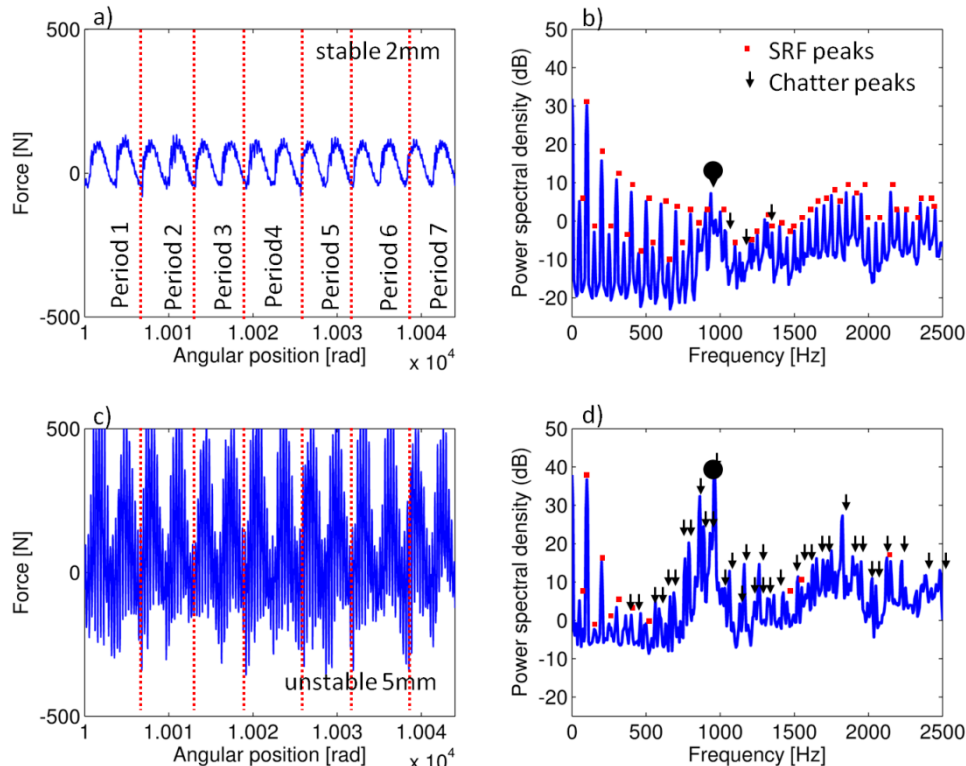
Figure 49 -Représentation angulaire et spectrale (PSD) des signaux de force dans la direction d'avance F_f . (a,b) Conditions stables (3000rpm, 2mm, N 2 dents). (c,d) Conditions instables (3000rpm, 5mm, N 2 dents). Les points rouges caractérisent la fréquence de rotation de la broche et ses harmoniques. Les flèches noires dénotent les fréquences excitées liées au broutage. Les disques noirs montrent les résonances.
