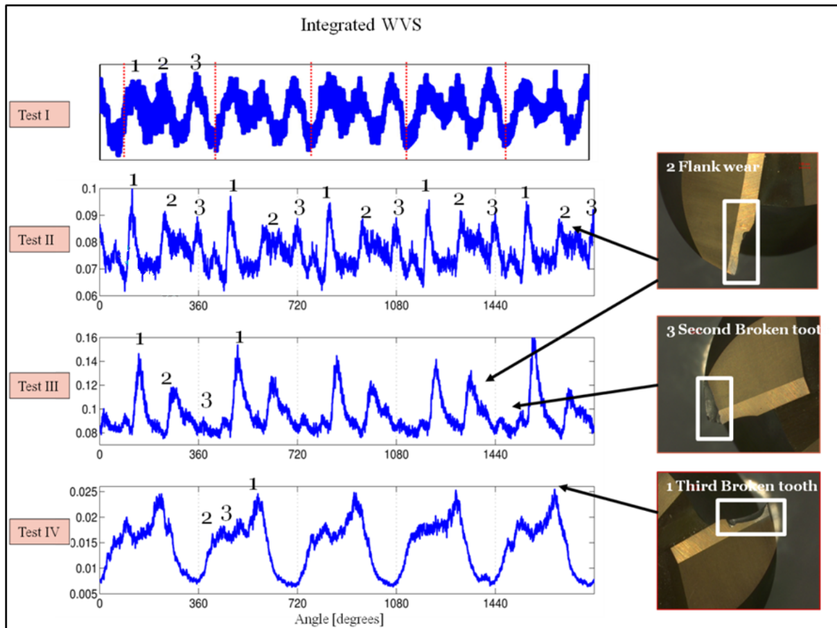
Figure 44 -Transformation de WignerVille intégrée estimée sur 5 rotations et 300 cycles pour les quatre scénarios.
