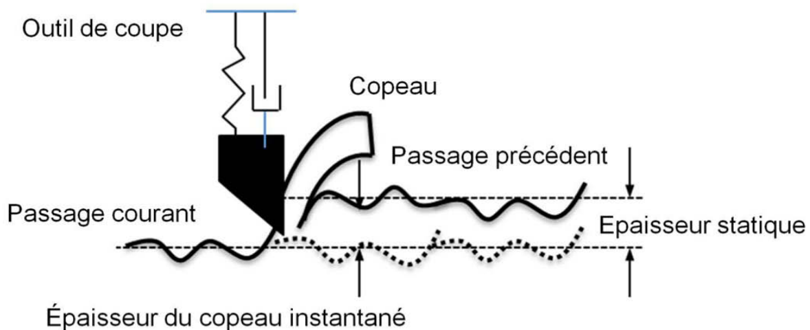
Figure 3 -Phénomène de régénération de la surface en opération de tournage.
