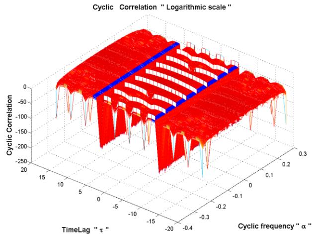
Figure 12 -Fonction d'autocorrélation cyclique en échelle logarithmique d'un train d'impulsions modulé en amplitude.
