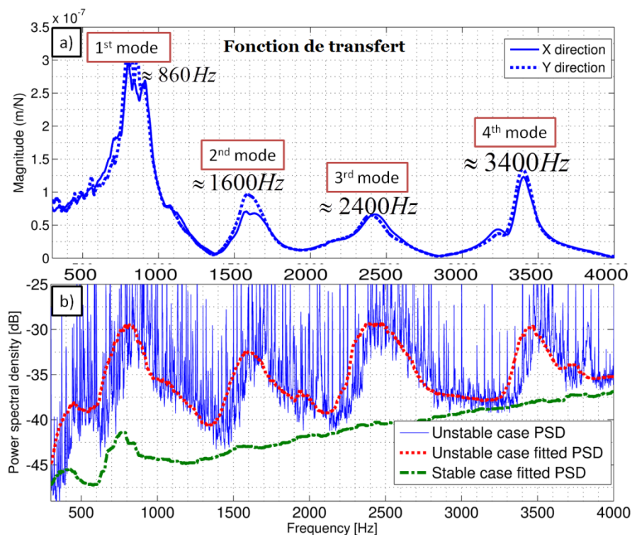
Figure 55 - Comparaison entre la densité spectrale de puissance de la vitesse instantanée et la fonction de réponse en fréquence du système outil/ porte outil/ broche. (a) La fonction de réponse en fréquence mesurée dans les directions X (courbe continue) et Y (courbe en pointillés). (b) La courbe bleue montre la densité spectrale de puissance dans les conditions instables. La courbe rouge montre la densité spectrale de puissance dans les conditions stables.
