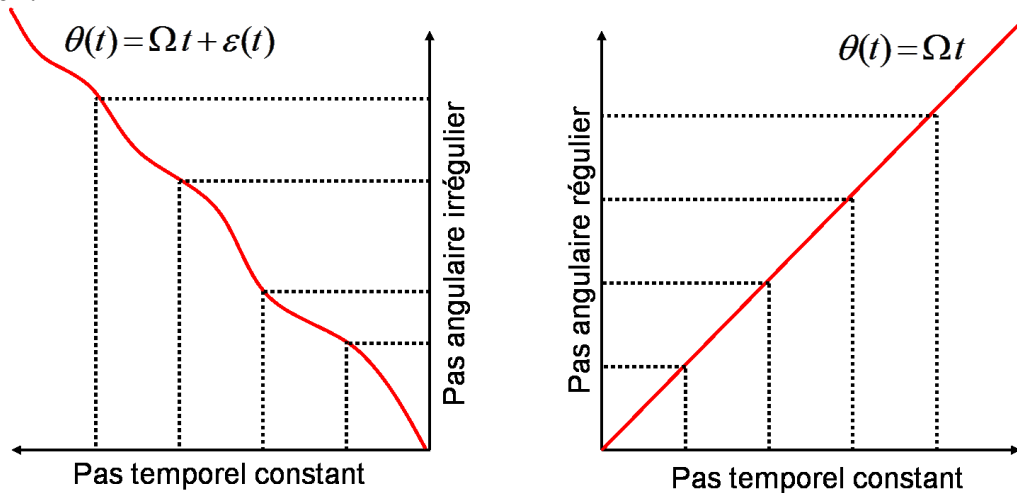
Figure 17 -Échantillonnage temporel vs angulaire.
