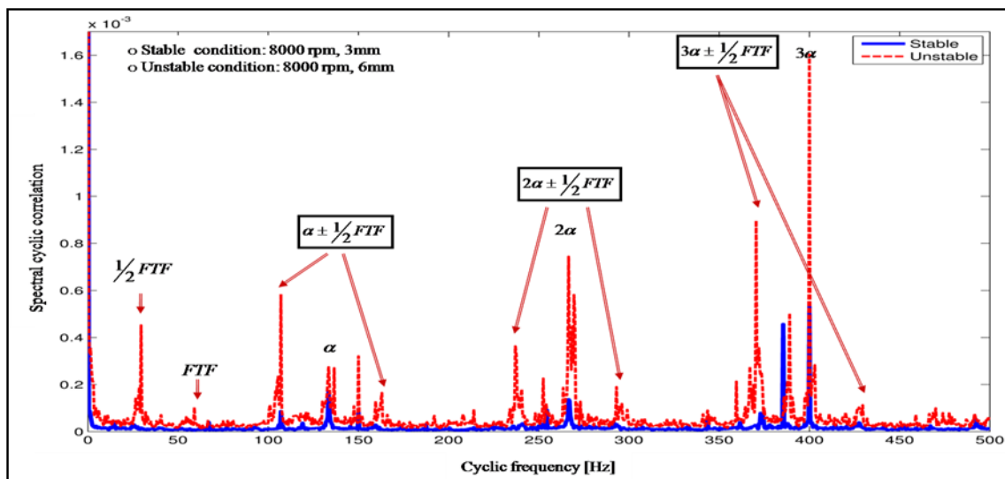
Figure 38 -Densité spectrale cyclique intégrée dans les conditions stables (courbe en bleu et rouge). FTF=59 Hz.
