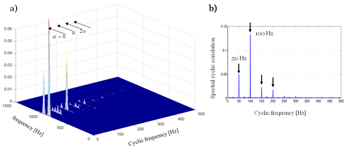
Figure 35 - (a) Corrélation spectrale cyclique. (b) Corrélation spectrale cyclique intégrée du signal acquis à l'état stable (3000rpm, 3mm). Les flèches montrent les fréquences cycliques.
