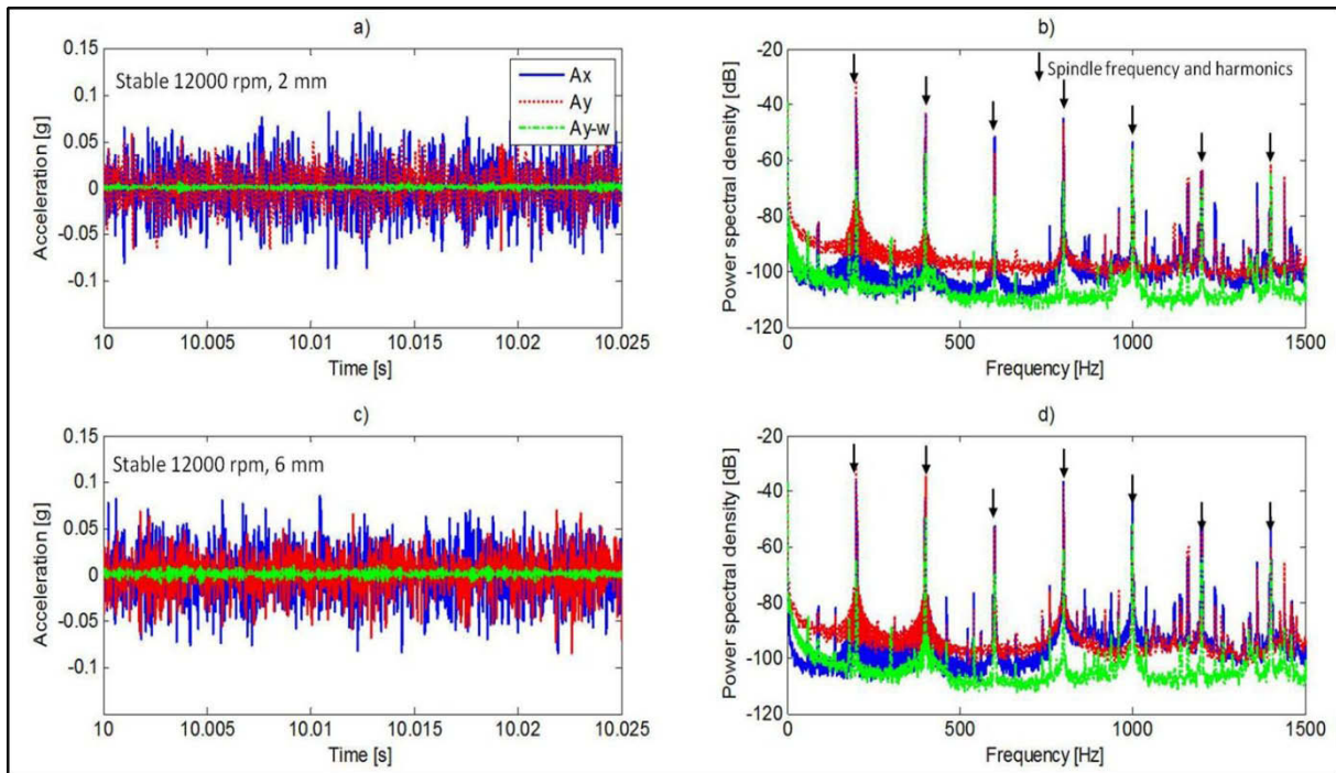
Figure 31 -Présentations temporelles et densité spectrale de puissance des signaux d'accélération. Ax : le signal issu du capteur placé dans la partie non rotative de la broche dans la direction X. Ay : le signal issu du capteur placé dans la partie non rotative de la broche dans la direction Y. Ayw : le signal issu du capteur placé sur la pièce dans la direction Y. (a), (b), (c) et (d) présentent des conditions stables (12000rpm, 2mm et 12000rpm, 6mm). Les paramètres de la PSD sont : la résolution fréquentielle est égale à 1.3 Hz, le nombre de moyennes est 60, la fenêtre utilisée est hamming et la méthode d'estimation utilisée est le périodogramme de Welch. Les flèches noires indiquent la fréquence de rotation de la broche et ses harmoniques. D'autres composants correspondent aux fréquences du broutage.
