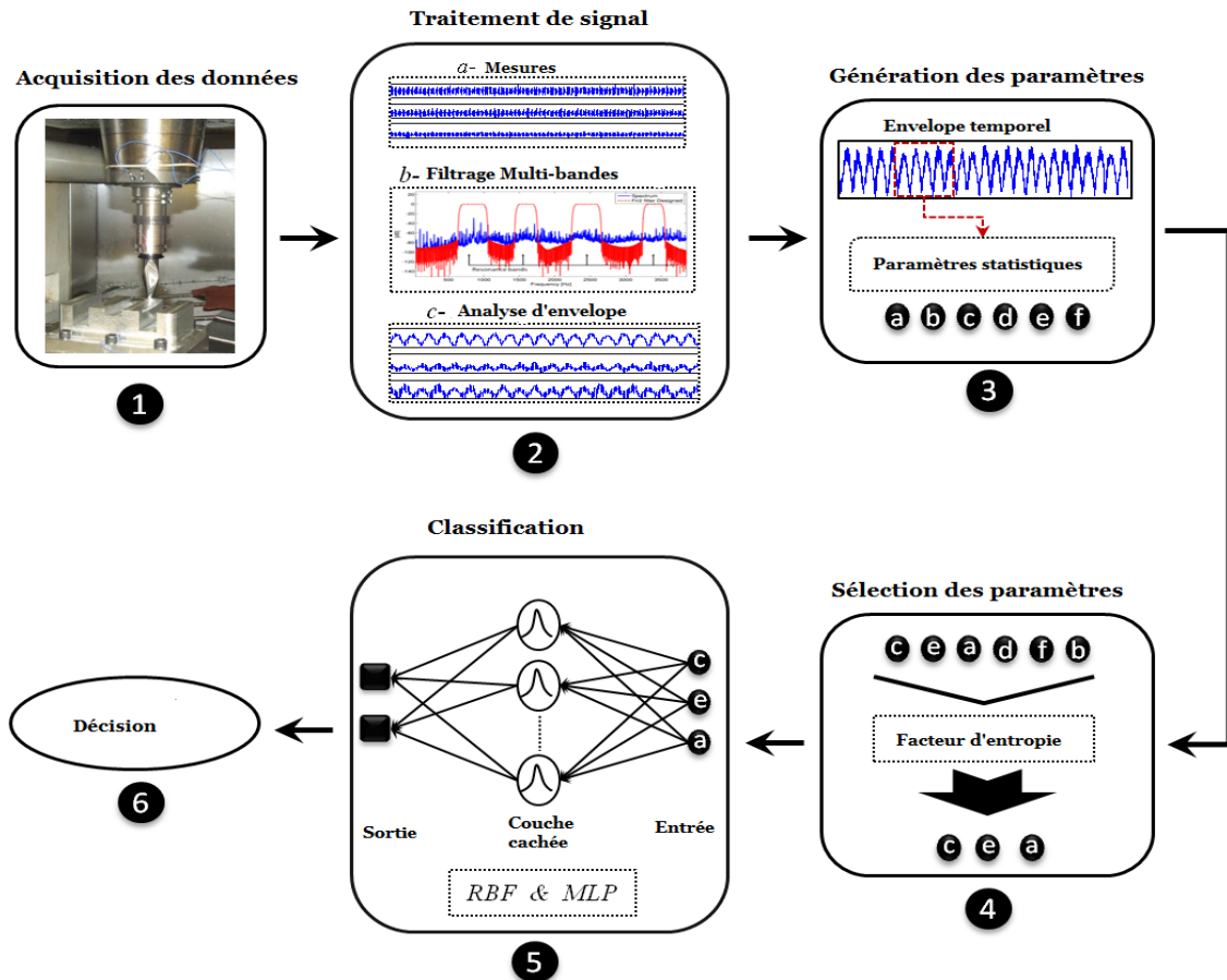
Figure 64 -Méthodologie pour la détection du broutage.
