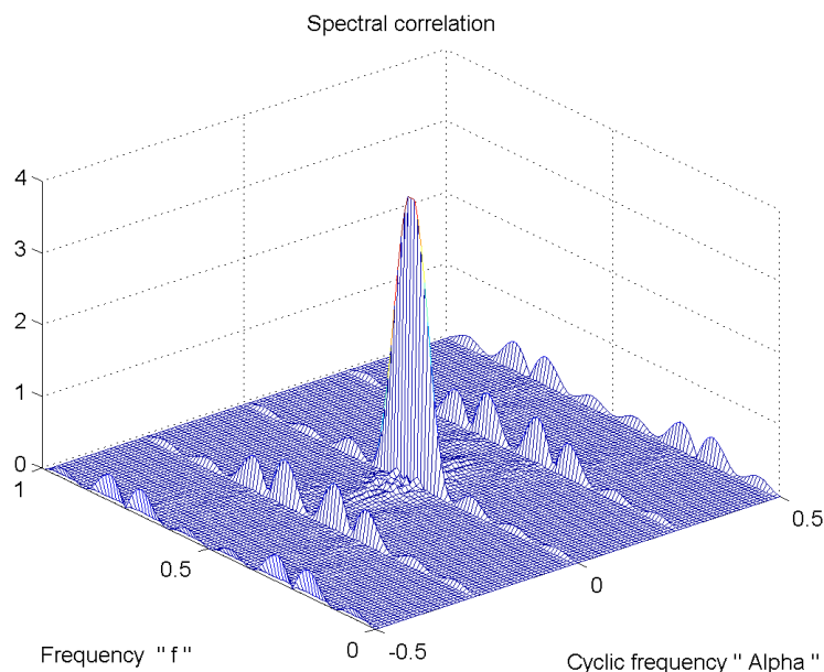
Figure 13 -Fonction de corrélation spectrale d'un train d'impulsions.
