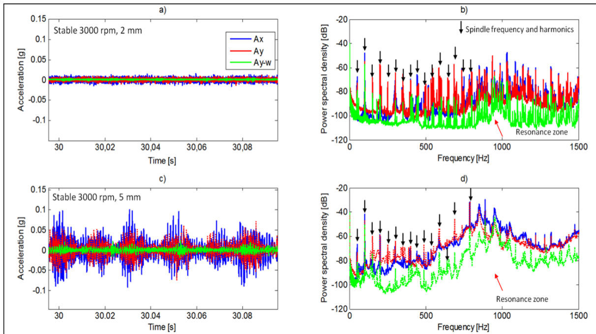
Figure 29 -Présentations temporelles et densité spectrale de puissance des signaux d'accélération. Ax : le signal issu du capteur placé dans la partie non rotative de la broche dans la direction X. Ay : le signal issu du capteur placé dans la partie non rotative de la broche dans la direction Y. Ayw : le signal issu du capteur placé sur la pièce dans la direction Y. (a) et (b) présentent les conditions stables (3000rpm, 2mm), (c) et (d) les conditions instables (3000rpm, 5mm). Les paramètres de la PSD sont : la résolution fréquentielle est égale à 1.3 Hz, le nombre de moyennes est 60, la fenêtre utilisée est hamming et la méthode d'estimation utilisée est le périodogramme de Welch. Les flèches noires indiquent la fréquence de rotation de la broche et ses harmoniques. D'autres composants correspondent aux fréquences du broutage.
