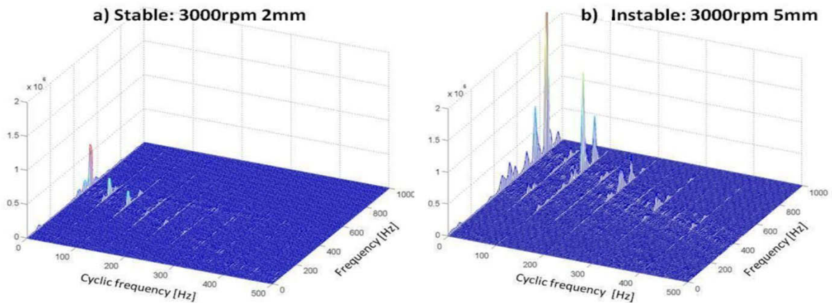
Figure 56 -Corrélation spectrale des signaux de vitesse dans les cas stable (a) et instable (b).
