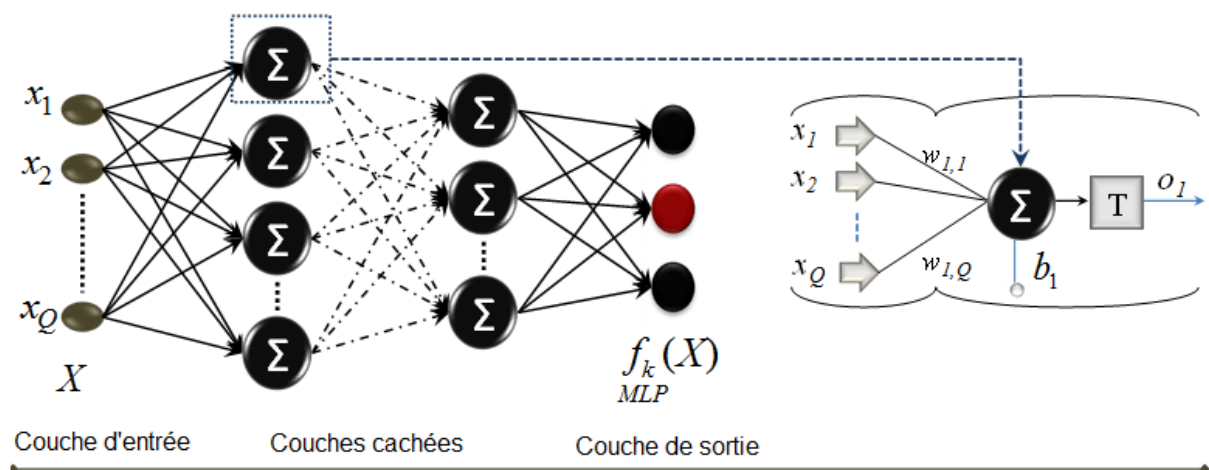
Figure 66 -Architecture du perceptron multicouche (MLP).
