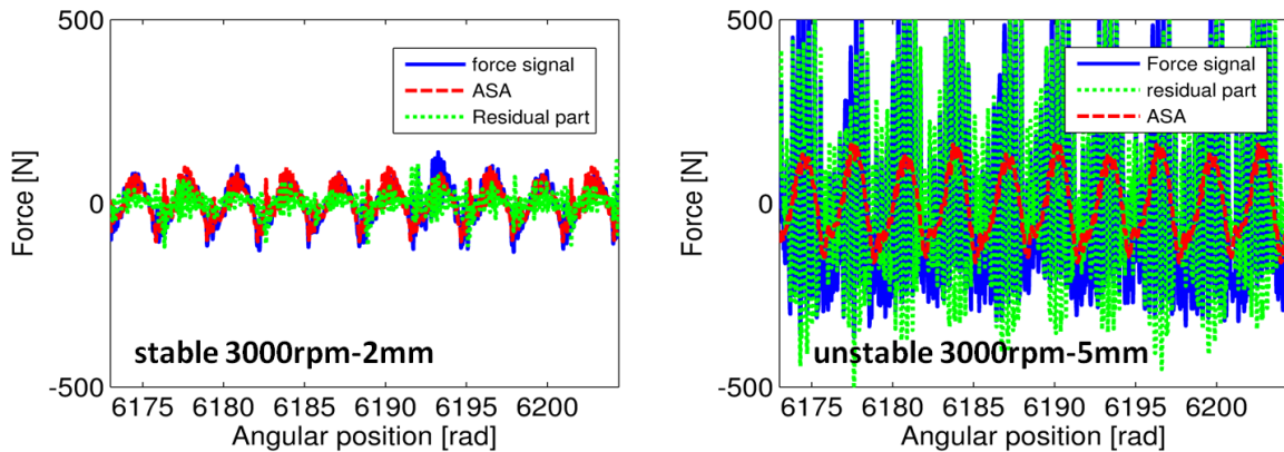
Figure 60 -Décomposition du signal de force de coupe.
