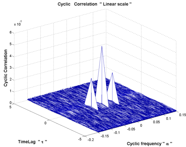
Figure 14 -Fonction d'autocorrélation cyclique en échelle linéaire d'un signal modulé en amplitude. Cette fonction n'est pas nulle pour les fréquences cycliques \alpha = 0 et \alpha = \pm 2f_0 .
