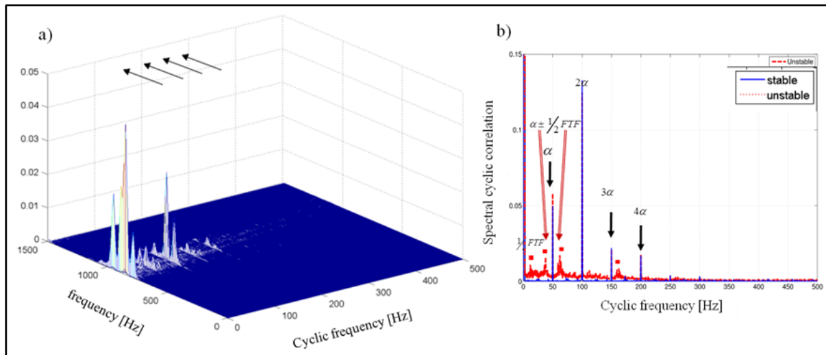
Figure 37 -(a) Corrélation spectrale cyclique aux conditions instables de fraisage (3000rpm, 5mm). (b) Densité spectrale cyclique intégrée pour les signaux acquis dans les conditions stables (courbe en bleu) et dans les conditions instables (courbe en rouge). Les flèches noires montrent les fréquences cycliques et les points rouges dénotent les fréquences de défaut de la cage (FTF 22 Hz) d'un roulement de la broche.
