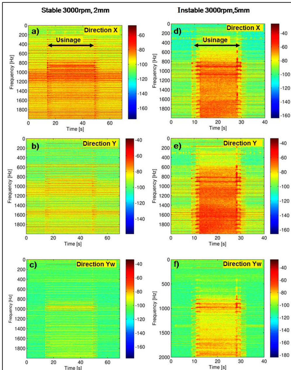
Figure 32 -Représentation temps fréquence des signaux d'accélération, dans les directions X ( A_x ) et Y ( A_y , A_{yw} ). (a,b,c) Les conditions de coupe stables sont : 3000rpm et 2mm de profondeur. (d,e,f) Les conditions de coupe instable sont : 3000rpm et 5mm de profondeur.
