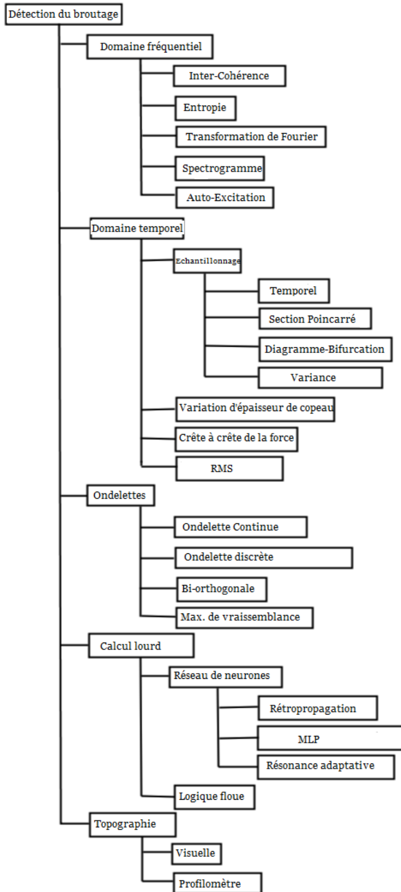
Figure 7 -Classification des techniques de détection du broutage [121].
