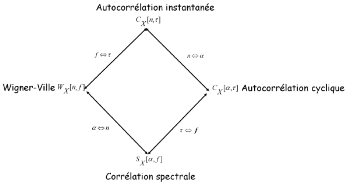
Figure 10 -Espace de représentation d'un processus cyclostationnaire à l'ordre (2).
