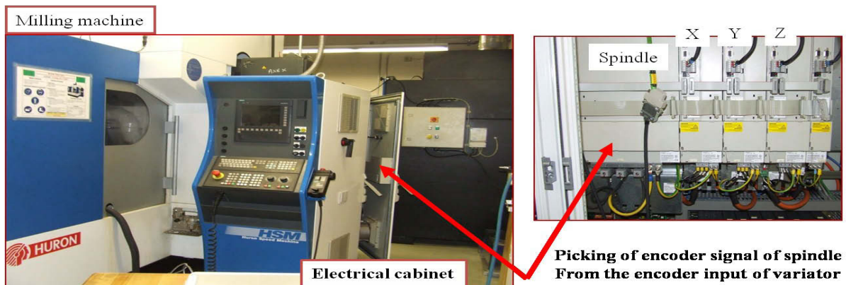
Figure 46 -Dérivation du signal du codeur angulaire de la broche
