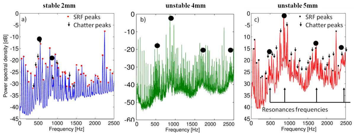
Figure 54 -Densité spectrale de puissance des signaux de vitesse dans différentes conditions. (a) 3000rpm et 2mm. (b) 3000rpm et 4mm. (c) 3000rpm et 5mm. Les points rouges dénotent la fréquence de rotation de la broche et ses harmoniques. Les flèches noires représentent les fréquences liées au broutage. Les disques noirs montrent les résonances.
