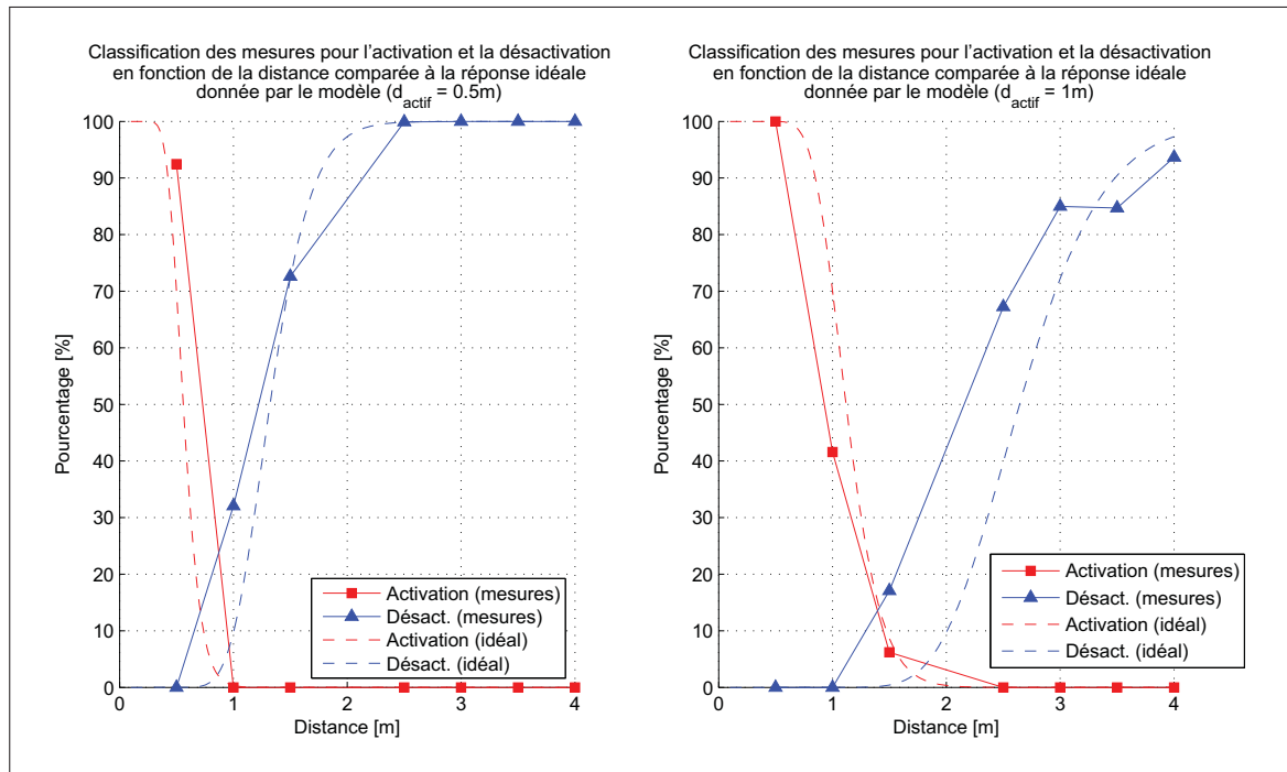
Figure 4.11 Résultats des décisions d'activation et de désactivation à partir des puissances mesurées en fonction de la distance pour une distance d'activation ( d_{\text{aktif}} ) de 0.5 mètre et de 1 mètre comparés aux courbes du modèle.
