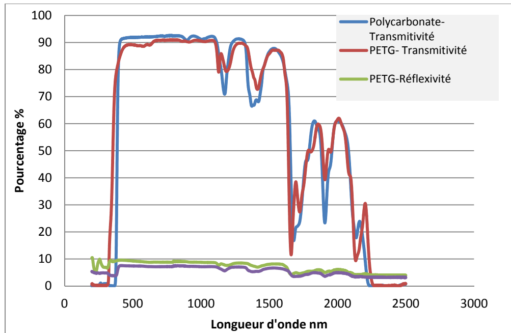
Figure-A II-1 : Transmittance et Réflectivité du polycarbonate et du PETG
