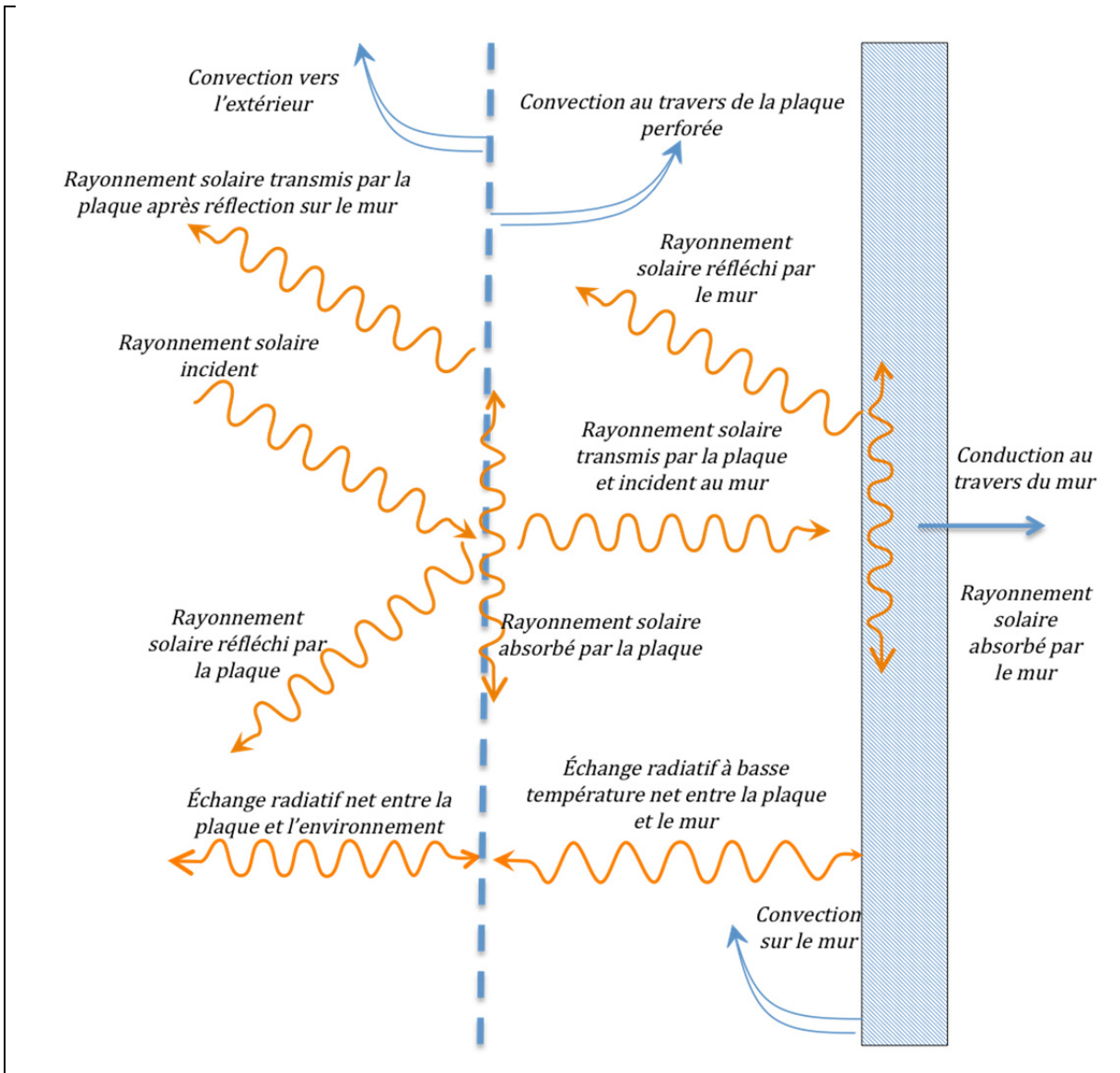
Figure 2.2 Ensemble des phénomènes physiques présents dans le TTC
