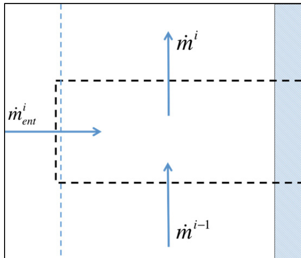
Figure 3.2 Bilan de masse de l'air dans un volume de contrôle
