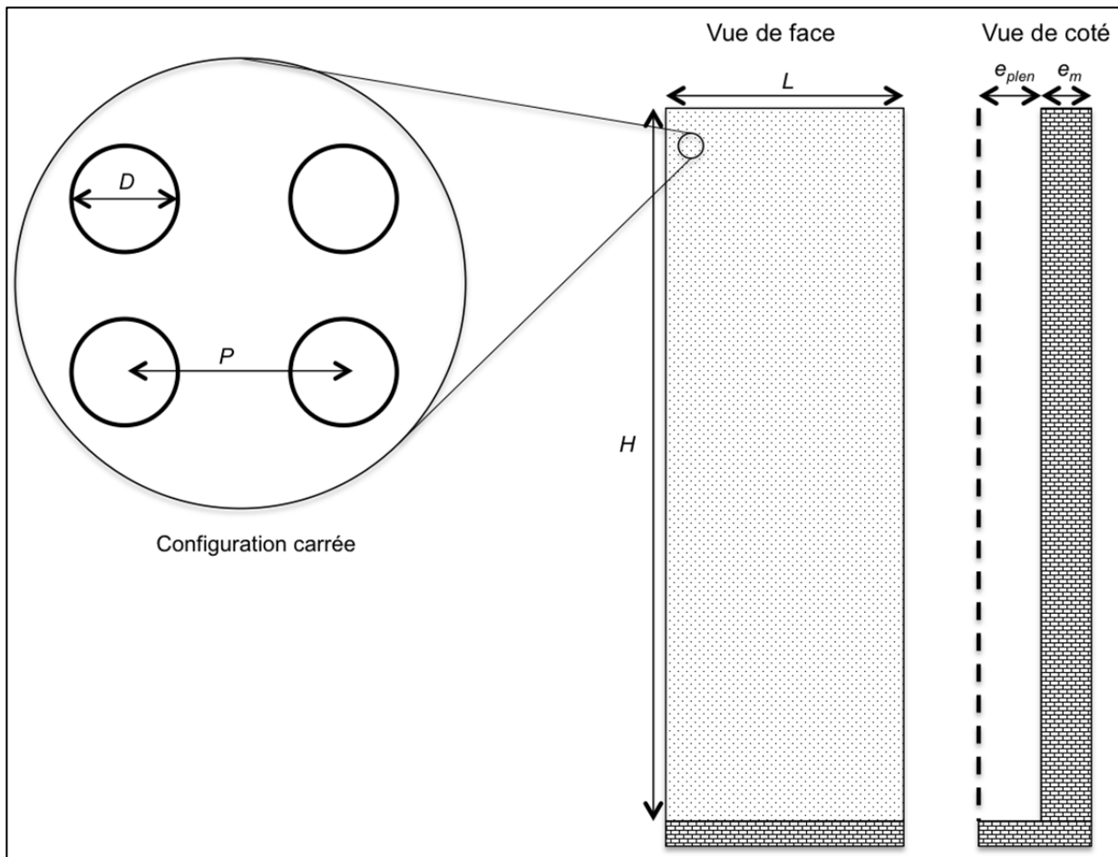
Figure 2.1 Géométrie d'un TTC
