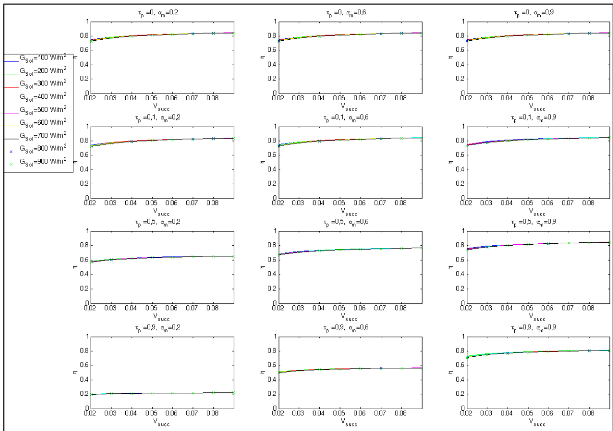
Figure-A III-1 : Rendement
