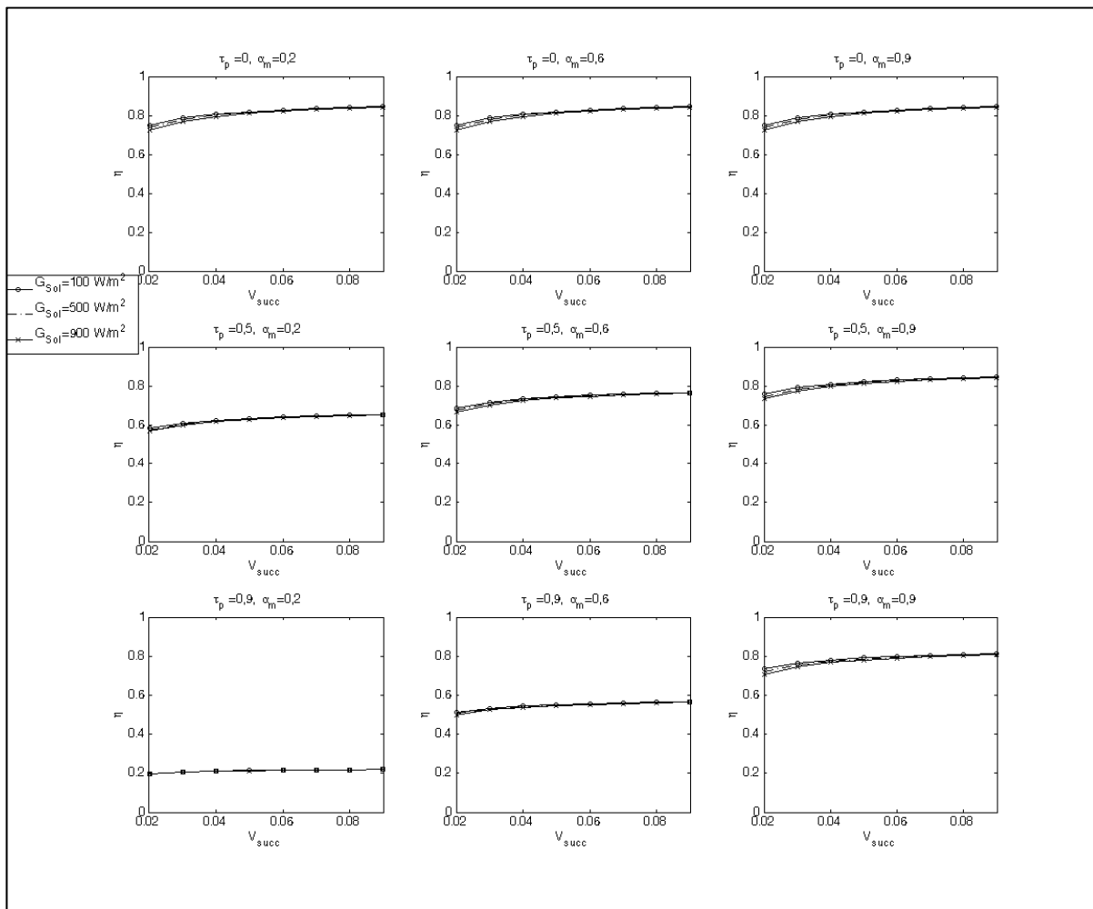
Figure 5.1 Rendement en fonction de V_{succ} , G_{Sol} , \tau_p et \alpha_m ( \epsilon_m=0,92 ; \epsilon_p=0,92 ; \epsilon_{amb}=1 ; \rho_p=0,08 )
