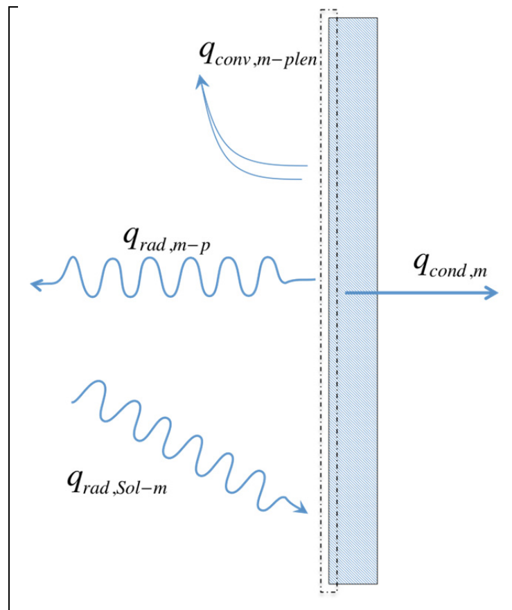
Figure 2.5 Bilan sur le mur
