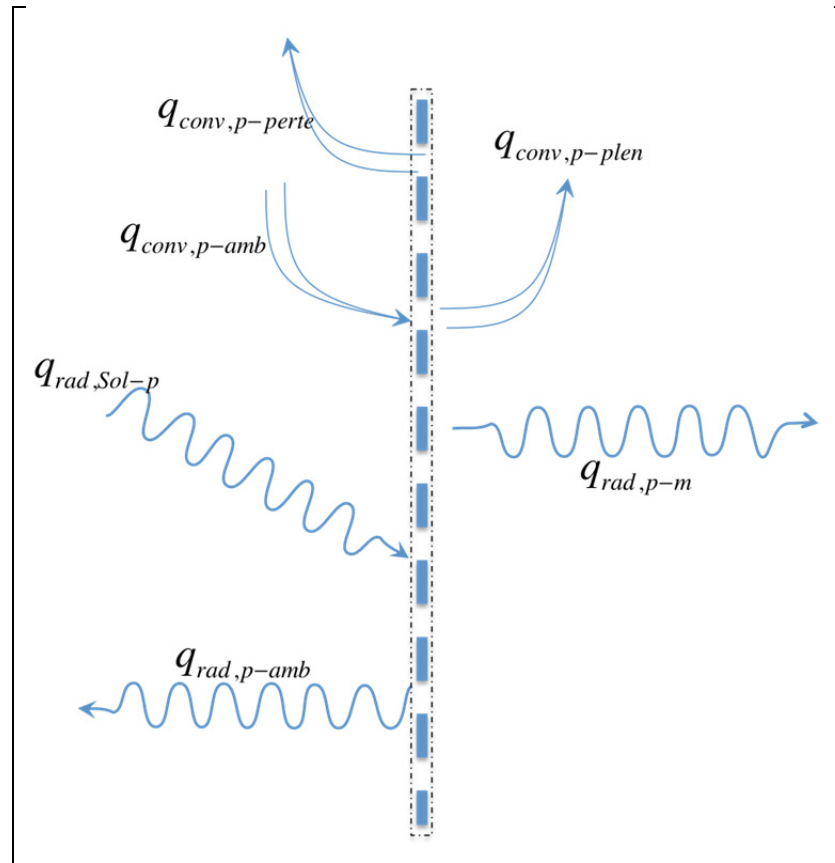
Figure 2.4 Bilan sur la plaque perforée semi-transparente
