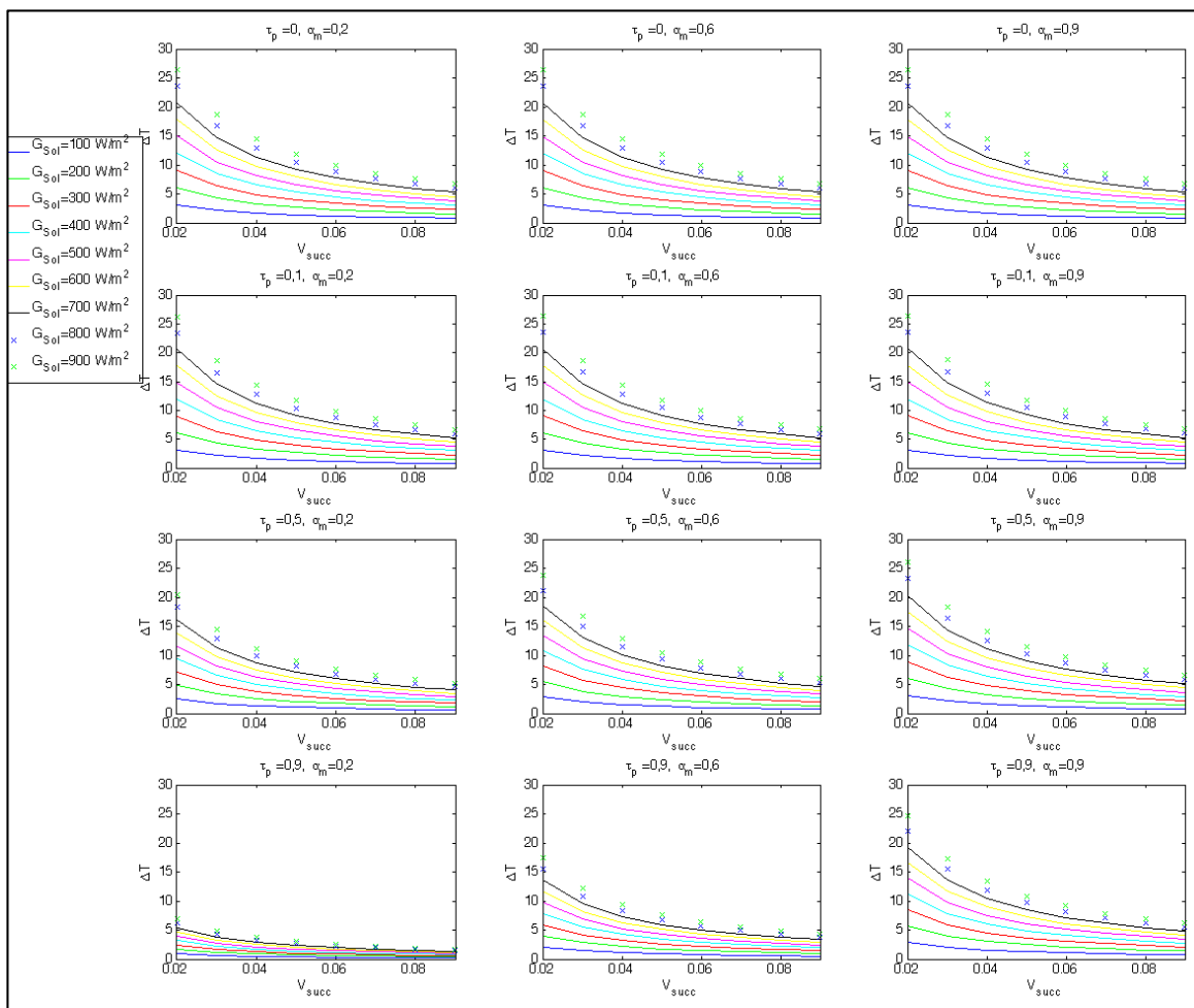
Figure-A IV-3 : Différence de température avec conduction
