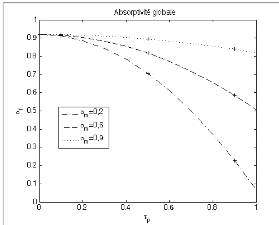
Figure 5.4 Évolution de l'absorptivité globale en fonction de \alpha_m et \tau_p
