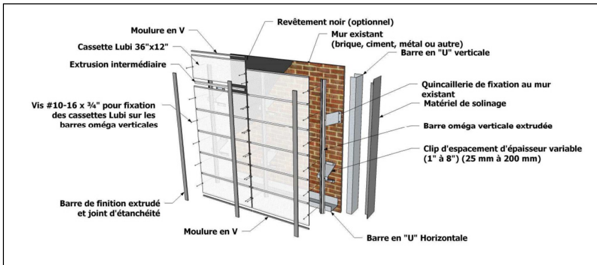
Figure 4.1 Montage du Lubi md tiré de (Enerconcept, 2012-03)
