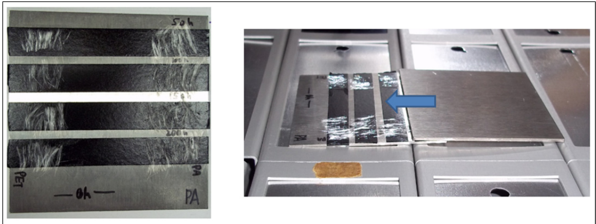
Figure 2.10: Méthode de préparation des échantillons pour le vieillissement accéléré
