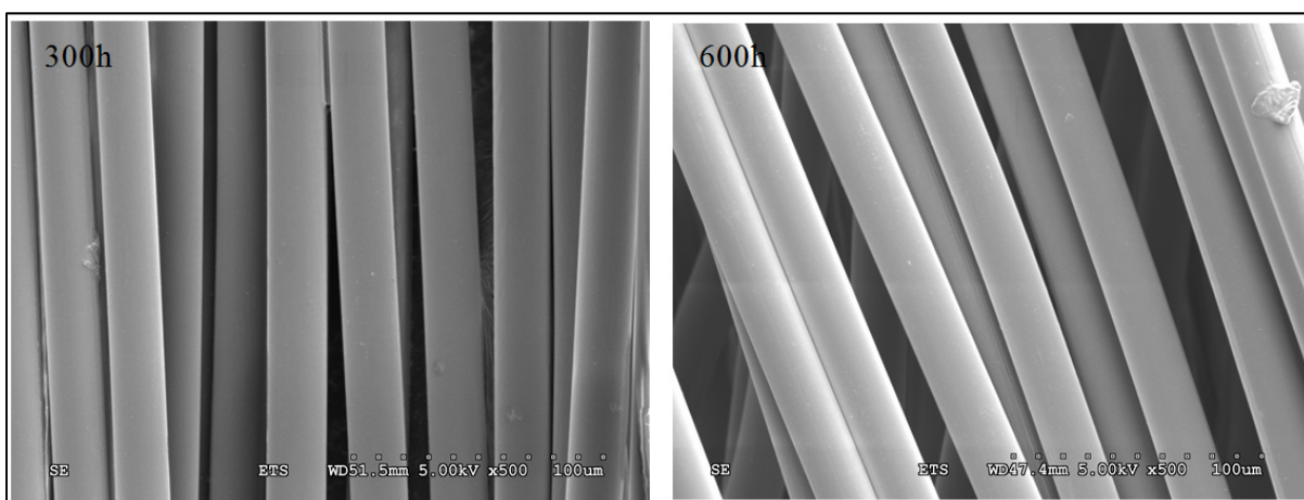
Figure 6.10: Fibres de PET au vieillissement photo-oxydatif à 0,68w/m^2 -50°C
