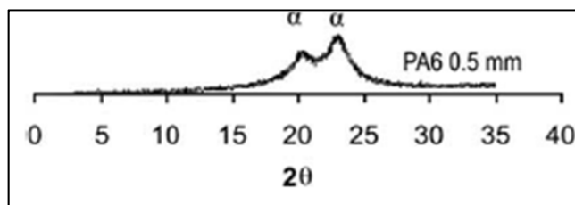
Figure 2.8: Exemple de DRX du PA-6 Tiré de Yebra-Rodriguez et al (2009)
