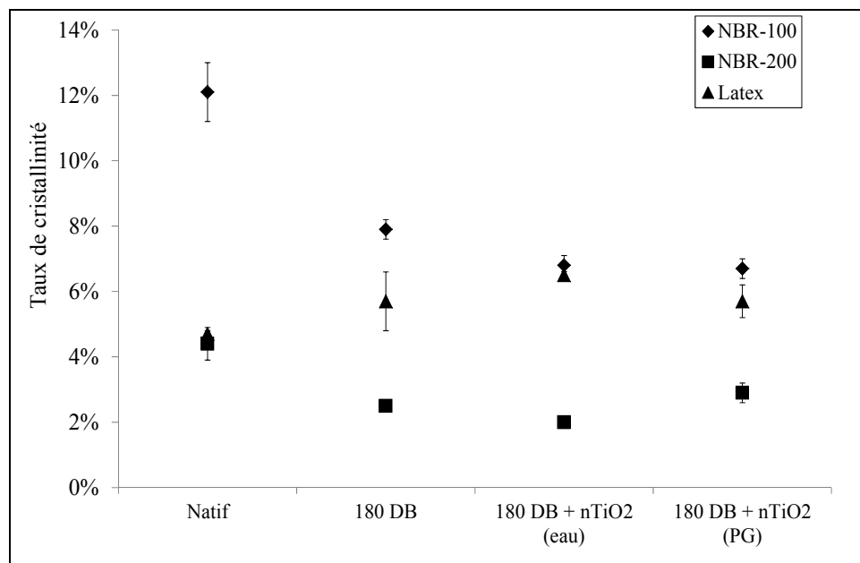
Figure 6-10. Variation du taux de cristallinité des échantillons en nitrile et en latex en fonction des conditions expérimentales
