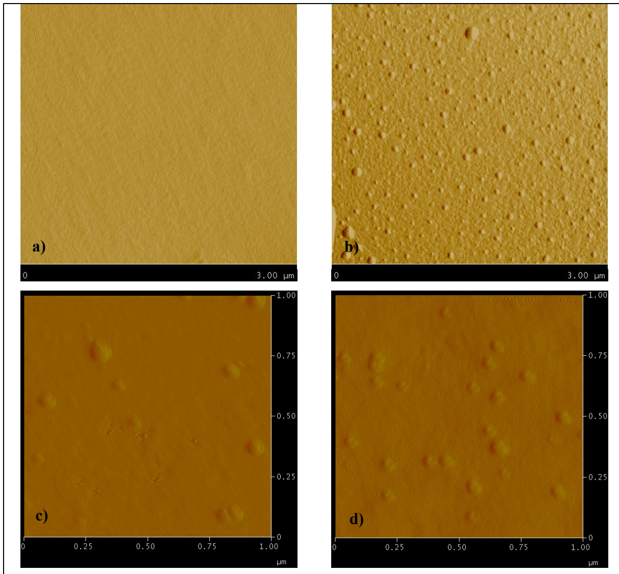
Figure 5-12. Images AFM a) d'un substrat de mica natif et b) c) et d) d'une solution d'échantillonnage centrifugée sur un substrat de mica correspondant un échantillon de NBR-100 soumis 120 DB en présence de nTiO 2 en poudre
