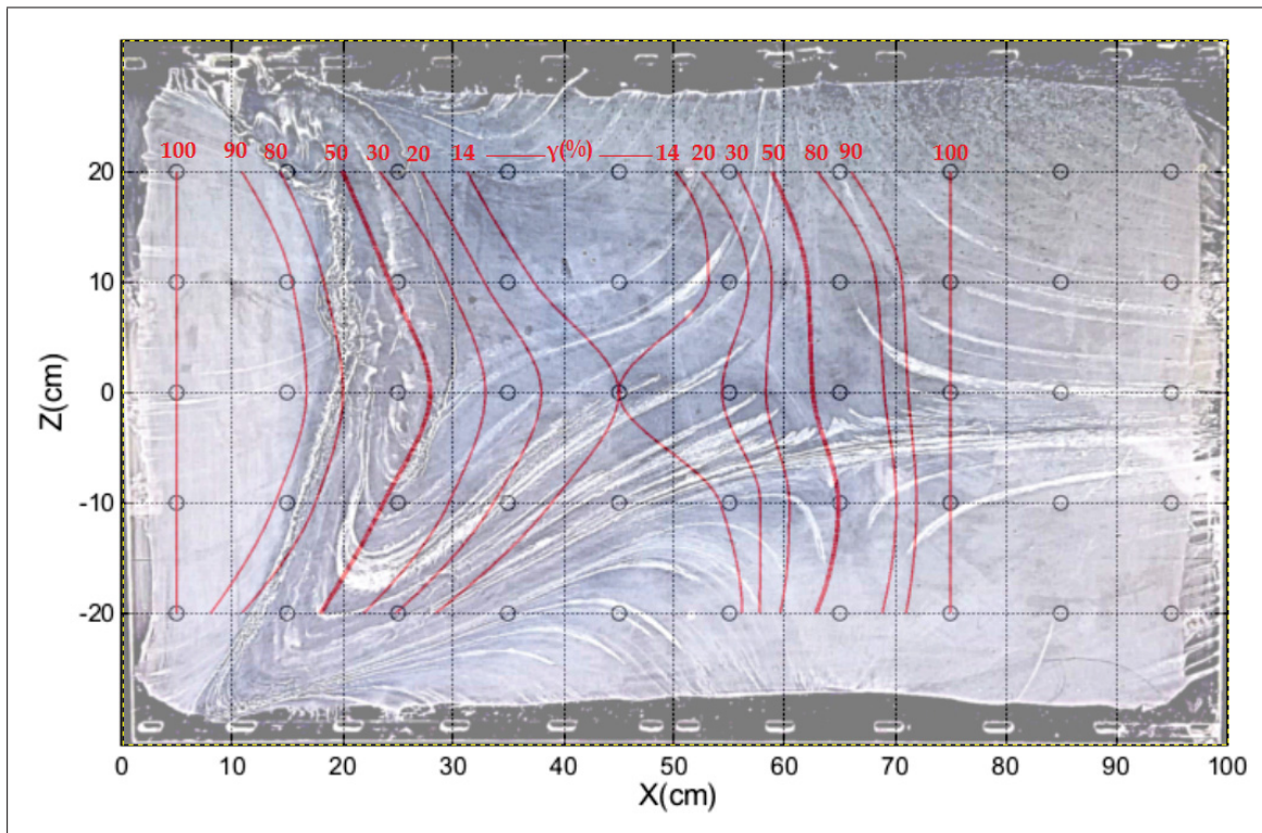
Figure 5.7 Superposition des courbes iso - \gamma au film d'huile obtenu pour U_0 = 25m/s
