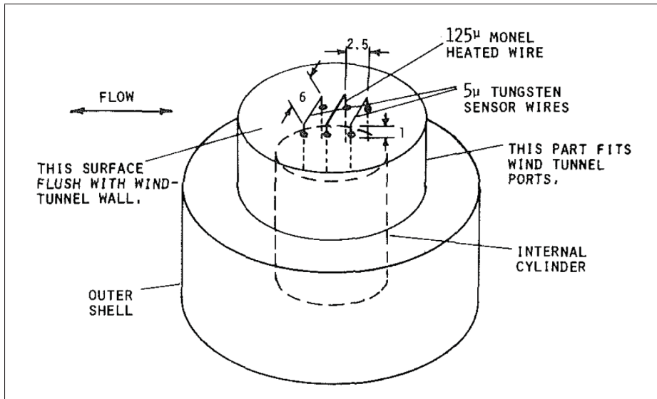
Figure 1.11 «Thermal Tuft» Tirée de Eaton et al. (1979)
