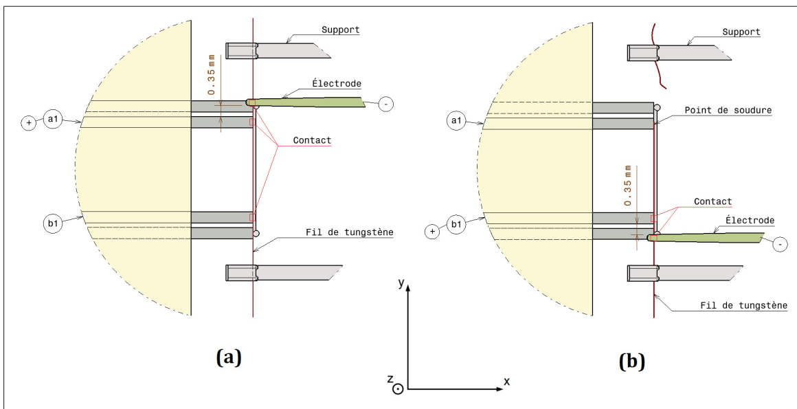
Figure-A II-7 Schéma des configurations (a) et (b) associées au Grafcet Figure-A II-5
