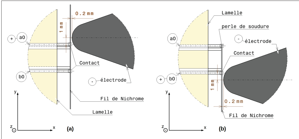
Figure-A II-6 Schéma des configurations (a) et (b) associées au Grafcet des Figures-A II-3 et II-4.
