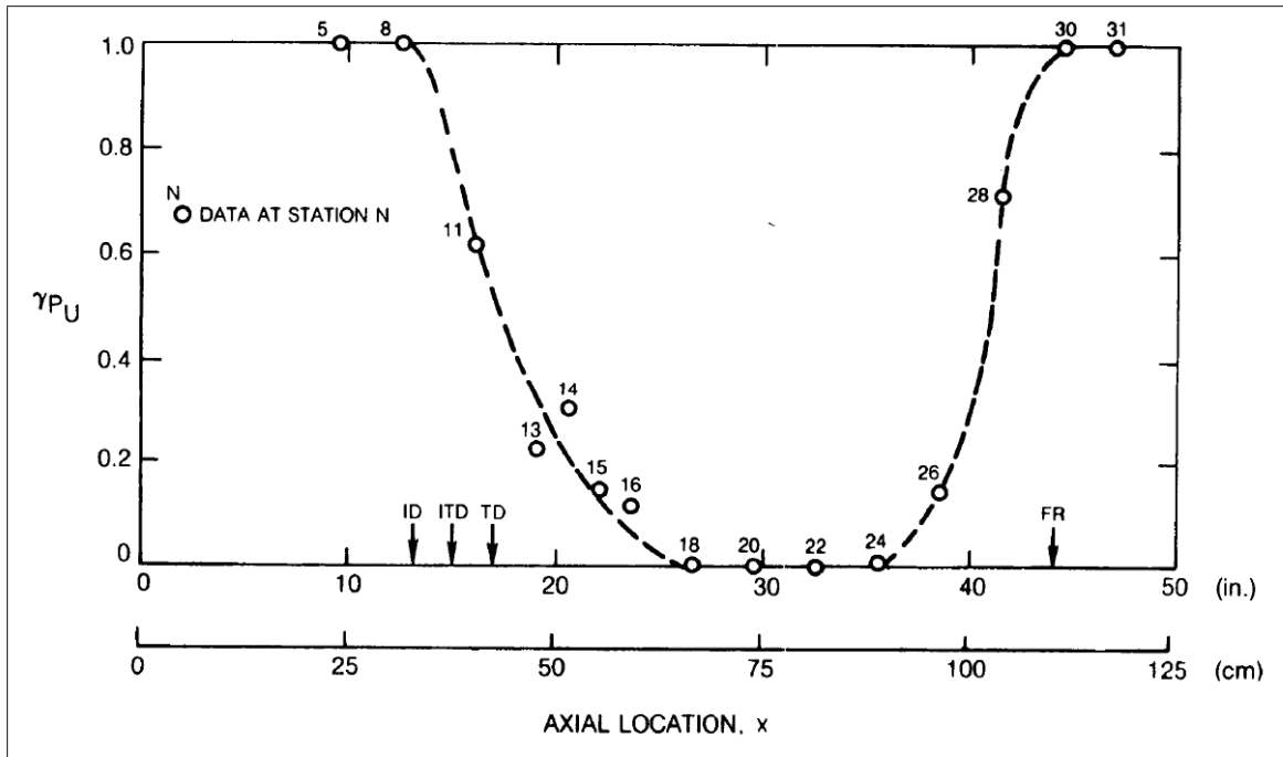
Figure 1.4 Distribution de \gamma dans le plan médian, à y = 1\text{mm} de la paroi Tirée de Patrick (1987)
