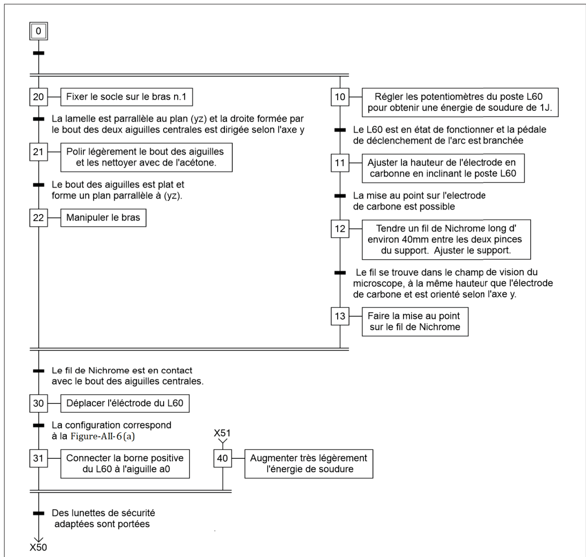
Figure-A II-3 Graficet du procédé de soudure à l'arc du fil de Nichrome : Partie 1
