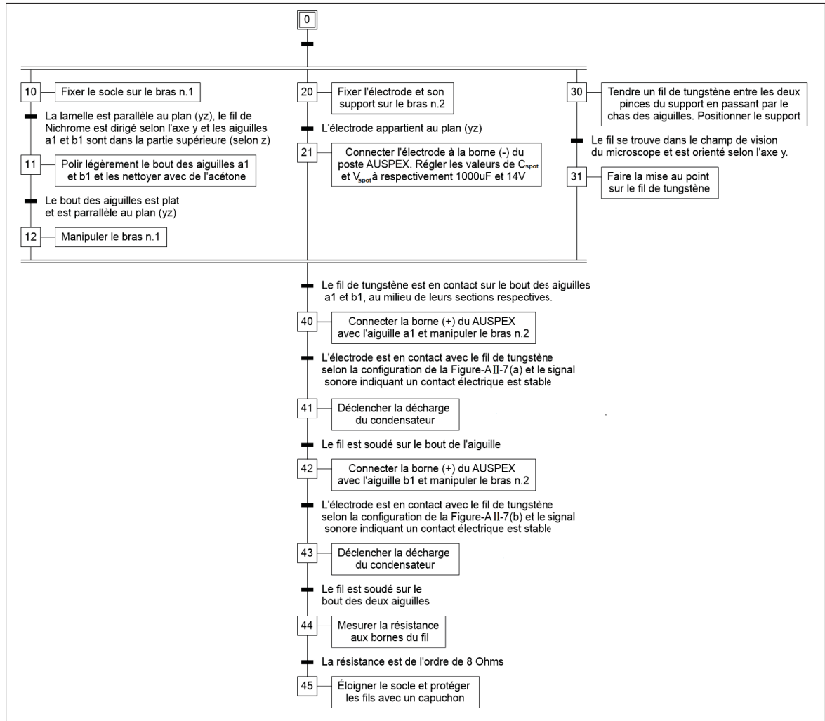
Figure-A II-5 Graficet du procédé de soudure par résistance d'un des deux fils latéraux
