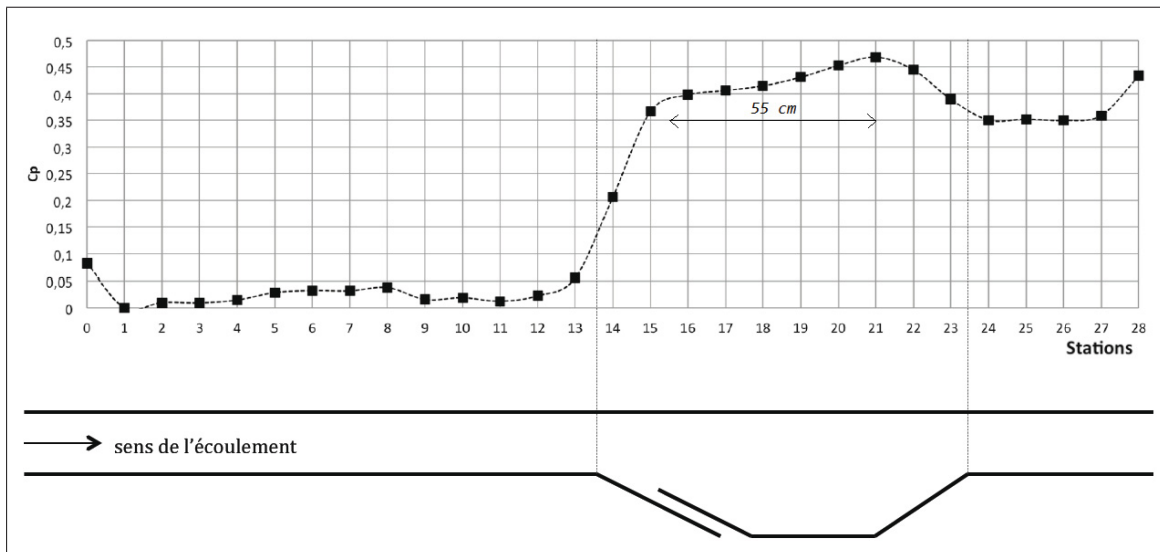
Figure 1.8 Évolution du coefficient de gradient de pression statique ( C_p ) le long du canal d'essai de la soufflerie du TFT pour une vitesse de référence de U_0 = 30\text{m/s} Tirée de Pionon (2012)
