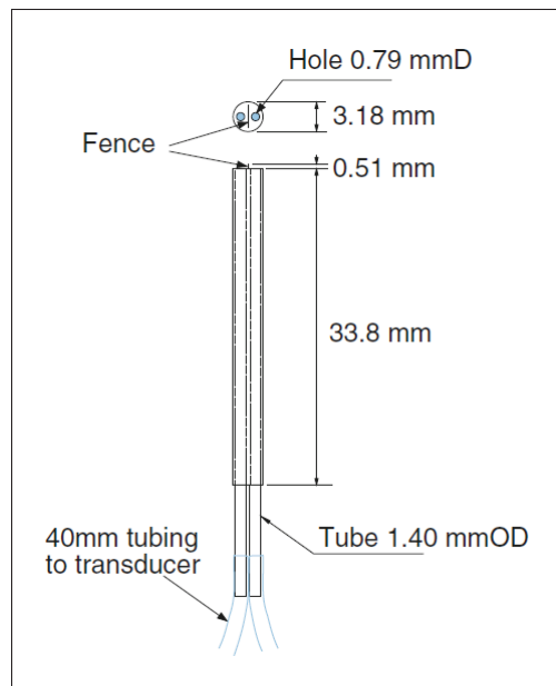
Figure 1.10 Principe du capteur «Fence Probe» Tirée de Sandborn et Seong (2012)
