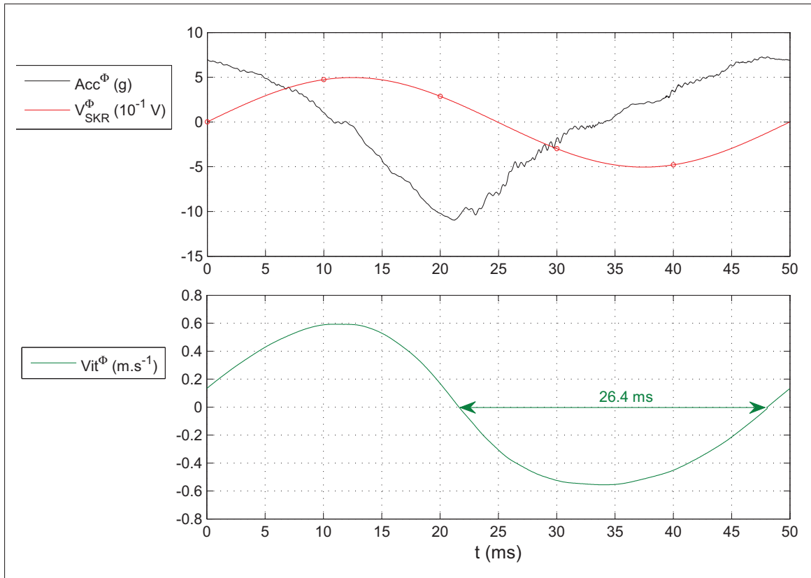
Figure 4.11 Calcul de la vitesse du pot vibrant
