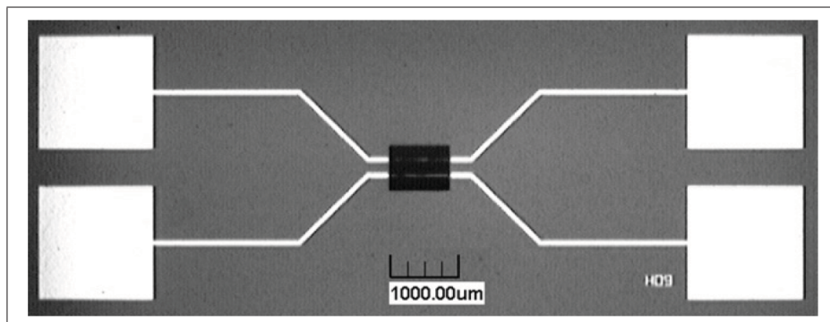
Figure 1.16 Vue de dessus du micro-capteur à deux fils Tirée de Buder et al. (2008)
