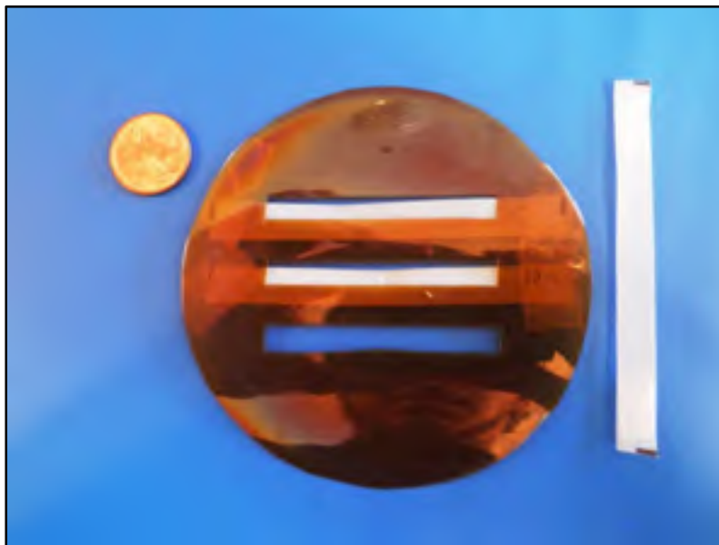
Figure 2.15 Masque de Kapton® et échantillons de PTFE pour essai de traction
