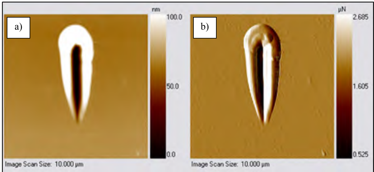
Figure 3.27 Relevé topographique (a) et gradient (b) de la surface de l'essai de nano-striage sur échantillon mince à sec par SPM
